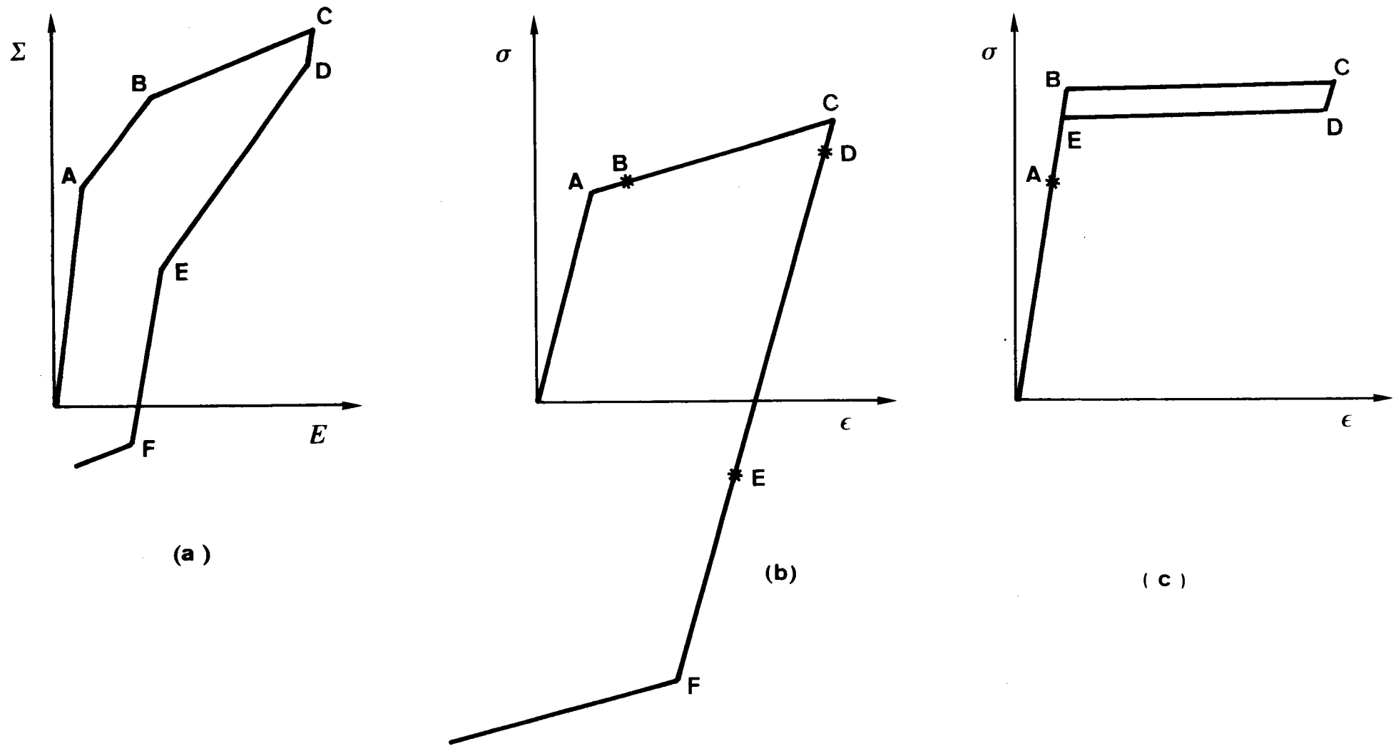
FIGURE VI.3 : Schéma décrivant l'évolution des contraintes dans le biphasé et dans les deux phases. 3.a : Courbe de traction du biphasé. 3.b : Evolution des contraintes dans la phase \alpha (supposée sans effet Bauschinger). 3.c : Evolution des contraintes dans la phase \beta .
