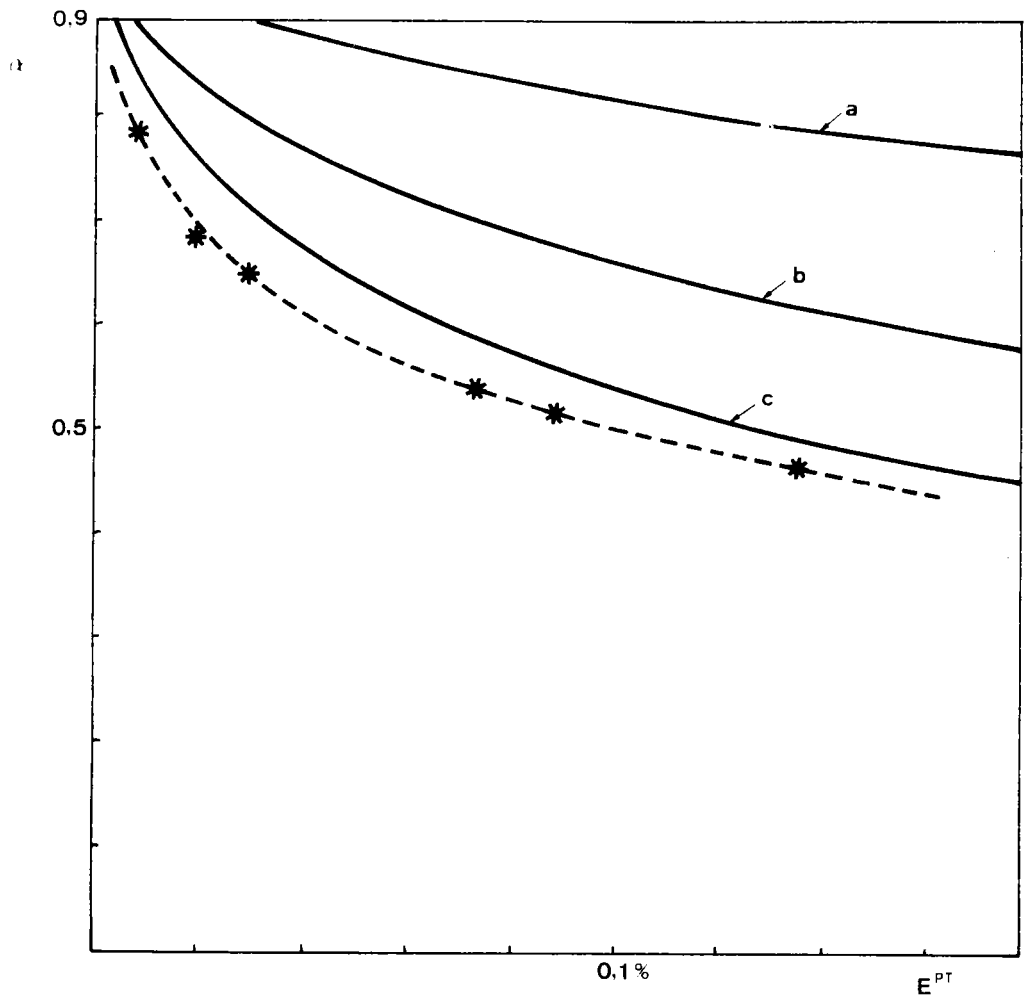
FIGURE V.15 : Evolution du paramètre d'accommodation plastique \alpha lors de la transformation martensitique d'un polycristal de Cu-Zn-Al.
