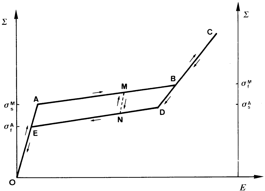
FIGURE III.5 : Modélisation de la courbe contrainte-déformation d'un monocristal pseudoélastique en traction uniaxiale isotherme.
