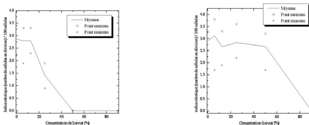
Figure 30 : Allure de la courbe concentration-réponse obtenue avec l'indice mitotique chez Vicia (à gauche) et Allium (à droite). Cas du lixiviat du sol SI.
