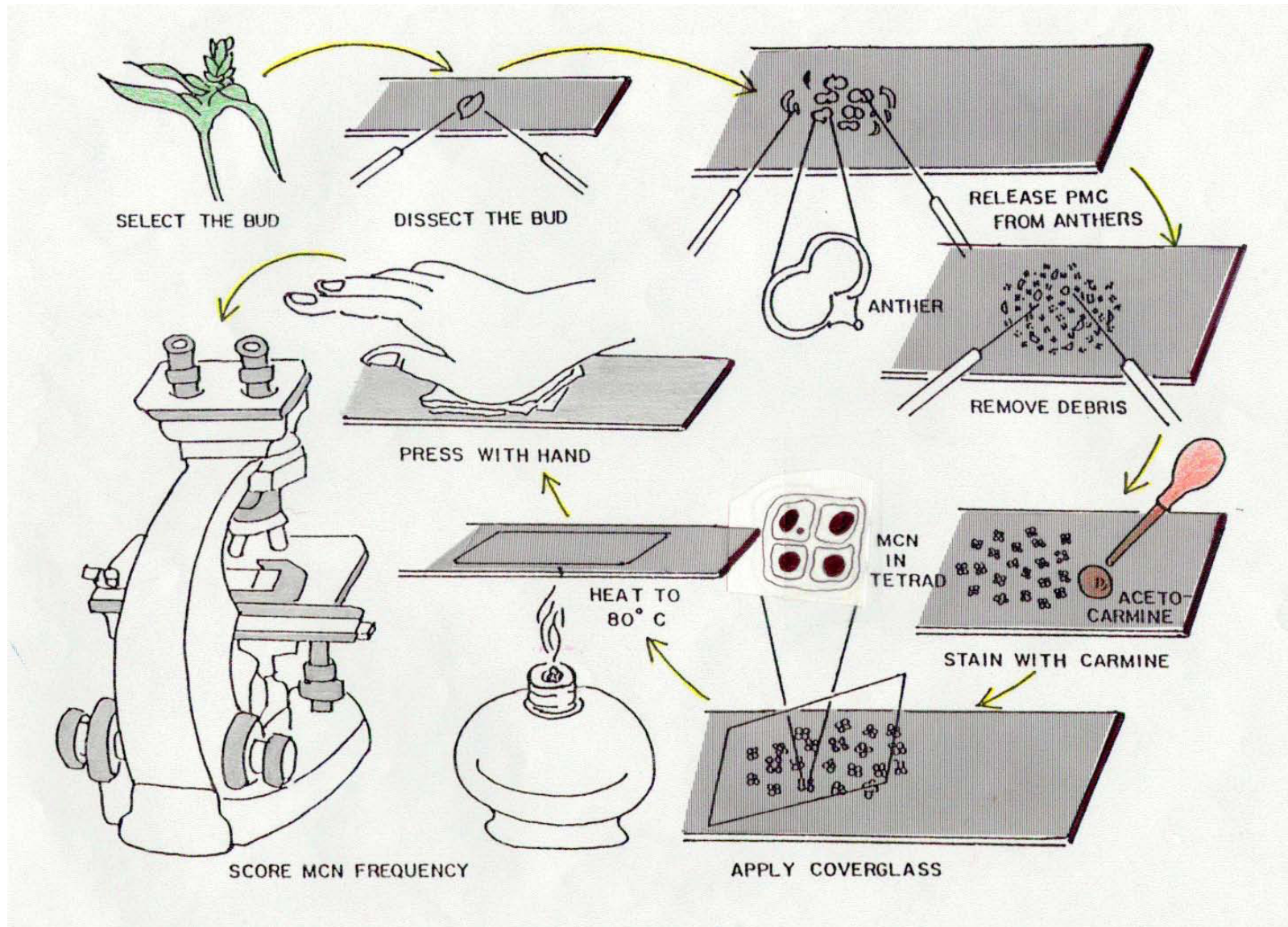
Figure 12 : Protocole du test Tradescantia-MCN d'après Ma et al. , 1981
