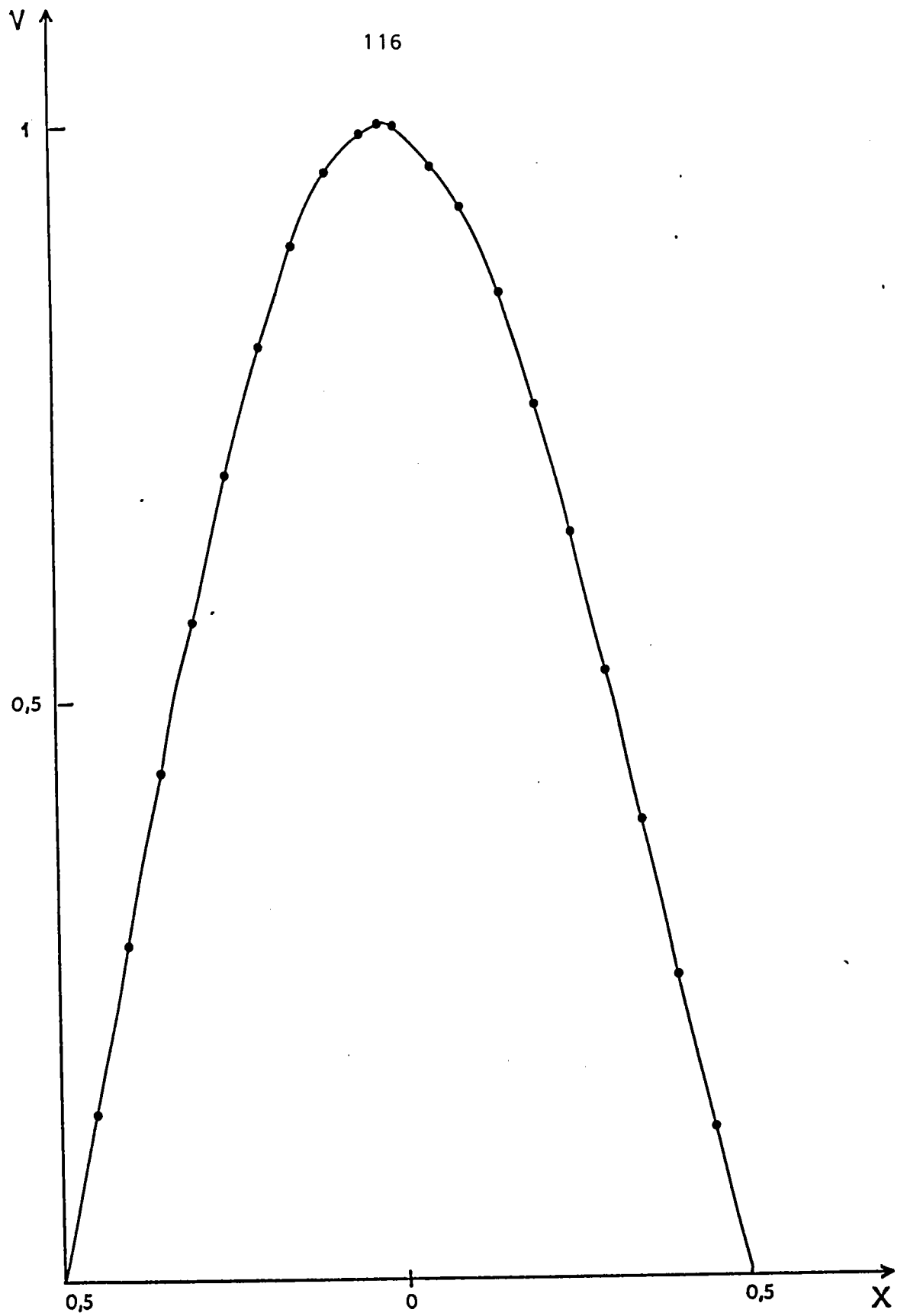
Figure 2.h : Champ des vitesses tangentiellees normalisees du mouvement secondaire .
