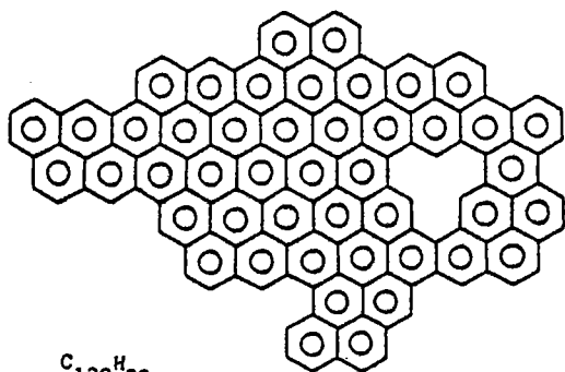
C 130 H 38
