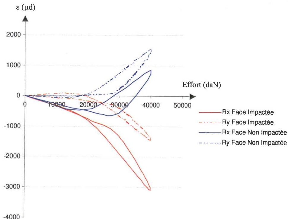
Figure A15 : Résultats expérimentaux en compression dominante sur une éprouvette biaxiale non impactée (éprouvette T1_01 - rapport de biaxialité de 0.344)
