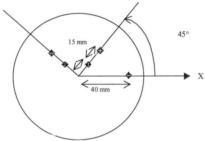
Figure P3-1 : Epruvettes de type 1
