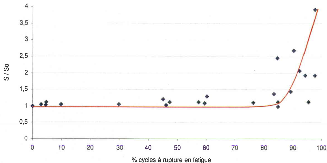
Figure A63 : Evolution de la surface délaminée
