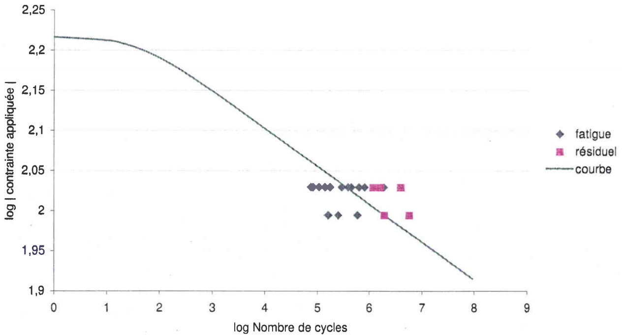
Figure A56 : Courbe de fatigue du drapage 2
