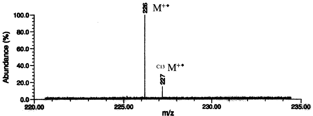
Figure 32 : Spectre FTICRMS Haute Résolution du complexe Benzo[ghi]fluoranthène/C3-DBT-TNF à 193nm [ < 2 \cdot 10^7 \text{ W/cm}^2 ].
