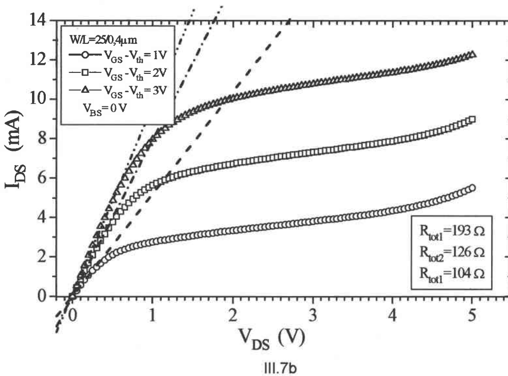
Figure III.7 : Mesure des résistances totales R_{tot} pour différentes polarisations de grille (V_{GS} - V_{th}) = 1, 2 et 3 \text{ V} dans le cas des transistors de W/L = 25/25 \mu m et de W/L = 25/0,4 \mu m .
