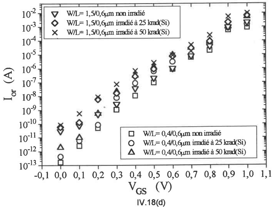
Figure IV.18 : Courant de recombinaison en fonction de la polarisation de grille pour les transistors (a) W=25\mu m , (b) W=0,6\mu m , (c) L=25\mu m et (d) L=0,6\mu m avant et après irradiation.
