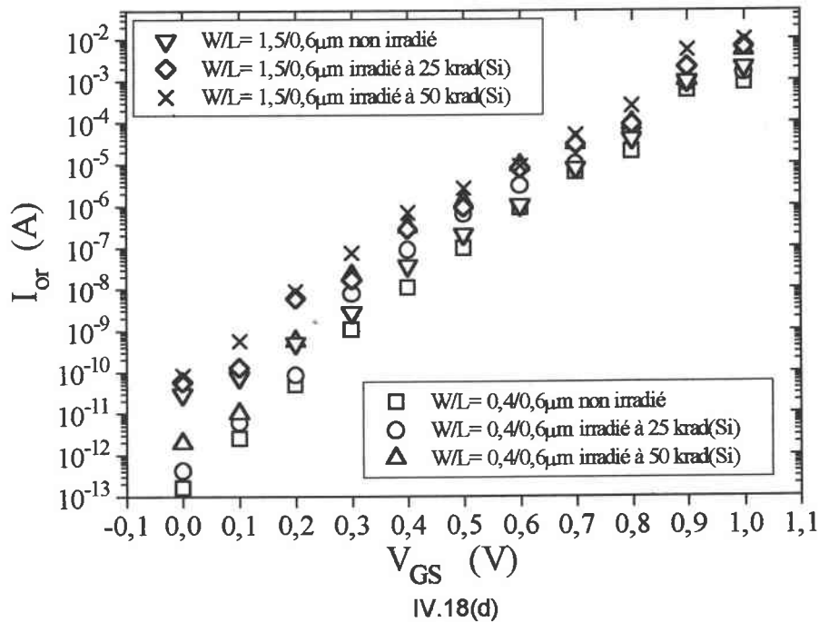
Figure IV.18 : Courant de recombinaison en fonction de la polarisation de grille pour les transistors (a) W=25\mu m , (b) W=0,6\mu m , (c) L=25\mu m et (d) L=0,6\mu m avant et après irradiation.
