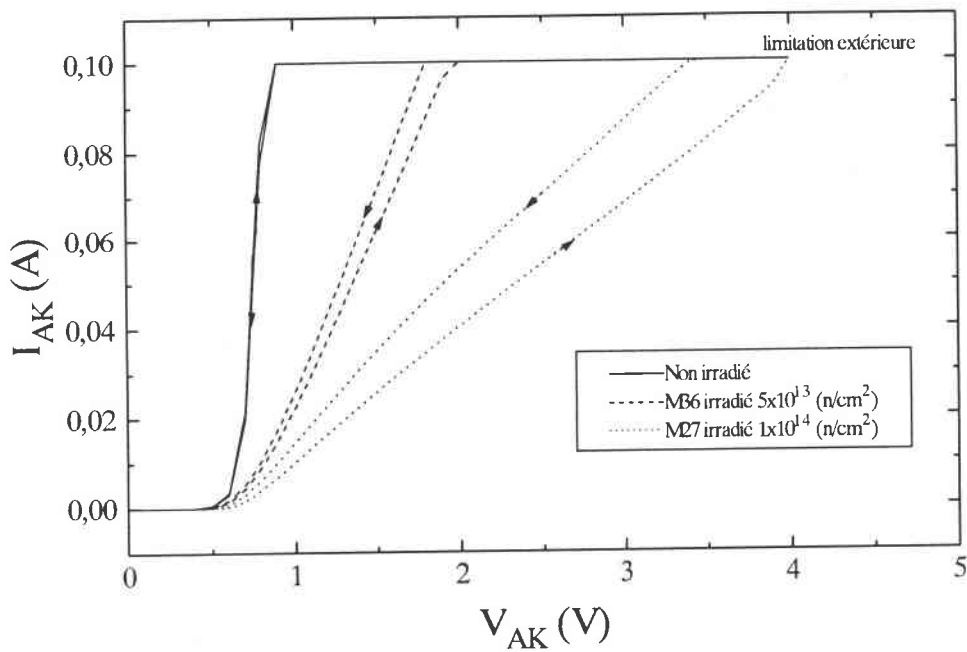
Figure III.18 : Caractéristiques de sortie du MCT pour V_{GA} = -2,2V .
