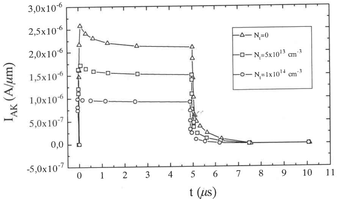
Figure IV.26 : Formes d'ondes simulées, en ouverture et en fermeture, pour le MCT non irradié et les deux densités de pièges simulées.
