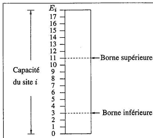
FIG. 4.3: Les bornes calculées par simulation.
