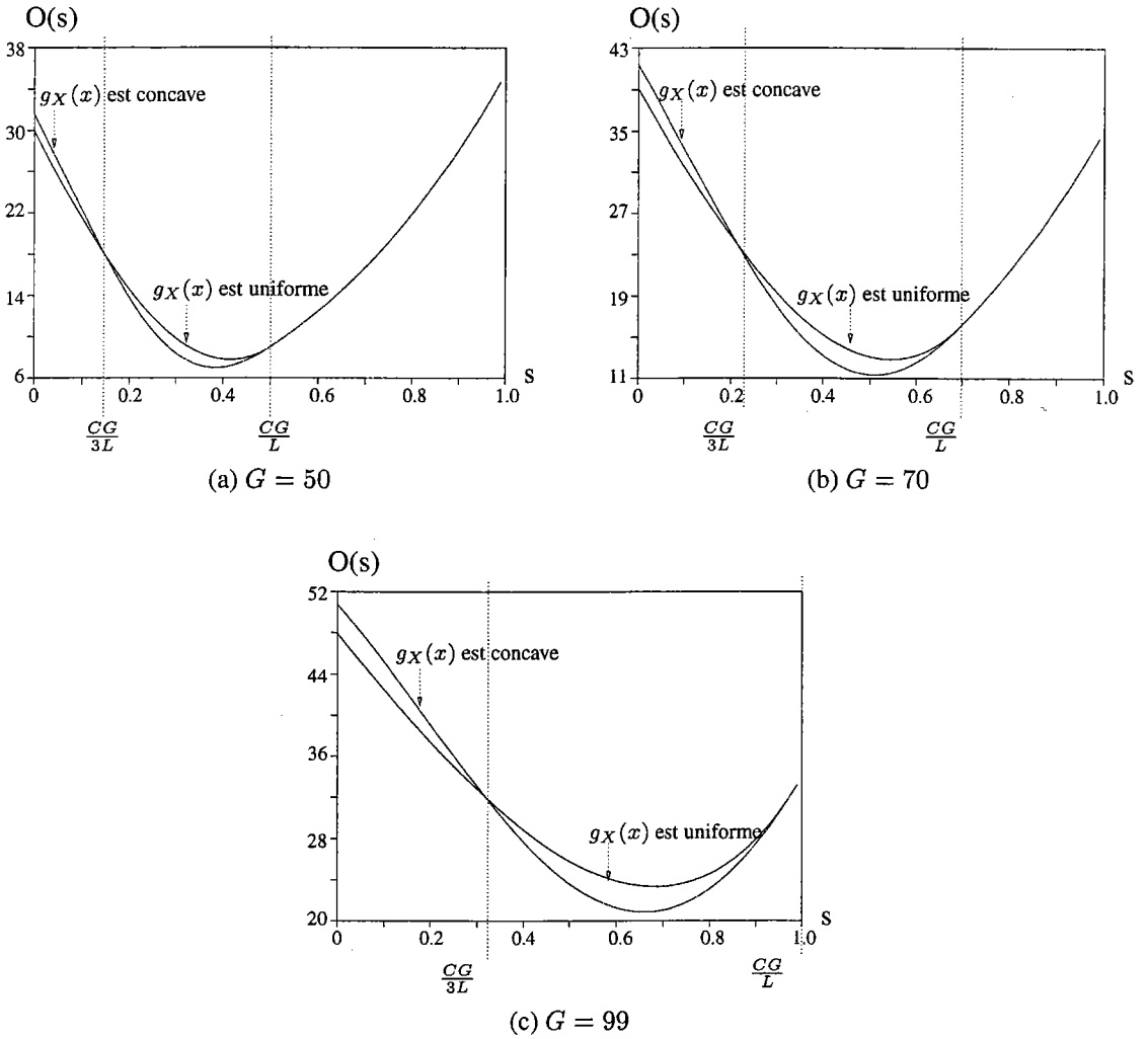
FIG. 1.9: Une comparaison entre deux tracés de O(s) en faisant varier leur g_X(x) , de même qu'en faisant varier le paramètre G .
