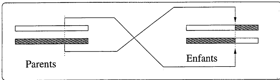
FIG. 1.7: Illustration de l'algorithme ONE POINT CROSSOVER.
