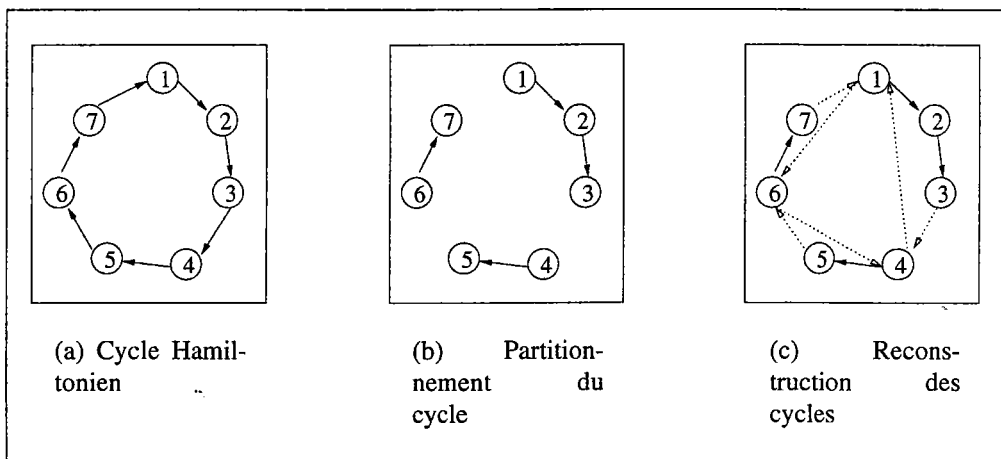
FIG. 4.6: Illustration de la première heuristique
