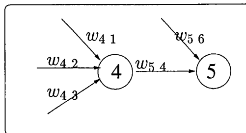
FIG. 1.8: Un réseau de neurones
