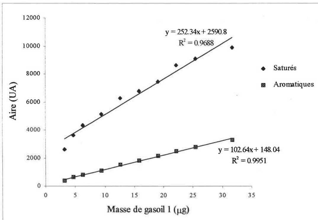
Figure 43 : Droites d'étalonnage direct des fractions aromatiques et saturées pour un intervalle de 3 à 30 \mu\text{g} de gasoil 1 (UA : unités arbitraires).
