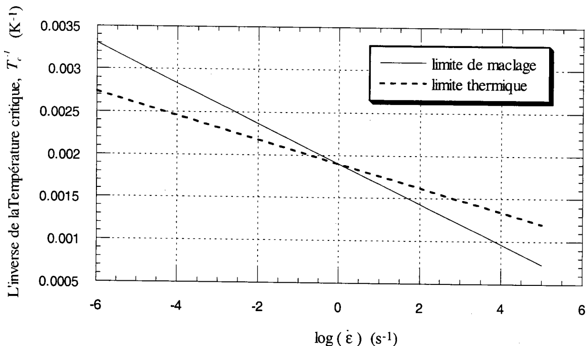
figure VI.9 Les deux domaines, limite de maillage et limite du mouvement des dislocation par activation thermique.
