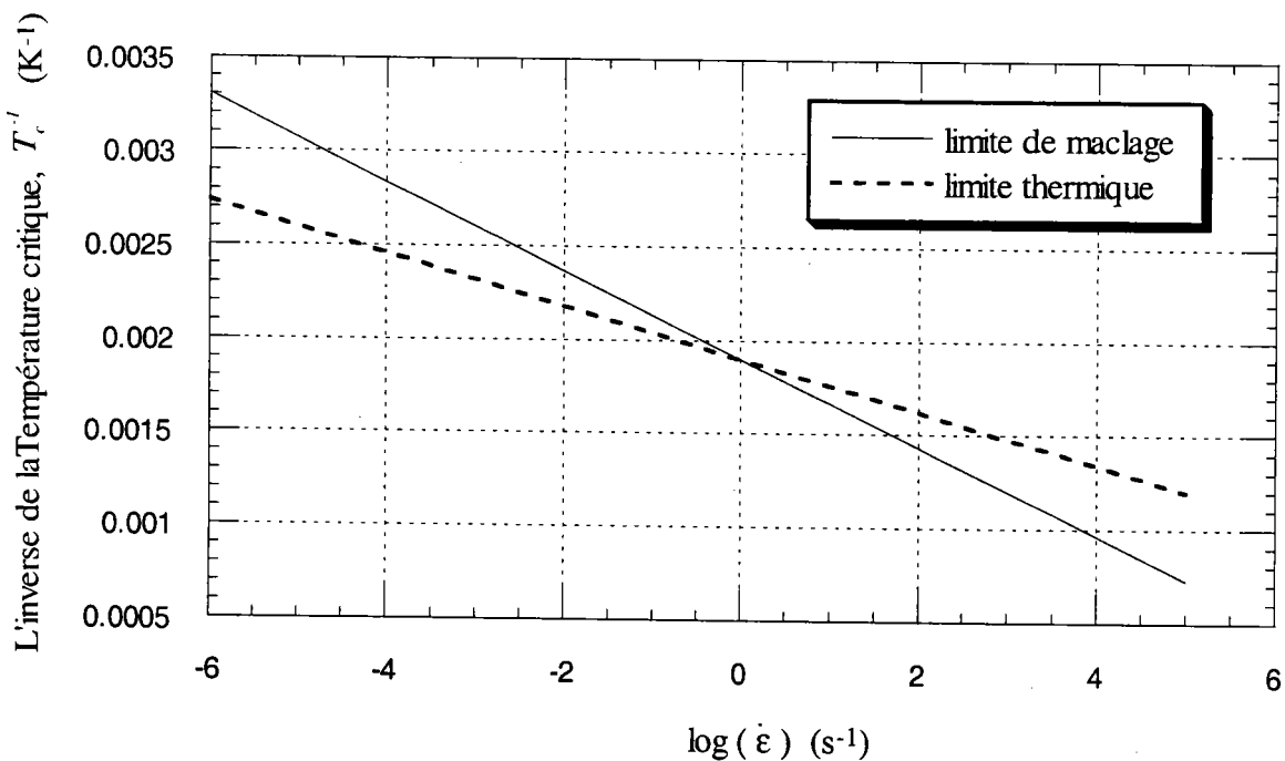
figure VI.9 Les deux domaines, limite de maillage et limite du mouvement des dislocation par activation thermique.
