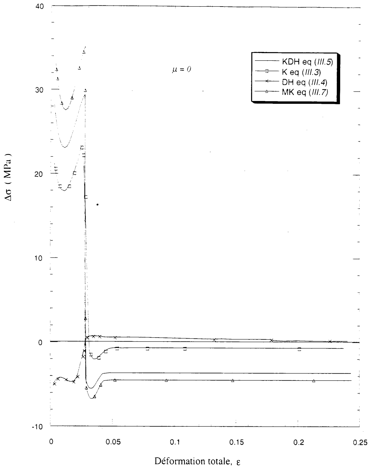
figure III.5a La correction de l'effet de l'inertie pour le titane pour la première vitesse de déformation \dot{\epsilon}_1 et s_0 = 0,5 .
