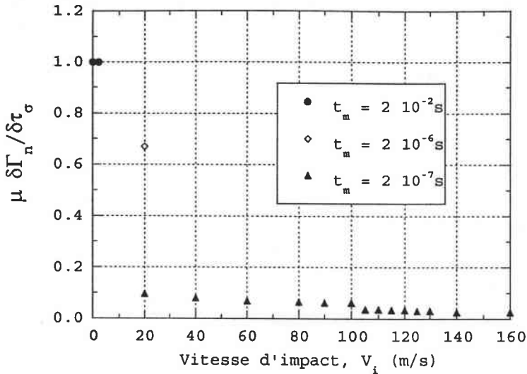
Fig. 3.27 Pentes nominales des courbes \tau_A(\Gamma)
