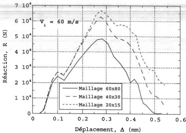
Fig. 4.24 Influence de la densité du maillage sur le comportement global de l'éprouvette (courbes R- \Delta )
