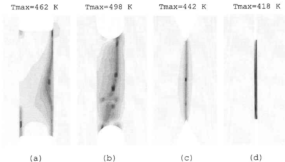
Fig. 4.17 Champs des températures au moment de la rupture: (a) géométrie standard, (b) entaille en U, (c) entaille en V, (d) entaille fine
