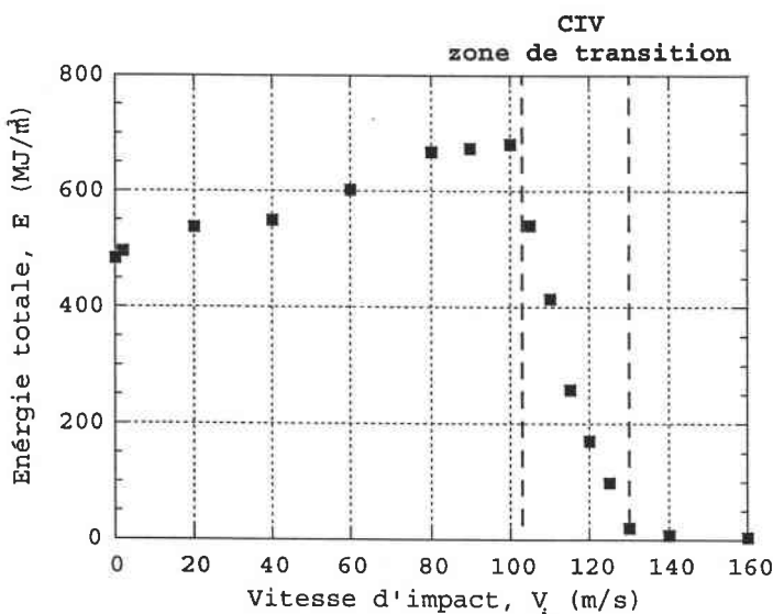
Fig. 3.31 Énergie plastique dissipée jusqu'à la rupture en fonction de la vitesse d'impact V_i
