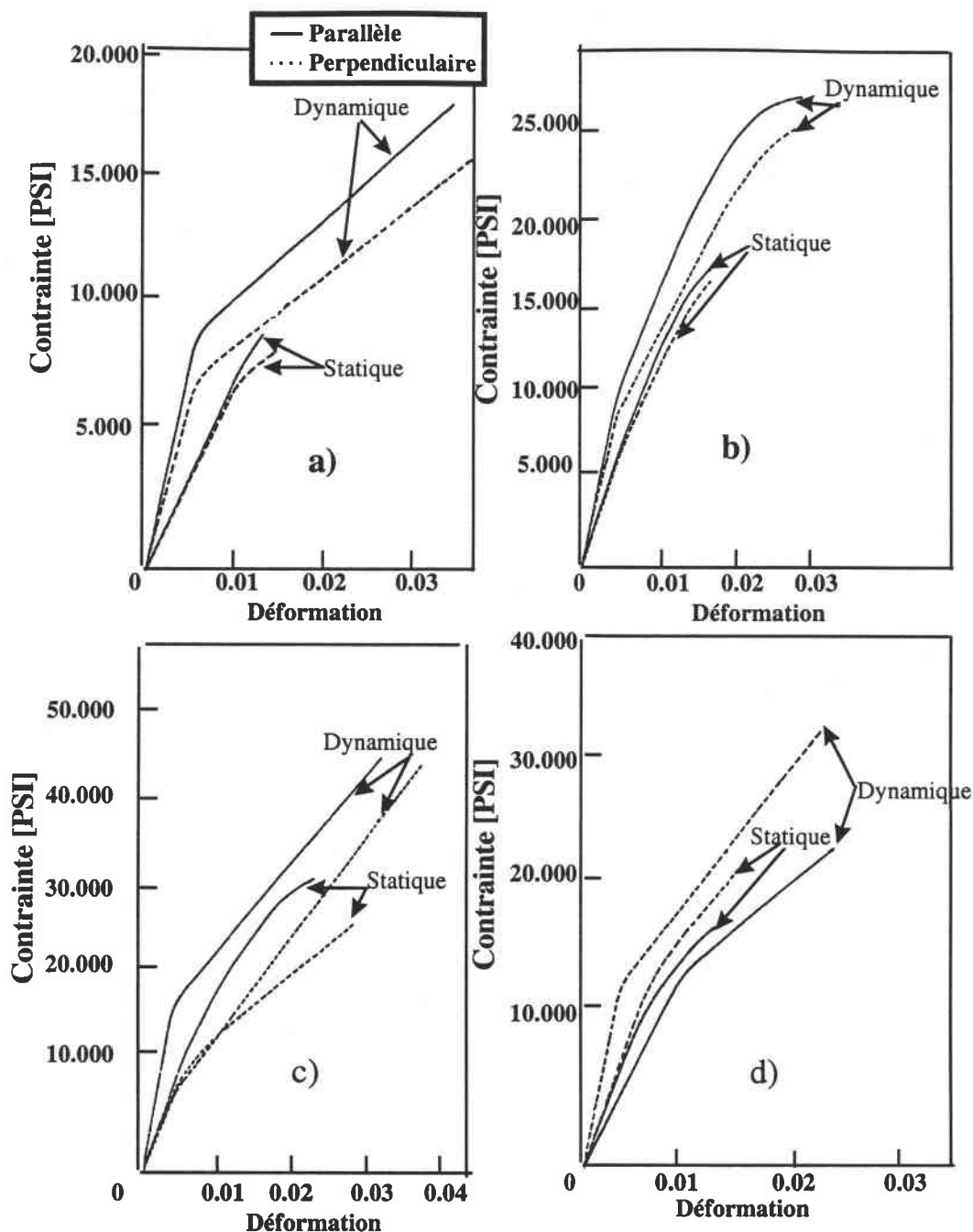
Figure 1-43 : Courbes contrainte-déformation en traction dynamique et statique pour les composites verres/polyester (dynamique : 150 \text{ 1/s} , statique : 0.1 \text{ 1/s} ) a) Renfort en fibres courtes (épaisseur de l'échantillon 1/8 pouce) b) Renfort en fibres courtes (épaisseur de l'échantillon 1/4 pouce) c) Renfort en 'roving tissé' (1/8 pouce) d) Renfort en tissu équilibré 1/8 pouce), [45].
