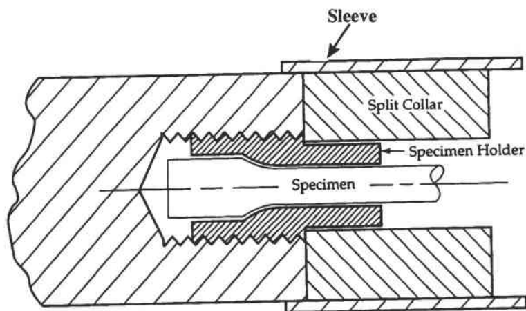
Figure 1-5 : Éprouvette haltère pour des essais de traction dynamique [7].
