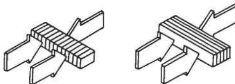
a) Cisaillement interlaminaire b) Cisaillement transversal
