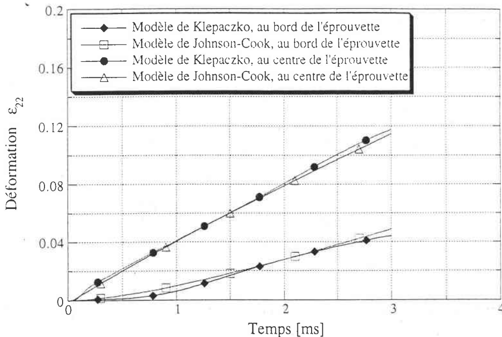
Figure VI.28 : Evolutions temporelles de la déformation \epsilon_{22} au bord et au centre de l'éprouvette.
