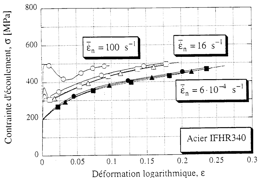
Figure II.17 : Ensemble des résultats des essais de traction réalisés sur la machine pour les deux vitesses de déformation \bar{\epsilon}_n = 6 \cdot 10^{-4} s^{-1} et \bar{\epsilon}_n = 16 s^{-1} et de l'essai réalisé sur les barres pour la vitesse \bar{\epsilon}_n = 100 s^{-1} .
