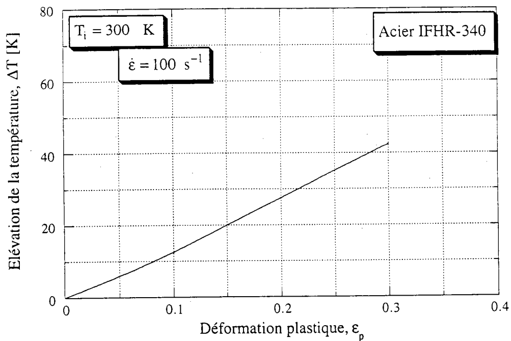
Figure III.33 : Elévation hypothétique de la température au cours de la déformation dans le cas de l'approximation adiabatique pour une vitesse de déformation \dot{\epsilon} = 100 s ^{-1} et une température initiale T_i = 300 K.
