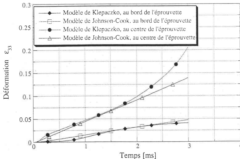
Figure VI.29 : Evolutions temporelles de la déformation \epsilon_{33} au bord et au centre de l'éprouvette.
