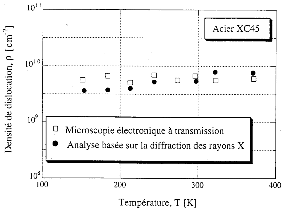
Figure I.20 : Variations de la densité moyenne de dislocations en fonction de la température pour un acier XC45 ( \epsilon_p = 5\% et \dot{\epsilon} = 3 \times 10^{-3} \text{ s}^{-1} ), Burgahn et coll. [35].
