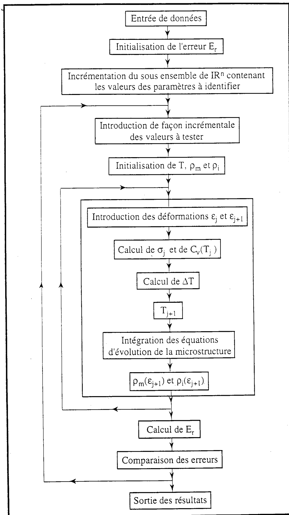
Figure III.4 : Schéma de la procédure utilisée pour l'identification des paramètres.
