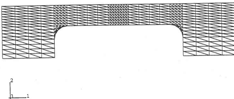
Figure VI.2 : Discrétisation spatiale de l'éprouvette de traction.
