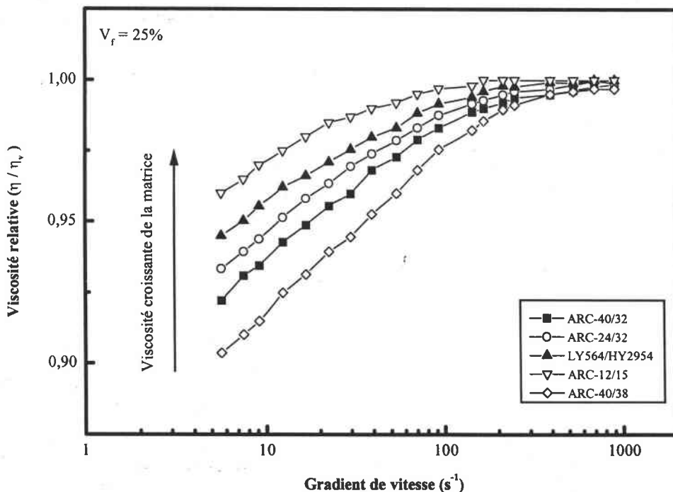
Figure III.C.9 : Evolution de la viscosité relative en fonction de la viscosité de la matrice (Cellule de Couette S1/S, fibres de carbone T300-ml, V f = 25%)
