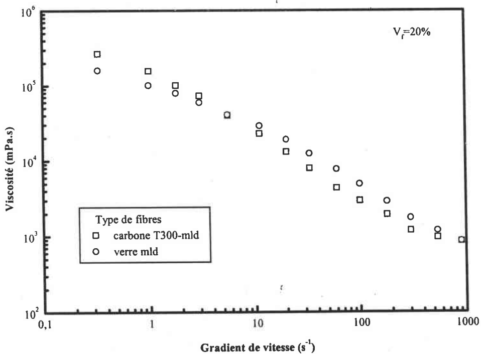
Figure III.B.15 : Comparaison du comportement rhéologique entre un mélange à base de fibres de carbone T300-mld et un mélange à base de fibres de verre (résine ARC-40/32, taux de charges de 20%, cellule cône plan)
