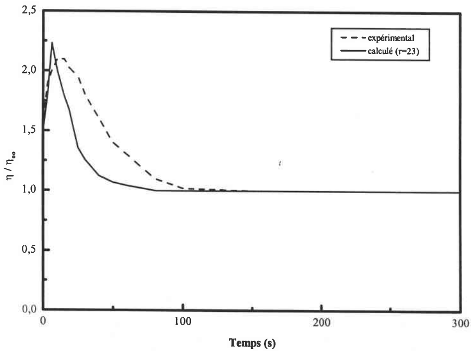
Figure V.B.3 : Modélisation du pic de viscosité dans le cas d'un composite chargé à 30%. (résine ARC-40/32, fibres T300-mld, \dot{\gamma} = 20 \text{ s}^{-1} )
