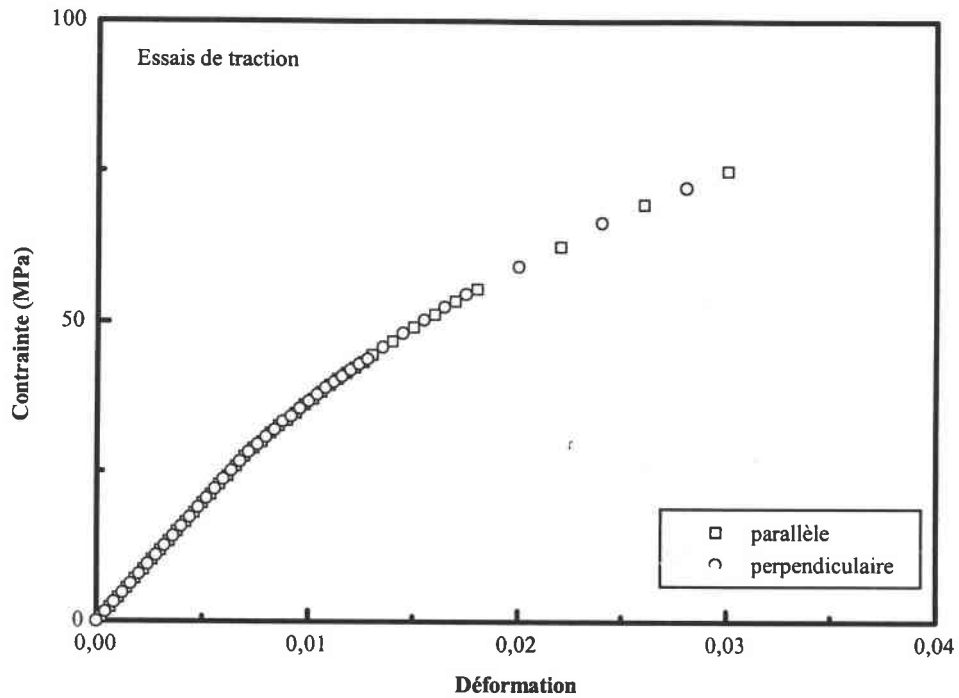
Figure IV.B.37 : Influence de la direction de découpes des éprouvettes de traction sur les propriétés mécaniques de la résine époxyde ARC-40/32.
