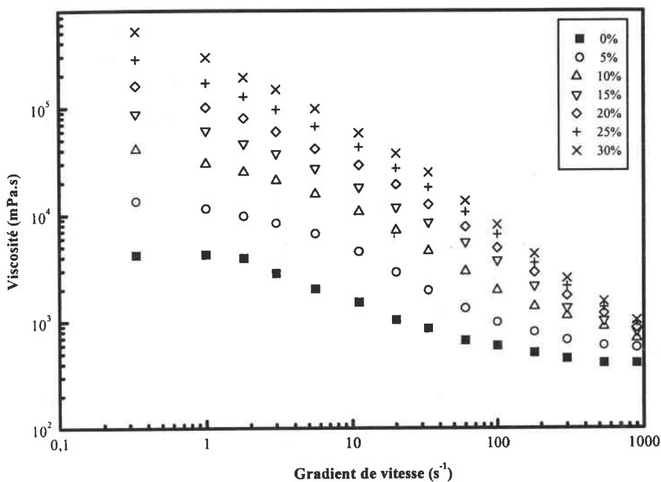
Figure III.B.14 : Viscosité de la résine ARC-40/32 en fonction du taux de charges en fibres de verre (essais en cellule cône-plan)
