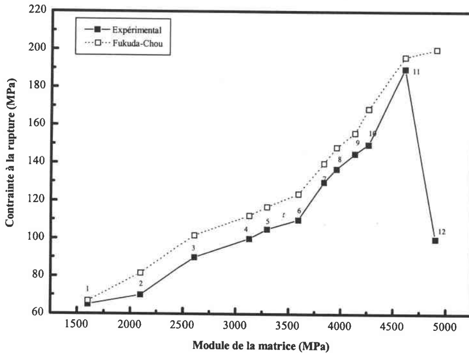
Figure V.C.8 : Contrainte à la rupture en fonction du module de la matrice (fibres T300-mld, V_f = 30\% )
