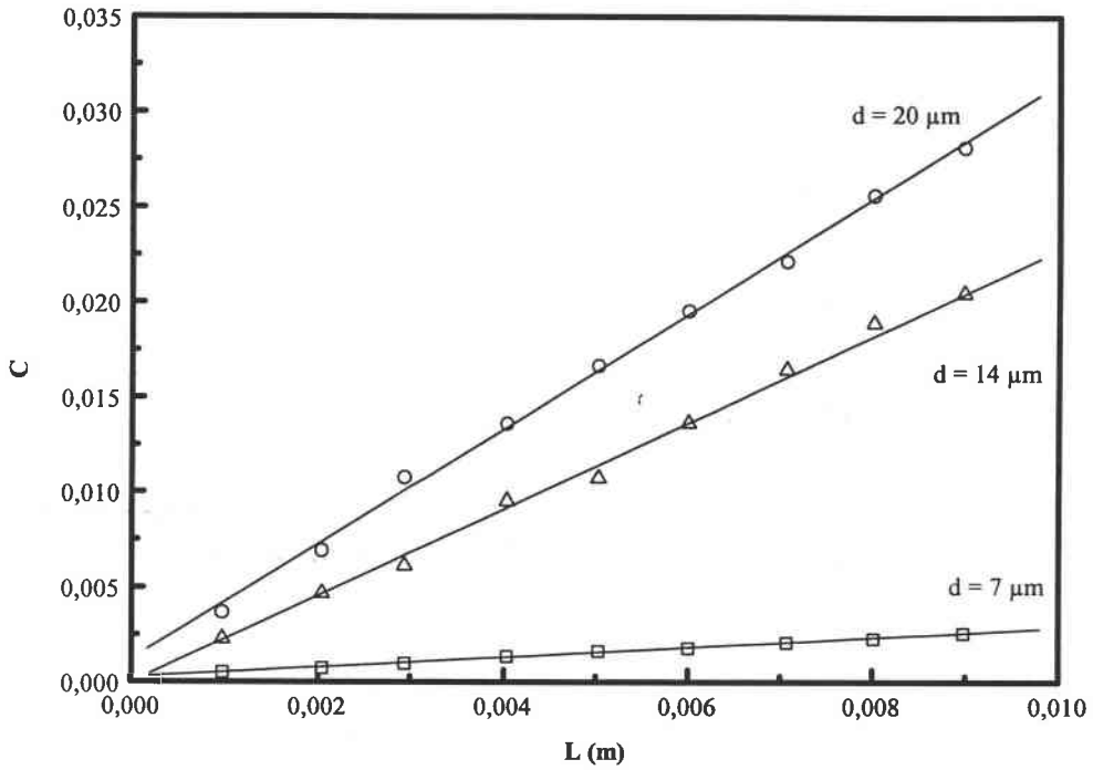
Figure V.A.2 : Evolution du coefficient de frottement en fonction de la longueur des fibres dans le glycérol (1 Pa.s)
