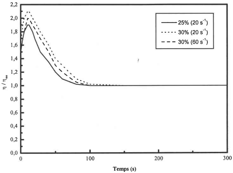
Figure III.B.21 : Mesure du pic de viscosité pour un mélange composite à base de la résine ARC-40/32 chargées à 25% et 30% en fibres de carbone T300-mld (cellule cône-plan, gradient de vitesse : 20 s -1 et 60 s -1 )
