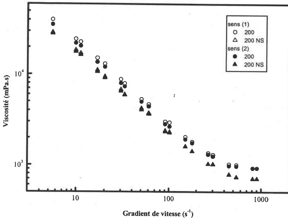
Figure III.B.13 : Mesure de la viscosité à gradient croissant (1) et à gradient décroissant (2) pour un mélange ARC-40/32 chargé à 20 % de fibres de carbone T300-200. (cellule de Couette S1/S)
