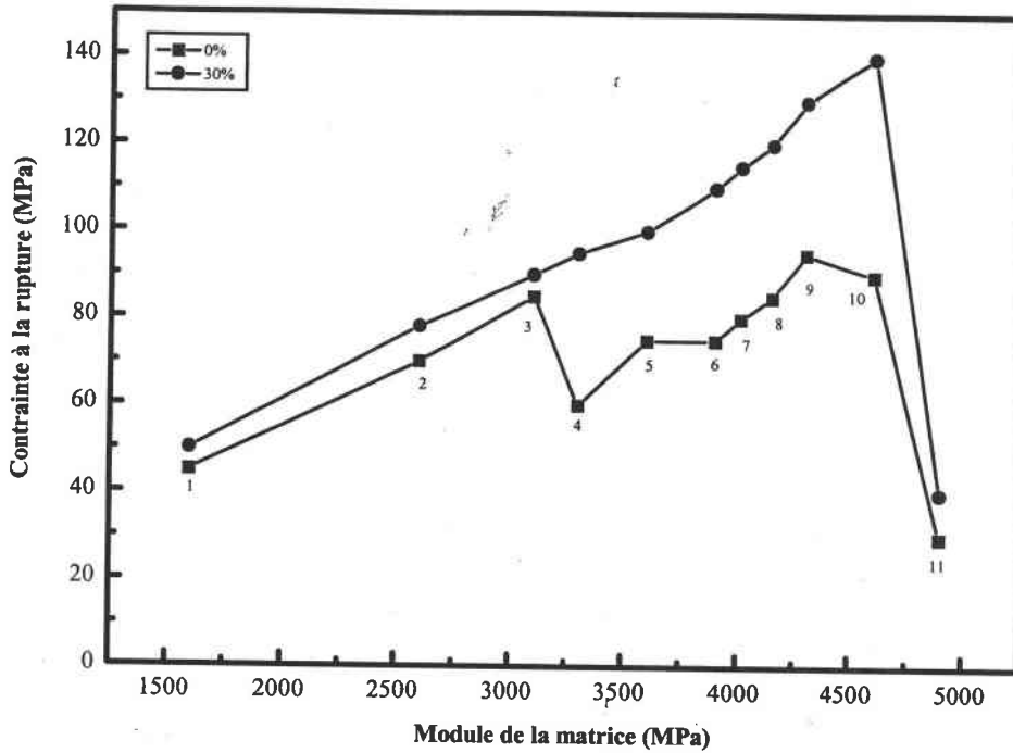
Figure IV.B.28 : Influence de la matrice sur la contrainte à la rupture en traction du matériau composite (fibres de carbone T300-200, vitesse d'essai : 1mm/min)
