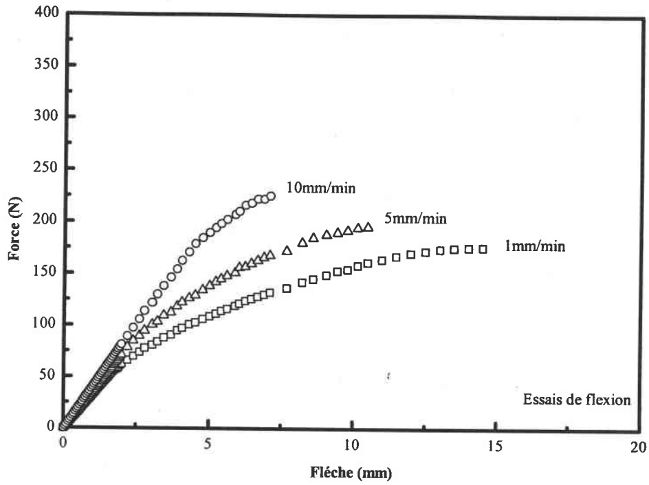
Figure IV.B.31 : Influence de la vitesse d'essai sur les propriétés mécaniques en flexion de la résine époxyde ARC-40/32
