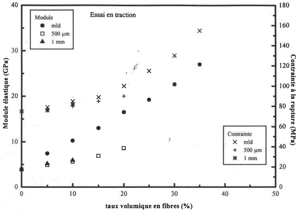
Figure IV.B.18 : Evolution des propriétés mécaniques en traction en fonction du taux de charges en fibres et de la longueur des fibres de carbone T300 (résine ARC-40/32, vitesse d'essai : 1mm/min)
