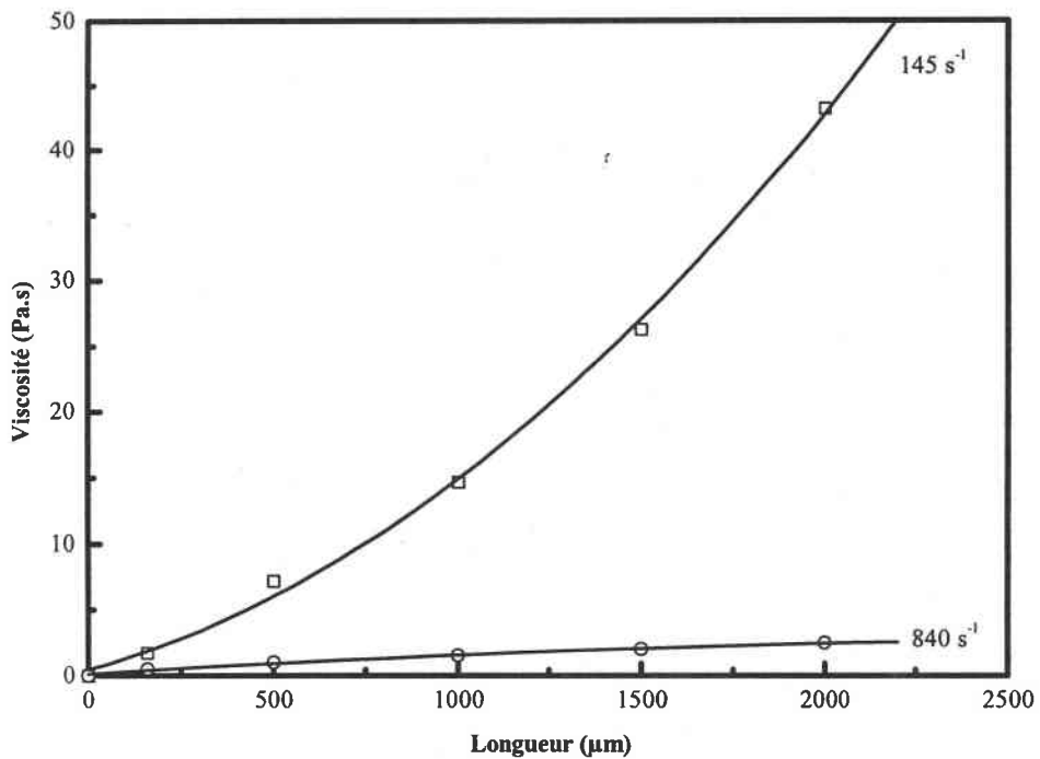
Figure III.B.7 : Influence de la longueur des fibres de carbone T300 sur la viscosité du composite ARC-40/32 chargé à 15 % en volume pour des gradients de vitesse de 145 \text{ s}^{-1} (□) et 840 \text{ s}^{-1} (○) (cellule de Couette S1/S)
