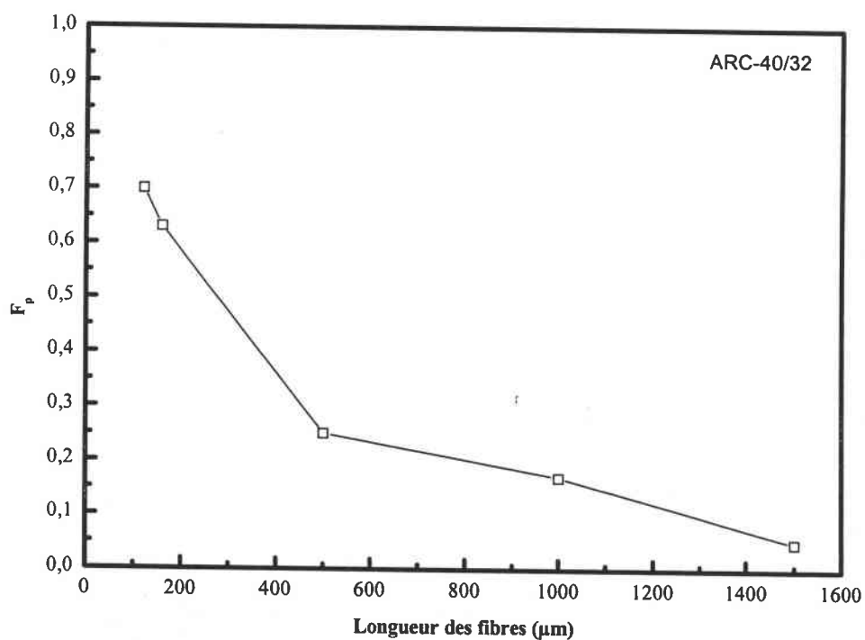
Figure IV.B.4 : Influence du rapport de forme des fibres sur le facteur d'orientation (Résine ARC-40/32 chargée à 10% en fibres de carbone T300)
