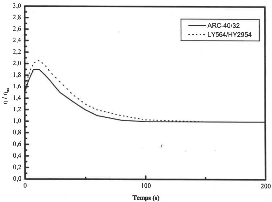
Figure III.B.25 : Influence de la matrice sur le pic de viscosité. ARC-40/32 et LY564/HY2954 chargées à 25% de fibres T300-mld. (cellule cône-plan, gradient de vitesse : 20 \text{ s}^{-1} )
