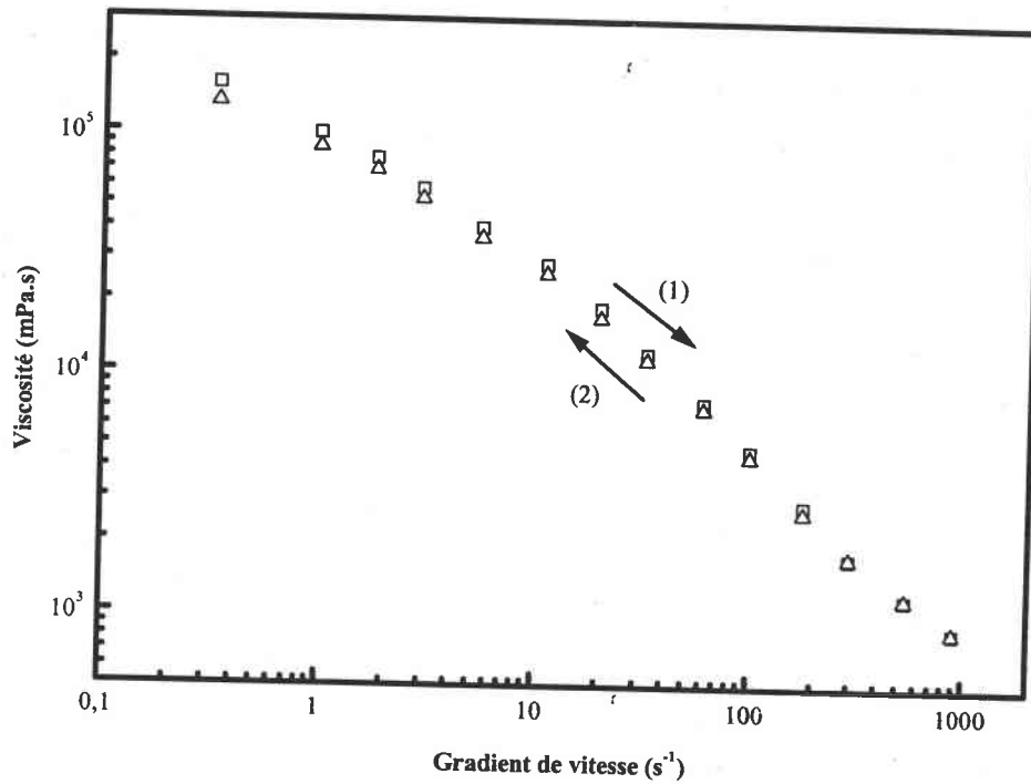
Figure III.B.16 : Mesure de la viscosité à gradient croissant (1) et à gradient décroissant (2) pour un mélange ARC-40/32 chargé à 20 % de fibres de verre. (cellule de Couette S1/S)
