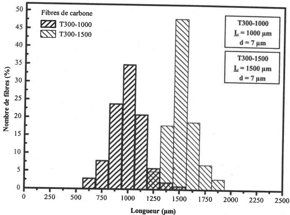
Figure I.A.13 : Distribution en longueur des fibres de carbone T300-1000 et T300-1500 (APPLY Carbon SA)
