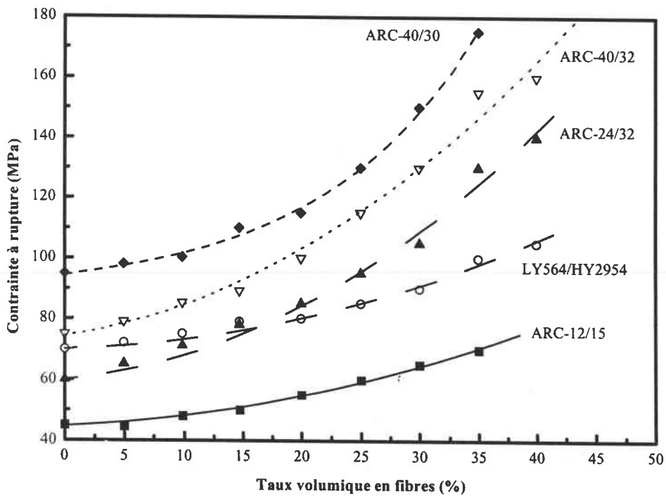
Figure IV.B.13 : Evolution de la contrainte à la rupture en traction en fonction du taux de charges en fibres de carbone T300-mld (vitesse d'essai : 1mm/min)
