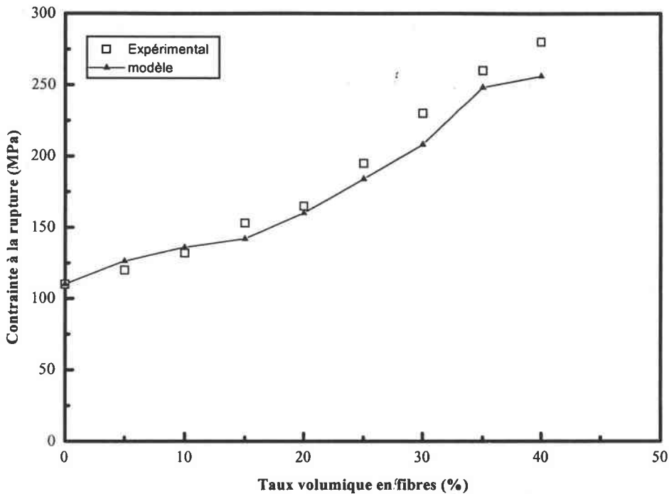
Figure V.C.11 : Modélisation de la contrainte à la rupture en fonction du taux de fibres (ARC-40/32, fibres T300-ml).
