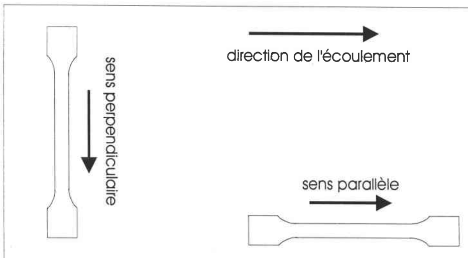
Figure IV.B.36 : Représentation des deux orientations principales de découpes des éprouvettes d'essais mécaniques dans la plaque composite.
