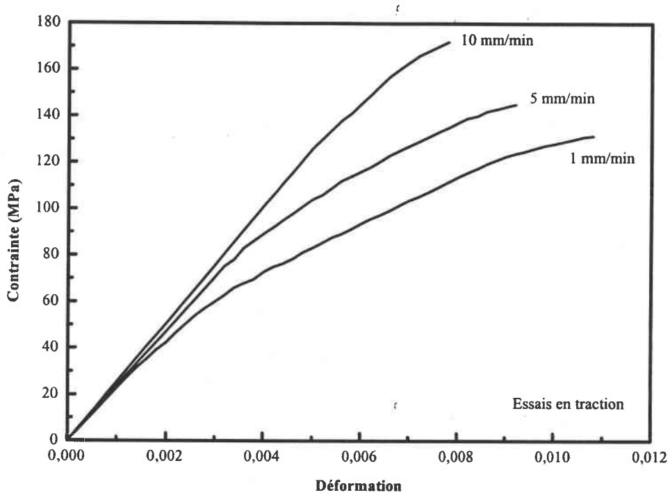
Figure IV.B.33 : Influence de la vitesse d'essai sur les propriétés mécaniques en traction de la résine époxyde ARC-40/32 chargée avec 30% de fibres de carbone T300-ml
