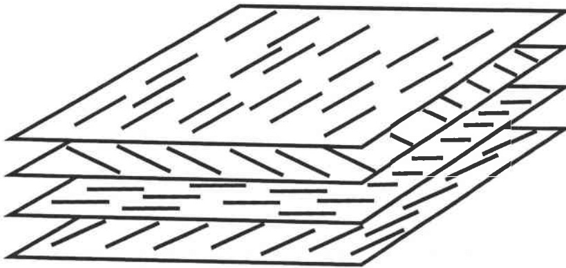
Figure IV.A.12 : Représentation schématique d'un composite "quasi-isotrope" selon HALPIN-KARDOS [1972]
