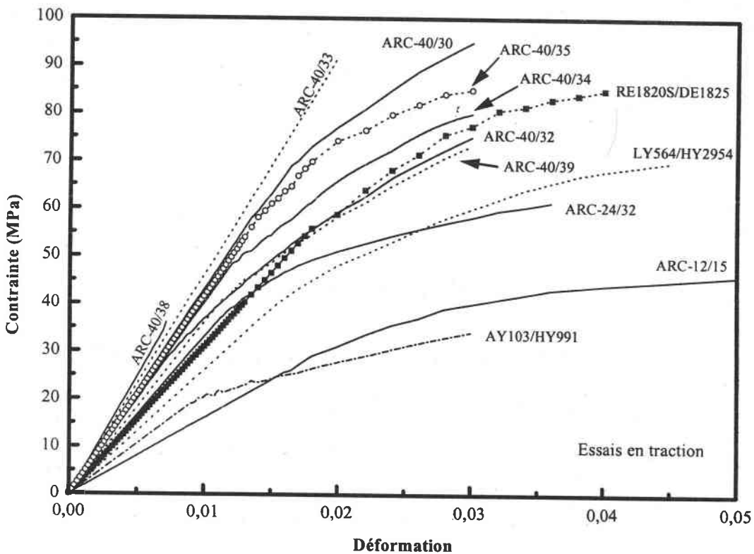
Figure I.A.3 : Courbes (Contrainte / Déformation) en essais de traction pour les différentes résines.
