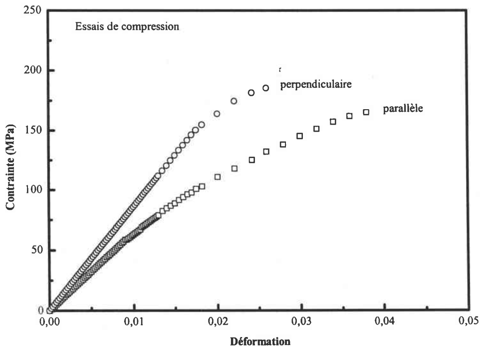
Figure IV.B.42 : Influence de la direction de découpe des éprouvettes de compression sur les propriétés mécaniques de la résine époxyde ARC-40/32 chargées à 20% de fibres de carbone T300-ml d ( F_p = 0,4 ).
