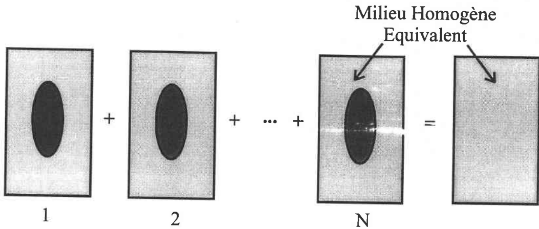
Figure IV.A.5 : Représentation du modèle autocohérent
