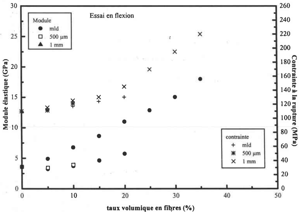
Figure IV.B.19 : Evolution des propriétés mécaniques en flexion en fonction du taux de charges en fibres et de la longueur des fibres de carbone T300 (résine ARC-40/32, vitesse d'essai : 1mm/min)
