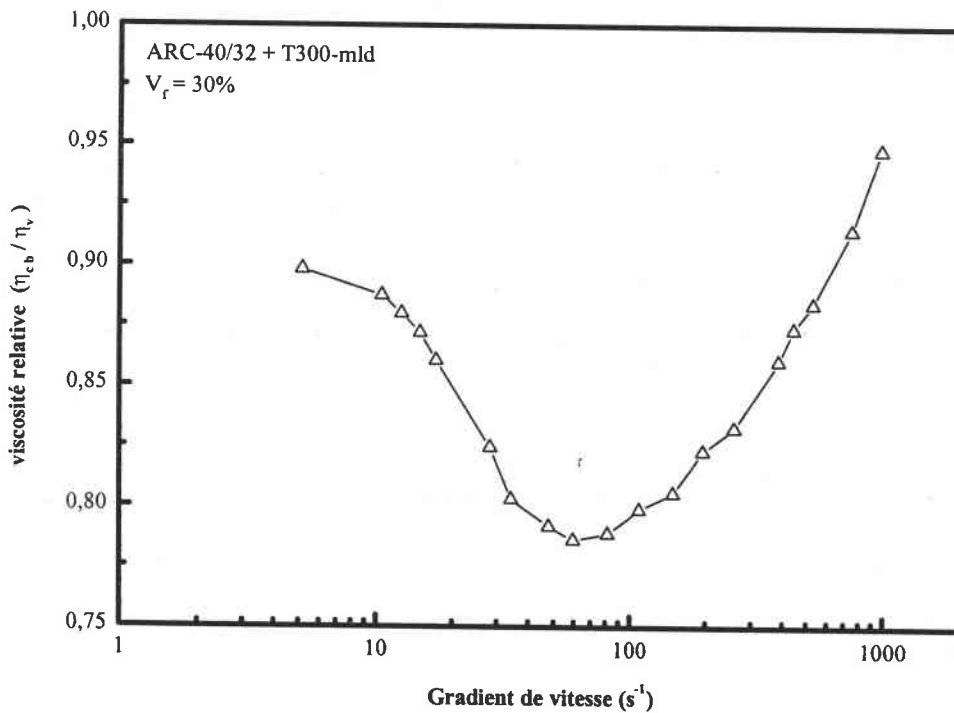
Figure III.C.16 : Evolution de la viscosité relative lors de l'ajout d'un faible taux de microbilles (1%) dans la résine ARC-40/32 chargée avec 30% de fibres de carbone T300-mld (cellule de Couette S1/S)
