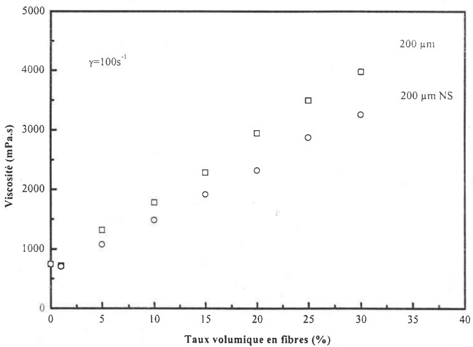
Figure III.B.12 : Influence de l'ensimage sur la viscosité d'un mélange à base de la résine époxyde ARC-40/32. (cellule de Couette S1/S)
