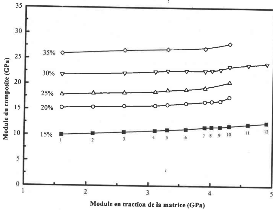
Figure IV.B.24 : Influence de la matrice sur le module en traction du matériau composite (fibres de carbone T300-ml, vitesse d'essai : 1mm/min)
