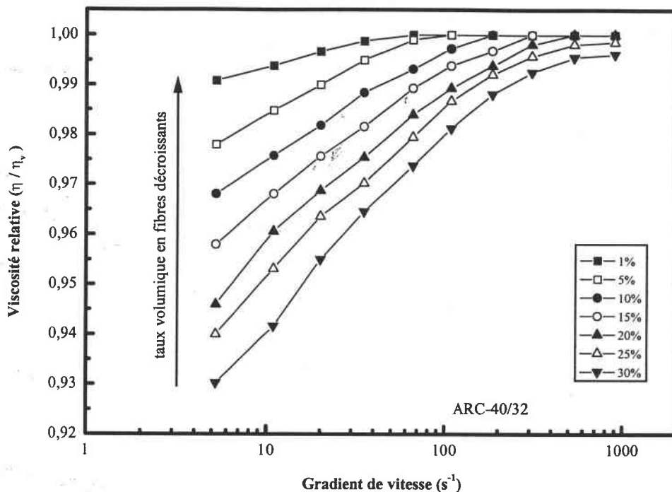
Figure III.C.8 : Evolution de la viscosité relative en fonction de la fraction volumique en fibres de verre (cellule de Couette S1/S, résine ARC-40/32)
