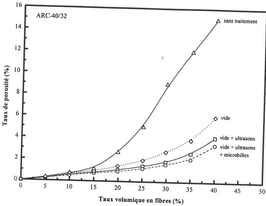
Figure IV.B.1 : Influence de la technique de mélange sur le taux de porosité des matériaux composites chargés en fibres de carbone T300-ml.
