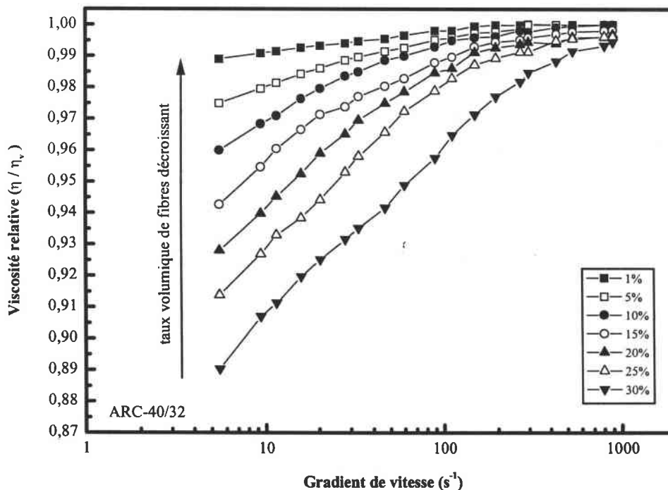
Figure III.C.7 : Evolution de la viscosité relative en fonction de la fraction volumique en fibres de carbone T300-mld. (cellule de Couette S1/S, résine ARC-40/32)
