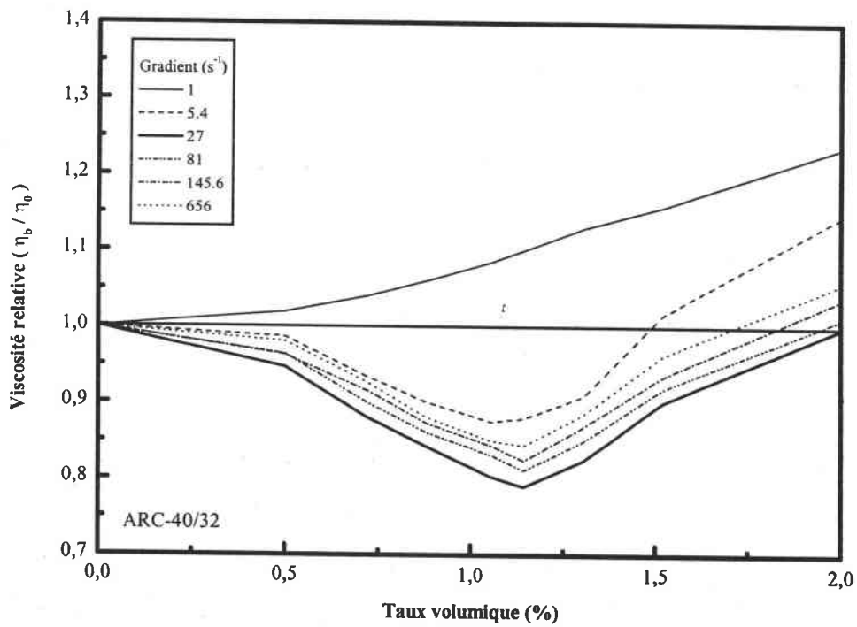
Figure III.C.13 : Influence de la fraction volumique en microbilles de verre K1 sur la viscosité relative de la résine ARC-40/32 (cellule cône-plan)
