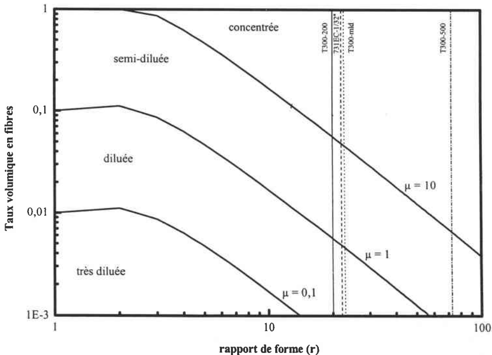
Figure V.B.1 : Les régimes de concentration en fibres
