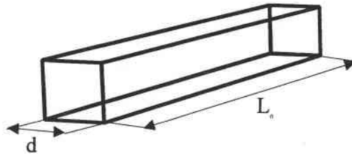
Figure II.E.3 : éprouvette de compression uniaxiale.
