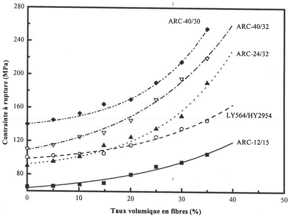
Figure IV.B.15 : Evolution de la contrainte à la rupture en flexion du taux de charges en fibres de carbone T300-mld (vitesse d'essai : 1mm/min)
