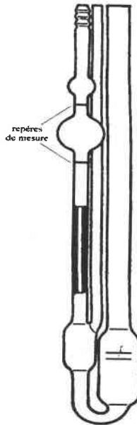
Figure II.A.1 : viscosimètre capillaire de type Ubbelohde
