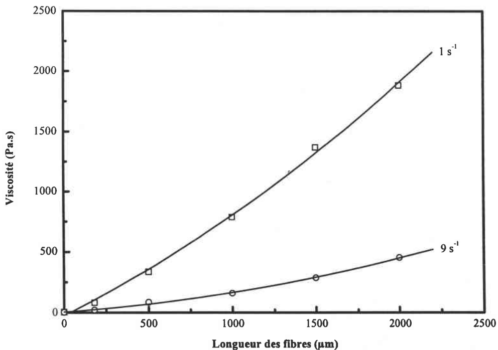
Figure III.B.6 : Influence de la longueur des fibres de carbone T300 sur la viscosité du composite ARC-40/32 chargé à 15 % en volume pour des gradients de vitesse de 1 \text{ s}^{-1} ( \square ) et 9 \text{ s}^{-1} ( \circ ) (cellule de Couette S1/S)
