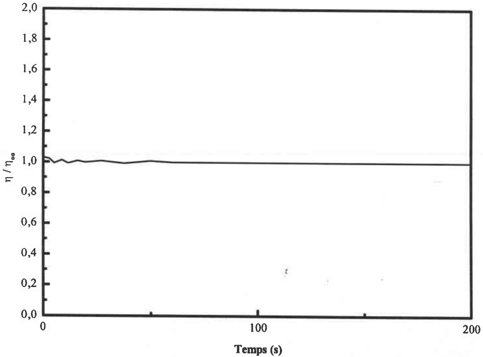
Figure III.B.27 : Mesure du pic de viscosité sur un échantillon précisailé. ARC-40/32 chargée à 25% de fibres T300-mld (cellule cône-plan, gradient de vitesse : 20 s -1 )
