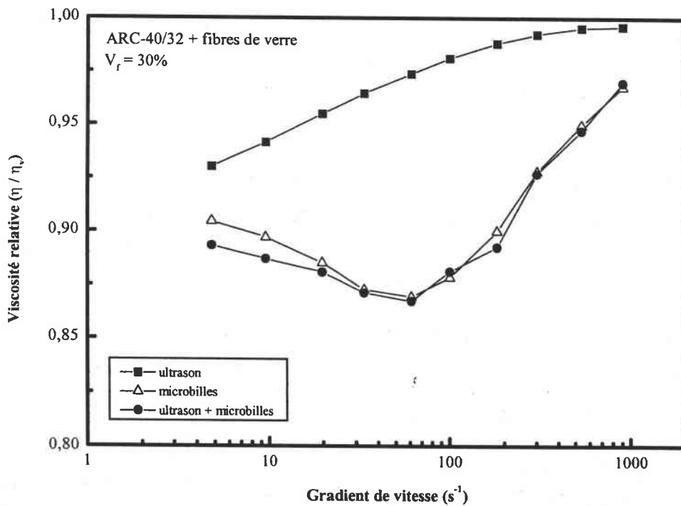
Figure III.C.19 : Influence du traitement sur la viscosité relative d'un mélange composite à base de la résine ARC-40/32 chargée à 30% en fibres de verre (cellule de Couette S1/S)
