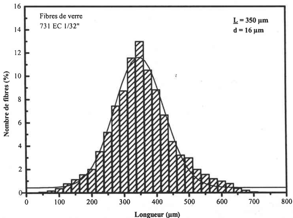
Figure I.A.14 : Distribution en longueur des fibres de verre 731EC1/32" (OWENS CORNING)
