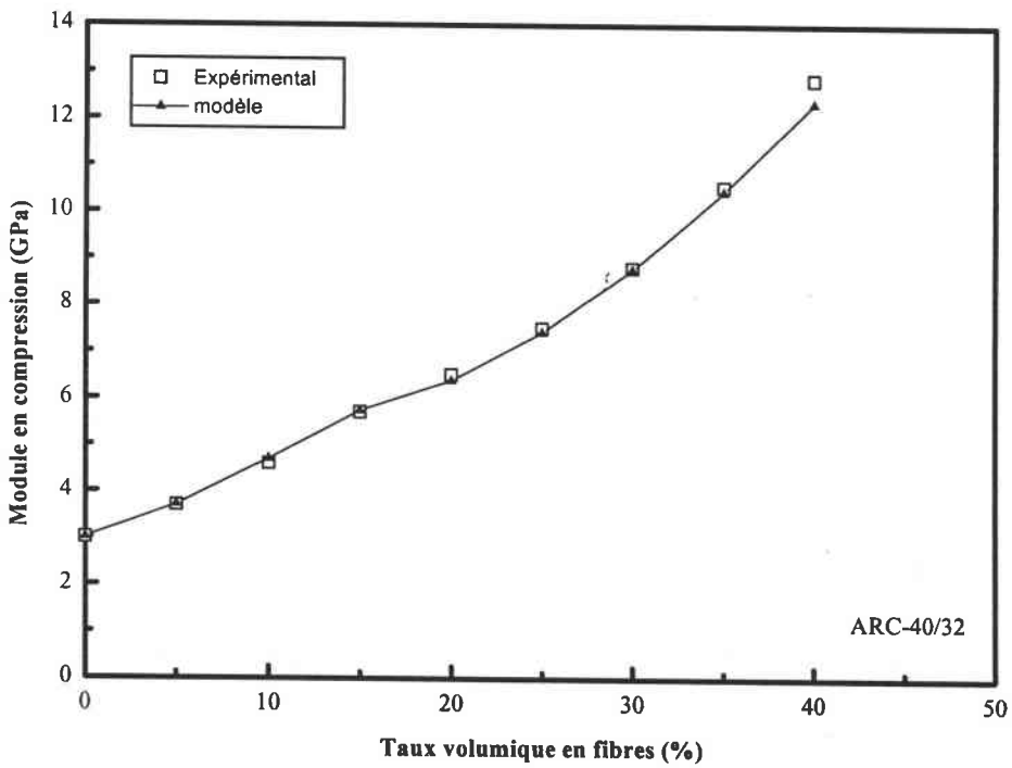
Figure V.C.10 : Modélisation du module en compression en fonction du taux de fibres (ARC-40/32, fibres T300-ml)
