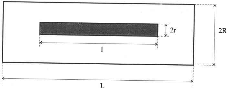
Figure III.A.7 : Géométrie de la cellule étudiée dans le modèle de COX
