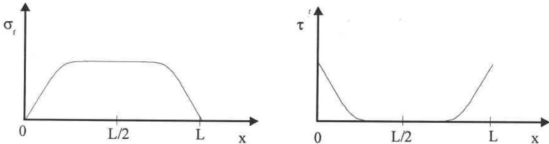
Figure IV.A.10 : Distribution de la contrainte de cisaillement à l'interface et de la contrainte de traction le long d'une fibre de longueur L
