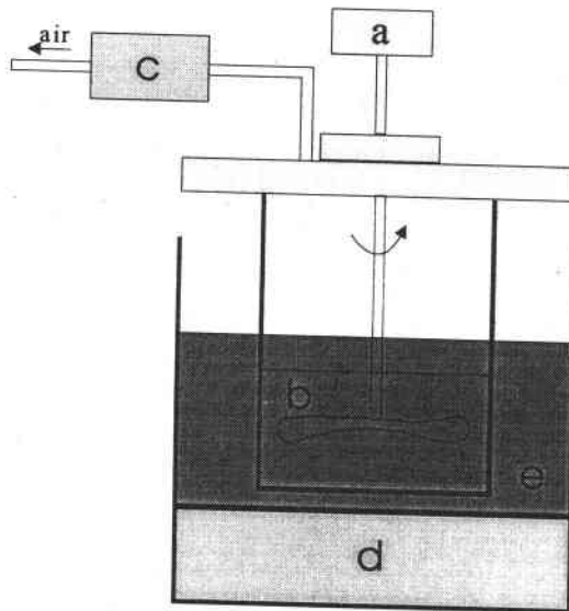
Figure I.B.1 : Dispositif de mélange
