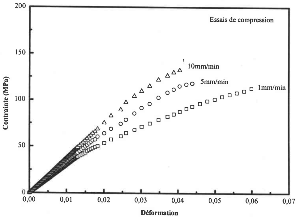
Figure IV.B.32 : Influence de la vitesse d'essai sur les propriétés mécaniques en compression de la résine époxyde ARC-40/32
