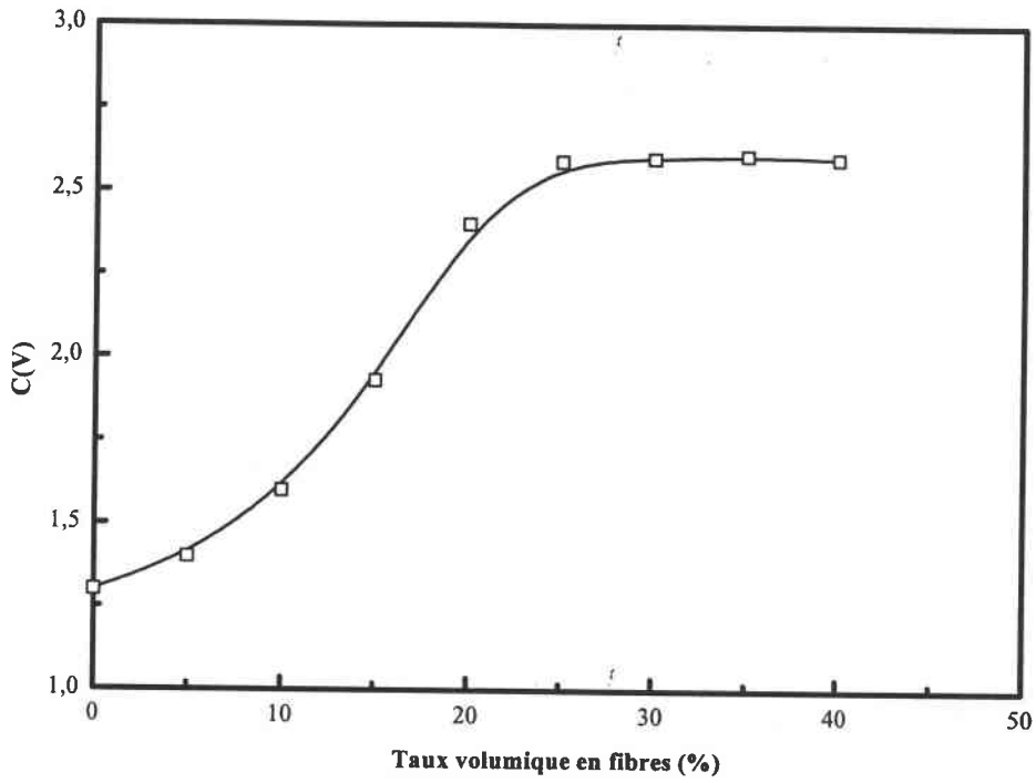
Figure V.C.9 : Evolution de C(V) en fonction du taux de fibres
