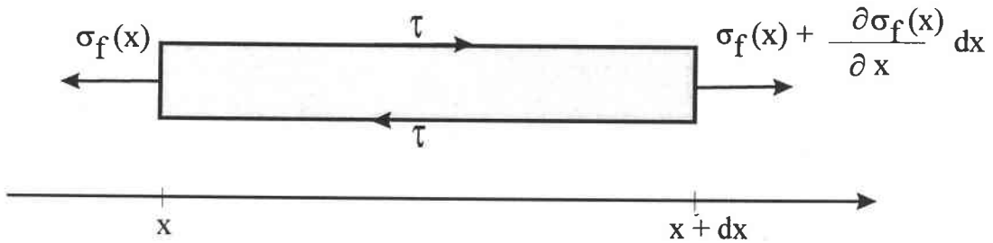
Figure IV.A.9 : Tronçon de fibre de longueur dx
