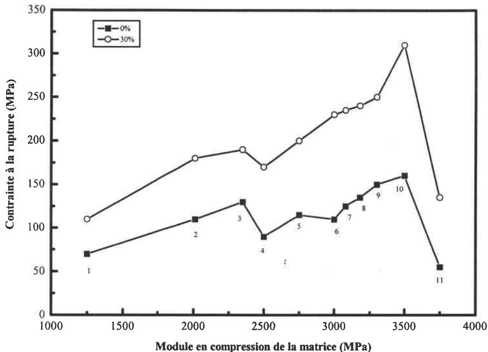
Figure IV.B.27 : Influence de la matrice sur la contrainte à la rupture en compression du matériau composite (fibres de carbone T300-mld, vitesse d'essai : 1mm/min)
