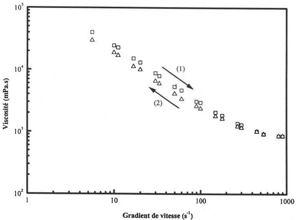
Figure III.B.4 : Mesure de la viscosité à gradient croissant (1) et à gradient décroissant (2) pour un mélange ARC-40/32 chargé à 20 % de fibres de carbone T300-mld. (Cellule cône-plan)
