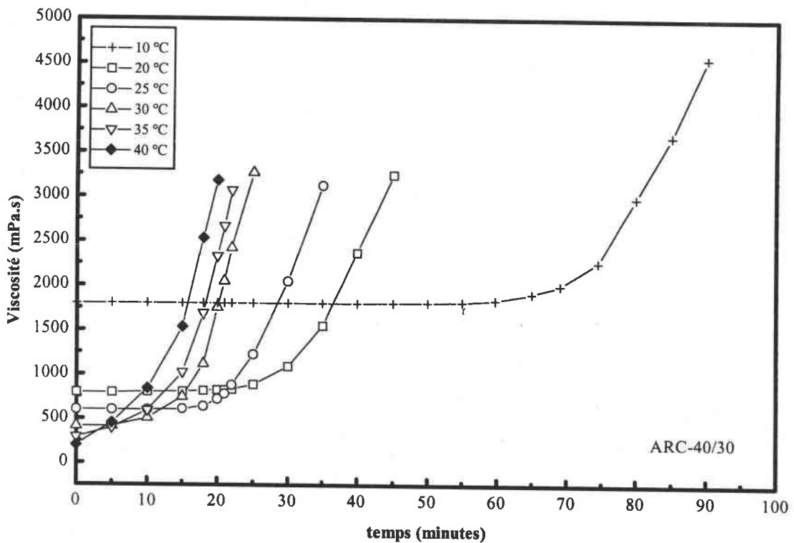
Figure I.A.6 : Influence de la température sur la viscosité de la résine ARC-40/30 pour un gradient de vitesse de 100 \text{ s}^{-1} .
