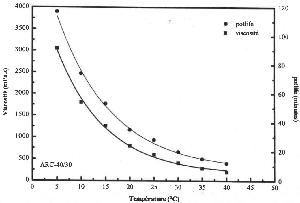
Figure I.A.8 : Variation du temps de gélification en fonction de la température ( \dot{\gamma} = 100 \text{ s}^{-1} )
