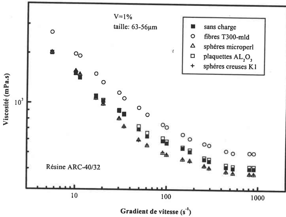
Figure III.C.12 : Influence du rapport de forme des particules sur la viscosité (résine ARC-40/32, taux volumique de 1%) (cellule cône-plan)
