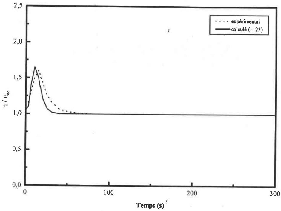
Figure V.B.2 : Modélisation du pic de viscosité dans le cas d'un composite chargé à 15%. (résine ARC-40/32, fibres T300-mld, \dot{\gamma} = 20 \text{ s}^{-1} )
