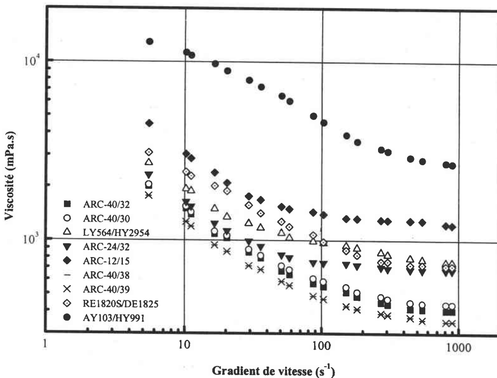
Figure I.A.2 : Viscosités des résines époxydes en fonction du gradient de vitesse (Essais en cellule cône-plan)
