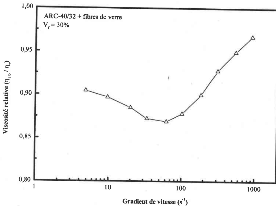
Figure III.C.17 : Evolution de la viscosité relative lors de l'ajout d'un faible taux de microbilles (1%) dans la résine ARC-40/32 chargée avec 30% de fibres de verre (cellule de Couette S1/S)
