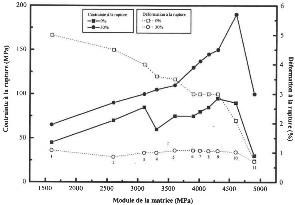
Figure IV.B.25 : Influence de la matrice sur la contrainte à la rupture en traction du matériau composite (fibres de carbone T300-mld, vitesse d'essai : 1mm/min)
