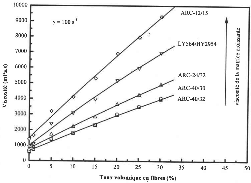
Figure III.B.17 : Viscosité mélange du composite en fonction du taux volumique en fibres de carbone T300-mlld pour différentes matrices époxydes. (gradient de vitesse de 100 \text{ s}^{-1} , cellule cône-plan)
