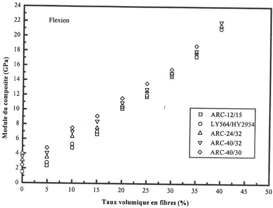
Figure IV.B.14 : Evolution du module élastique en flexion en fonction du taux de charges en fibres de carbone T300-mld (vitesse d'essai : 1mm/min)
