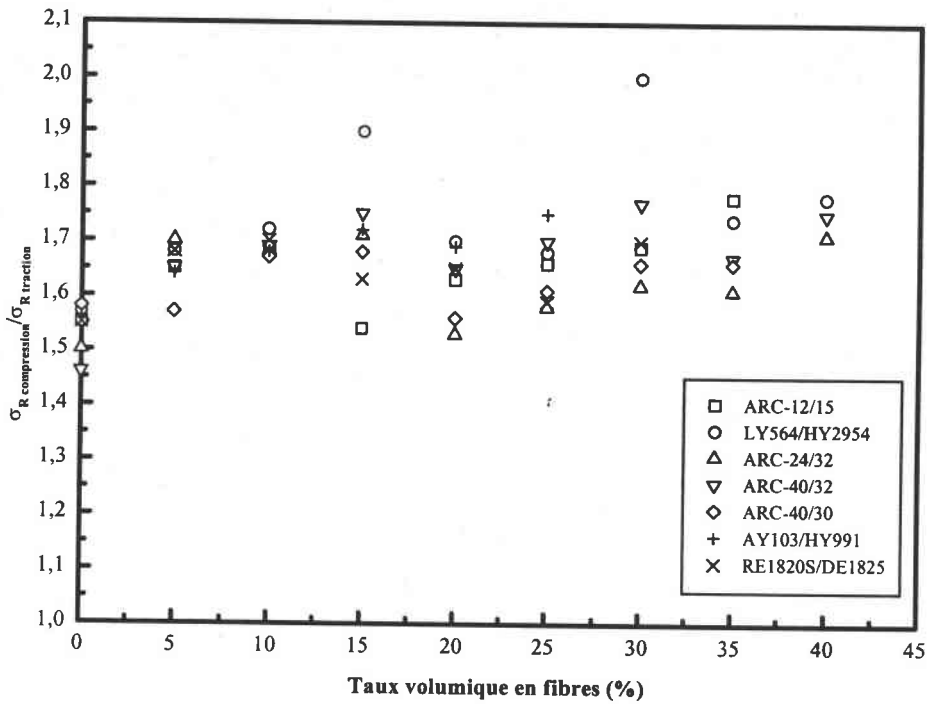
Figure V.C.5 : Rapport des contraintes à la rupture en traction et en flexion
