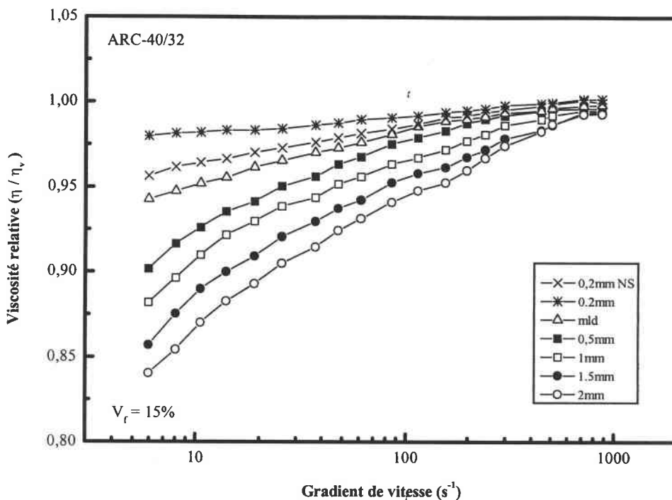
Figure III.C.6 : Evolution de la viscosité relative en fonction de la longueur des fibres de carbone T300 (cellule de Couette S1/S, résine ARC-40/32, V_f = 15\% )
