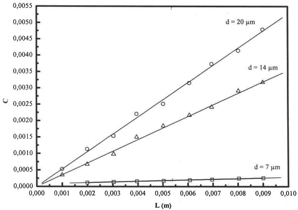
Figure V.A.3 : Evolution du coefficient de frottement en fonction de la longueur des fibres dans la paraffine (0,162 Pa.s)
