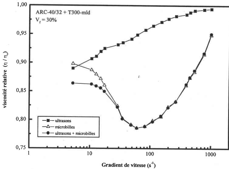
Figure III.C.18 : Influence du traitement sur la viscosité relative d'un mélange composite à base de la résine ARC-40/32 chargée à 30% en fibres de carbone T300-ml (cellule de Couette S1/S)
