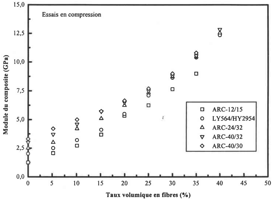
Figure IV.B.16 : Evolution du module élastique en compression en fonction du taux de charges en fibres de carbone T300-mld (vitesse d'essai : 1mm/min)
