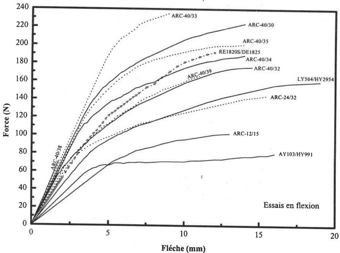
Figure I.A.4 : Courbes (Force / Flèche) en essais de flexion
