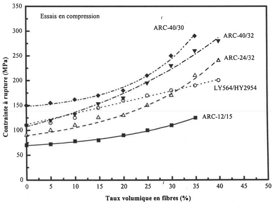
Figure IV.B.17 : Evolution de la contrainte à la rupture en compression en fonction du taux de charges en fibres de carbone T300-mld (vitesse d'essai : 1mm/min)
