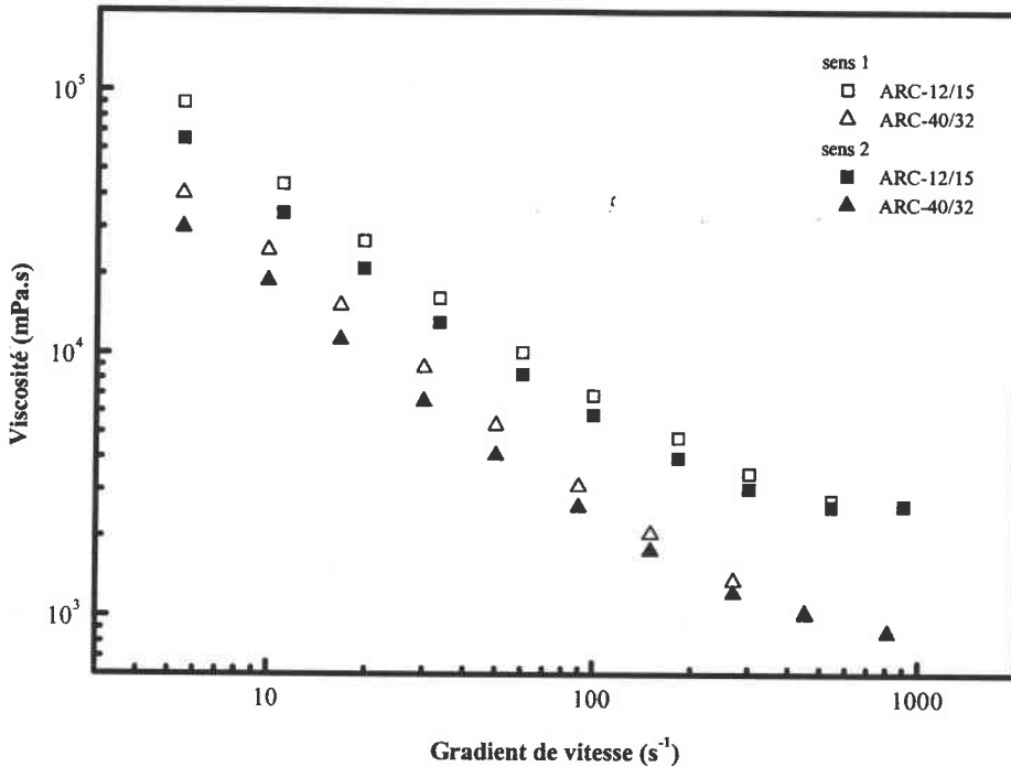
Figure III.B.20 : Mesure de la viscosité à gradient croissant (1) et à gradient décroissant (2) pour un mélange ARC-12/15 chargé à 20 % de fibres de carbone T300-ml et un mélange ARC-40/32 chargé à 20% de fibres de carbone T300-ml. (cellule de Couette S1/S)
