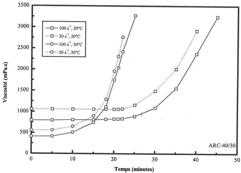
Figure I.A.7 : Influence du gradient de vitesse sur le temps de gélification de la résine ARC-40/30 à la température de 20°C (□) et 30°C (○).
