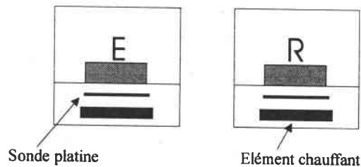
Figure II.B.1 : Tête de mesure d'un appareil de DSC
