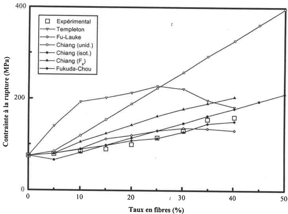
Figure V.C.7 : Comparatif entre les différents modèles et les résultats expérimentaux. (ARC-40/32, fibres T300-ml)
