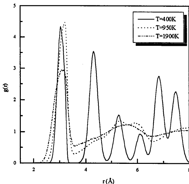
Figure III.11 : La fonction de distribution des paires de AgI (rocksalt) à p = 20 \text{ kbar} .
