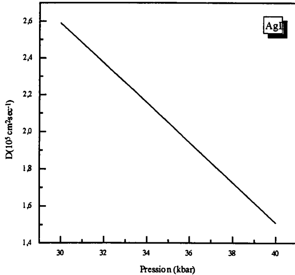
Figure III.10 : Le coefficient de diffusion de AgI (rocksalt) en fonction de la pression à T = 1200 \text{ K} .
