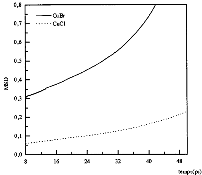
Figure III.3 : Le déplacement quadratique moyen des \text{Cu}^+ en fonction du temps pour le \text{CuCl} et le \text{CuBr} .
