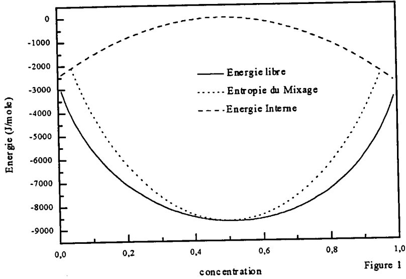
Figure II.1 L'énergie libre du C_xBN_{1-x} en fonction de la concentration x .
