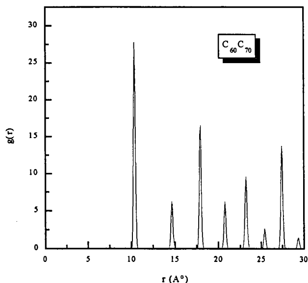
Figure II.2 : La fonction de distribution de paires du C_{60}C_{70} .
