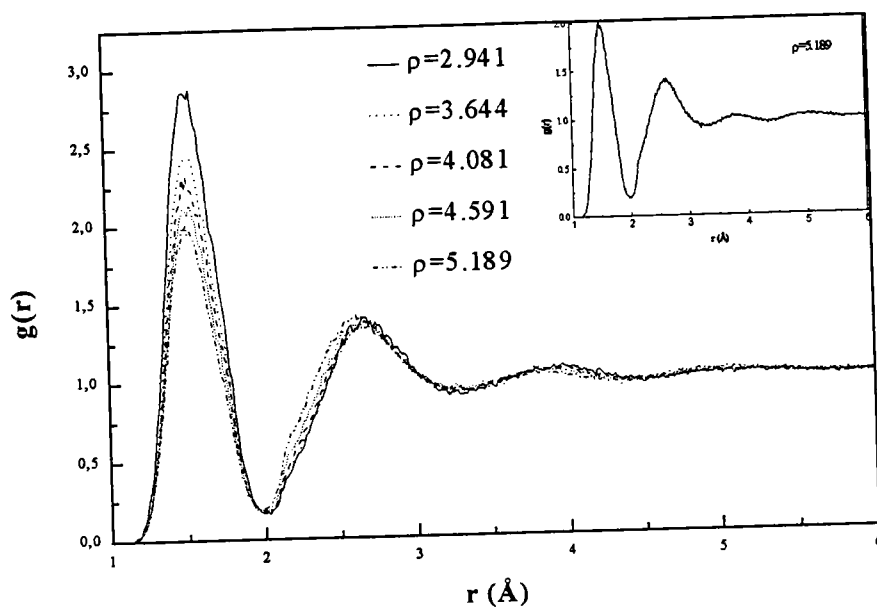
Figure I.5 : La fonction de distribution de paires du BN à l'état liquide pour différentes densités.
