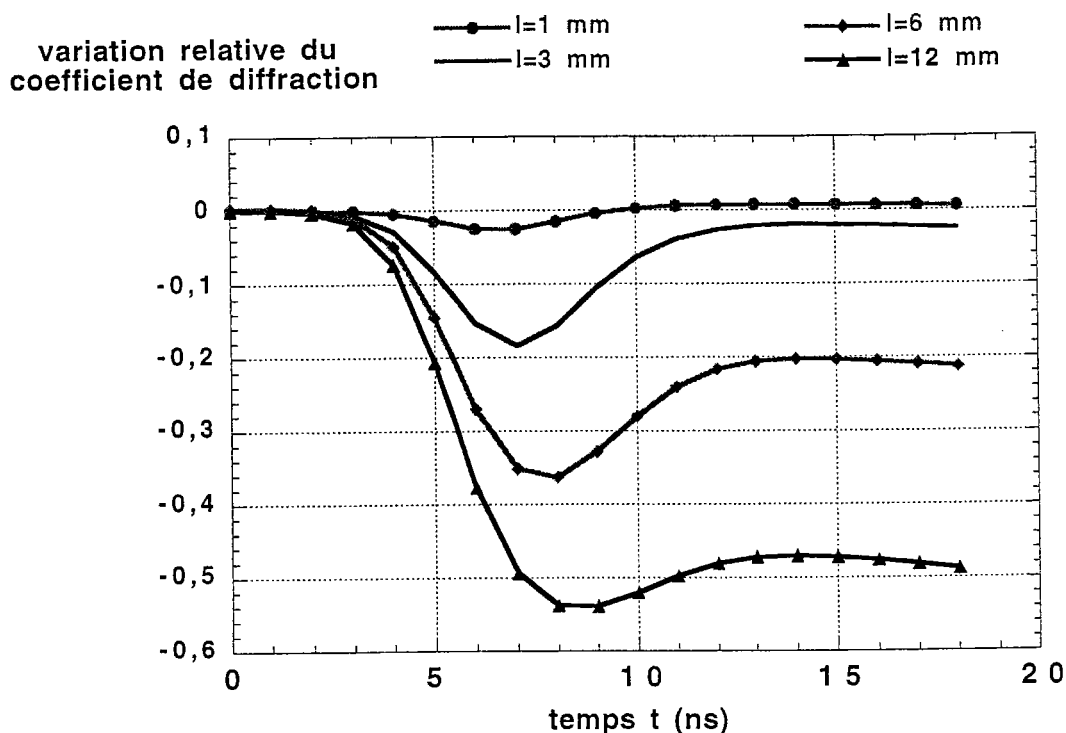
Figure 15 : Dépendance temporelle de la variation relative de \alpha par rapport à \alpha_r pour différentes longueurs l de cristal et une tension appliquée de 2500 V.
