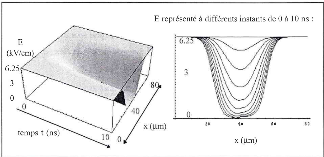
Figure 7 : Construction du champ de charge d'espace en fonction du temps t et de la dimension transversale x dans un cristal de \text{Bi}_{12}\text{SiO}_{20} pour une mobilité plus élevée \mu=3.10^{-4} \text{ m}^2/\text{V.s} : \tau_p = 10 \text{ ns} , à différents instants t=0, 2, 3, 4, 5, 6, 7, 8, 9, 10 \text{ ns} .
