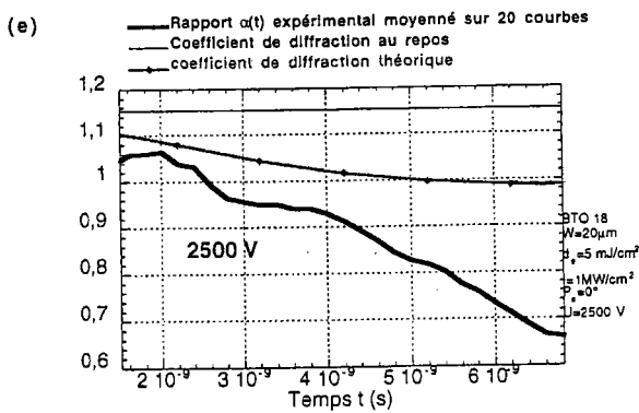
Figure 22 : Evolution temporelle du coefficient de diffraction \alpha(t) expérimental ( P_s=0^\circ ) et théorique ( P_s=-45^\circ ) pour w_e=20\ \mu\text{m} , I_0=1\ \text{MW}/\text{cm}^2 pour différentes tensions appliquées (a) 500 V (b) 1000 V (c) 1500 V (d) 2000 V (e) 2500 V
