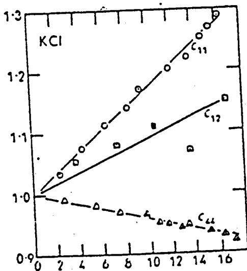
figure (V.2): effet de la pression sur les constantes élastiques de : Al,Cu,CuZn,KCl,NaCl [2] \eta défini par: V / V_0 = (1+2\eta)^{3/2} V :volume sous pression et V_0 :Volume initial C' : constantes élastiques sous pression C :constantes élastiques initiales.
