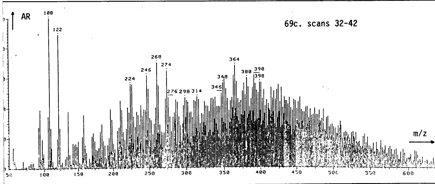
Figure 69. Analyse par Py-FIMS. Spectres de masse fractionnés de l'extrait NMP de la fusinite du GC : F-GC-E : AR = f(m/z) 69a. zone 1; 69b. zone 1'; 69c. zone 2
