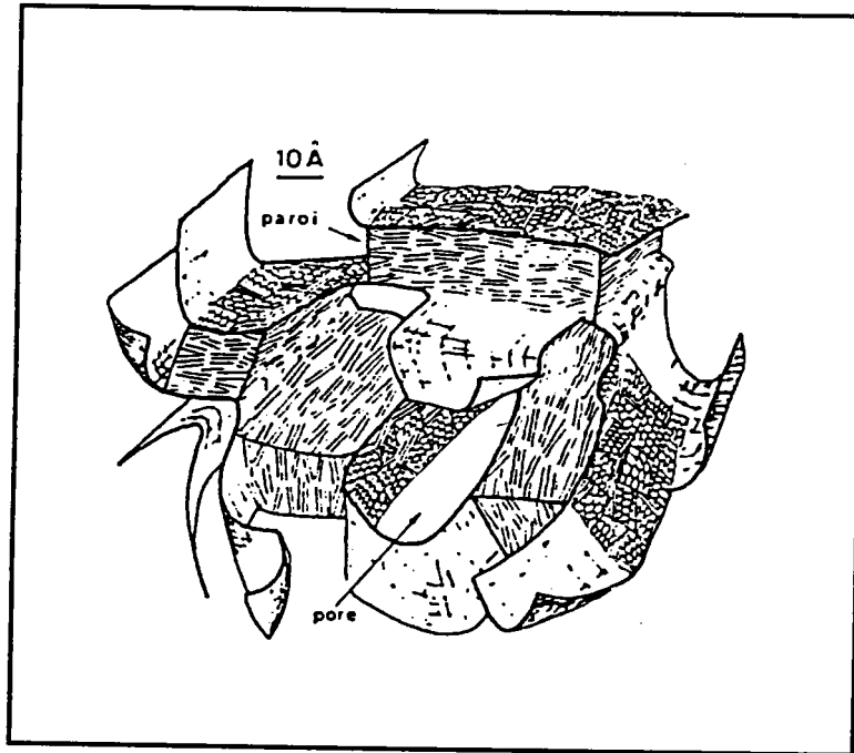
Figure 81. Modèle de la microtexture d'une matière carbonée après l'apparition d'une orientation moléculaire locale (14).
