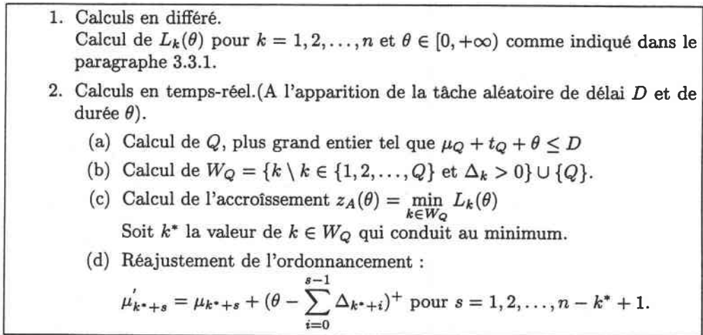
FIG. 3.8 – Algorithme général
