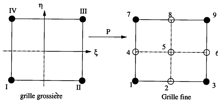
FIG. B.1: Construction de l'opérateur de prolongement P dans le cas ou N = 2
