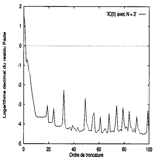
(b) Préconditionneur Incomplet de Cholesky pour N = 3
