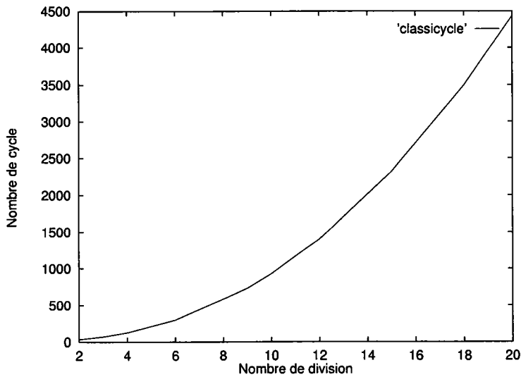
FIG. 2.13: Evolution du nombre de cycles de la méthode à 2-grilles classique en fonction du nombre de division N , lisseur de Jacobi, \omega = 0.8 , résolution itérative
