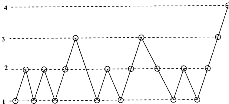
FIG. 1.12: V-cycle d'initialisation
