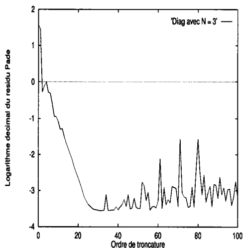
(b) Préconditionneur diagonal pour N = 3
