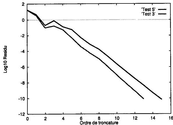
FIG. 3.1: Logarithme décimal du vecteur résidu (Padé) en fonction de l'ordre I pour les tests 3 et 5
