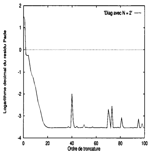
(a) Préconditionneur diagonal pour N = 2
