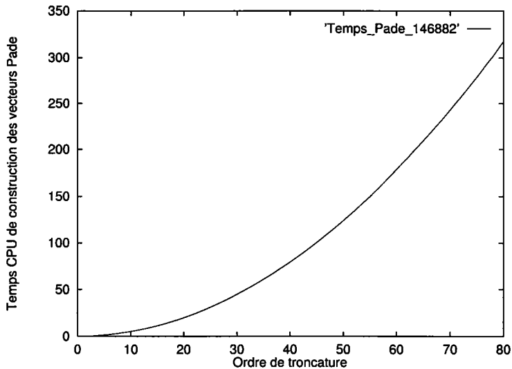
FIG. 2.11: Evolution du temps CPU en secondes de construction des vecteurs Padé en fonction de l'ordre de troncature de l'algorithme à 2-grilles ( N=3 , grille grossière : 16562 d.d.l, grille fine : 146882 d.d.l, convergence obtenue à l'ordre 63)
