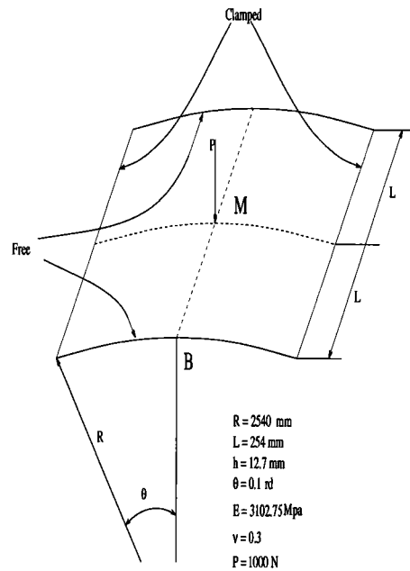
FIG. 1.1: Toit : description géométrique
