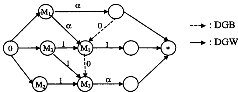
Figure 3.8 : Contre-exemple
