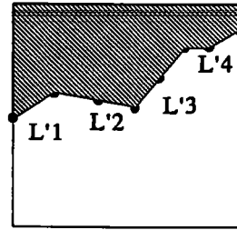
espace paramétrique associé à F_j
