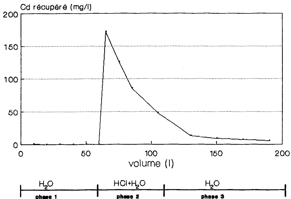
figure 5.6 : suivi de la concentration de cadmium en sortie de colonne (essai de désorption par lavages acides).
