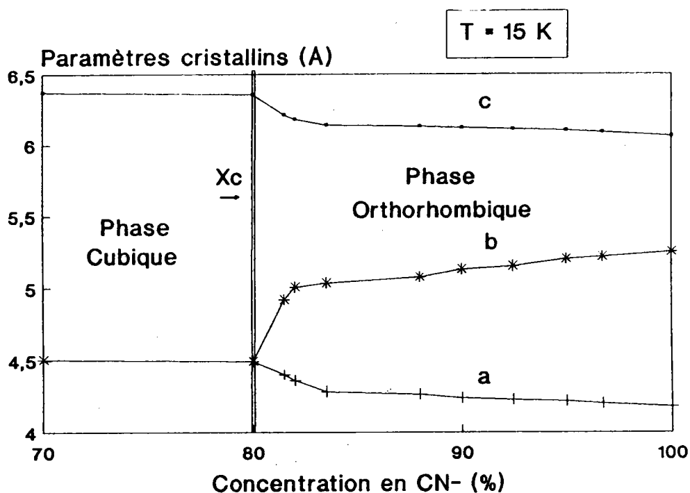
Figure 1.25 : Evolution avec la concentration des paramètres de la phase orthorhombique à 15 K pour le système mixte (KCN)_x(KCl)_{1-x} .
