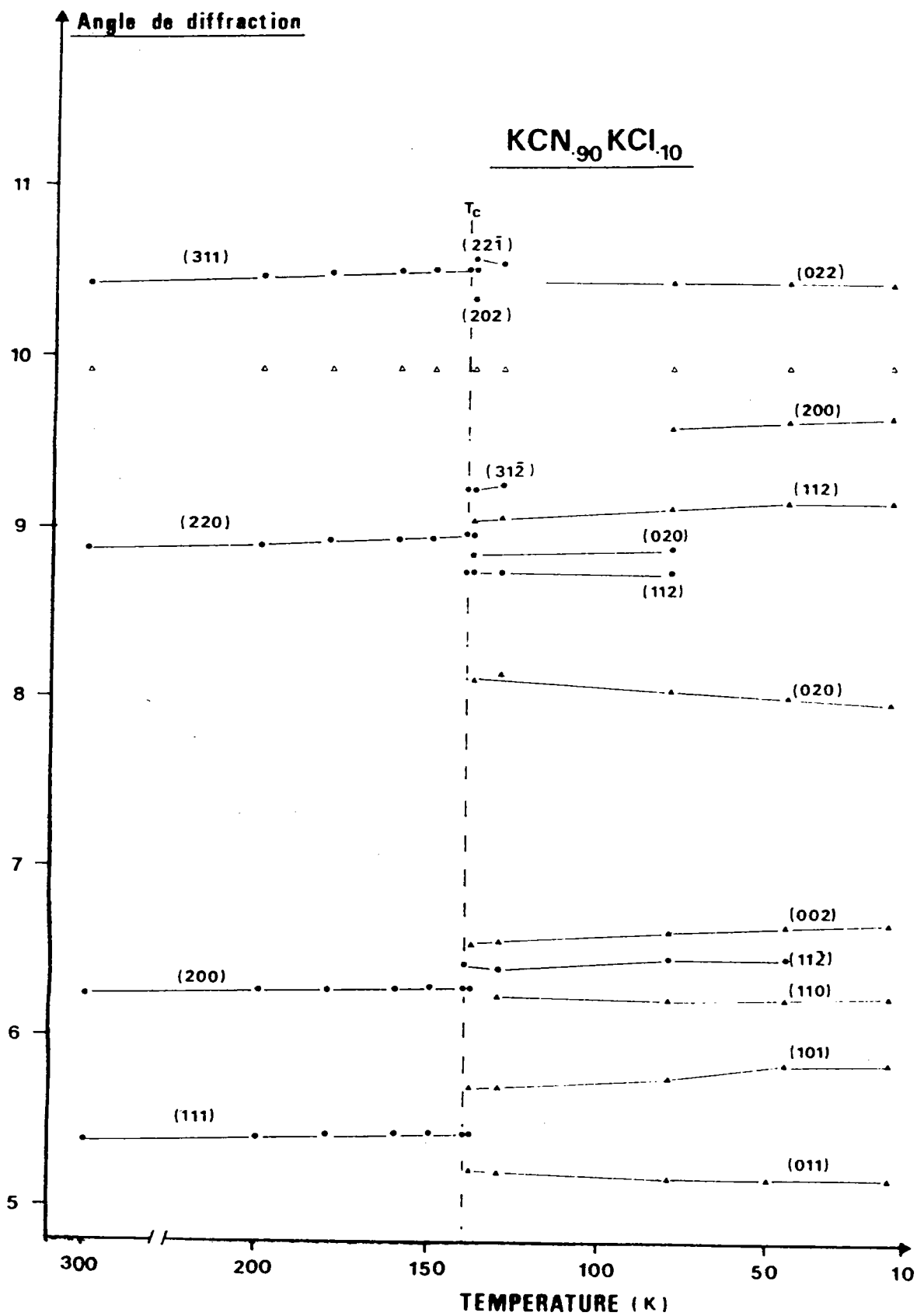
Figure 1.22: Evolution des raies (hkl) de diffraction de (\text{KCN})_{0.90}(\text{KBr})_{0.10} en fonction de la température (• raies cubiques, * raies monocliniques, ▲ raies orthorhombiques et Δ position de la raie de référence du diamant).
