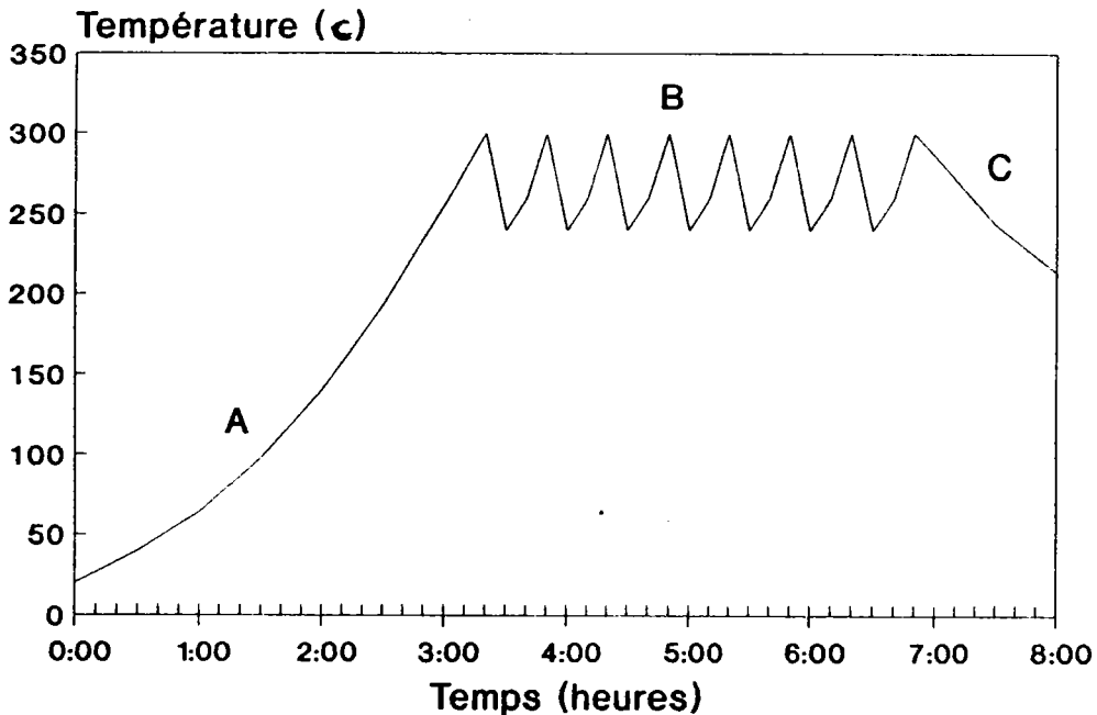
Figure 1.19: Forme du traitement thermique choisi pour réduire les contraintes résiduelles dues au broyage en poudre.
