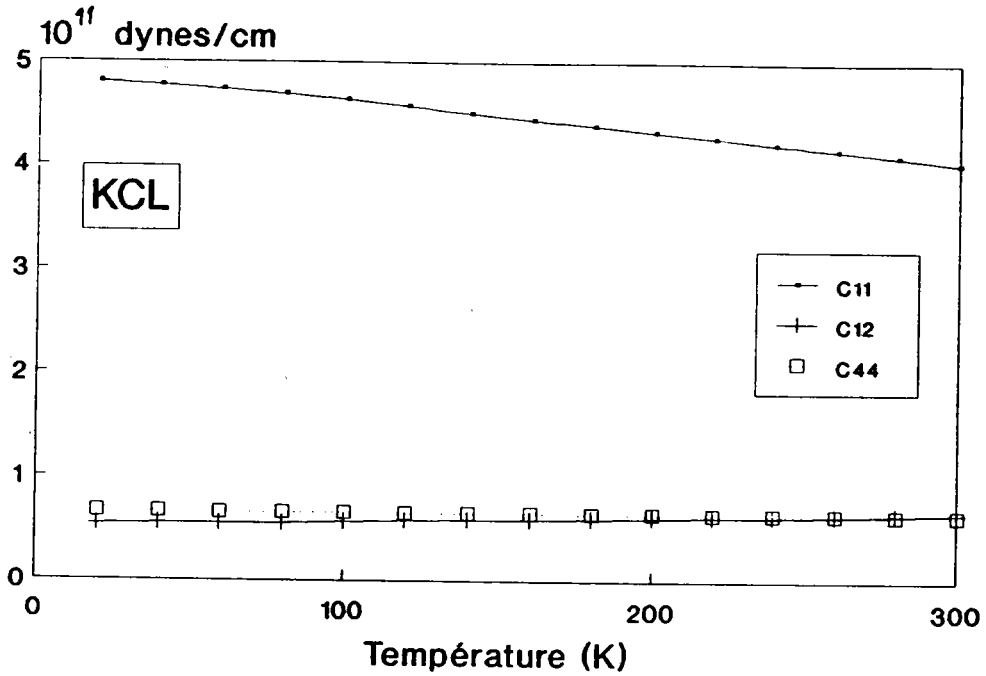
Figure 2.5 : Evolution avec la température des constantes élastiques de KCl (Norwood 1958)
