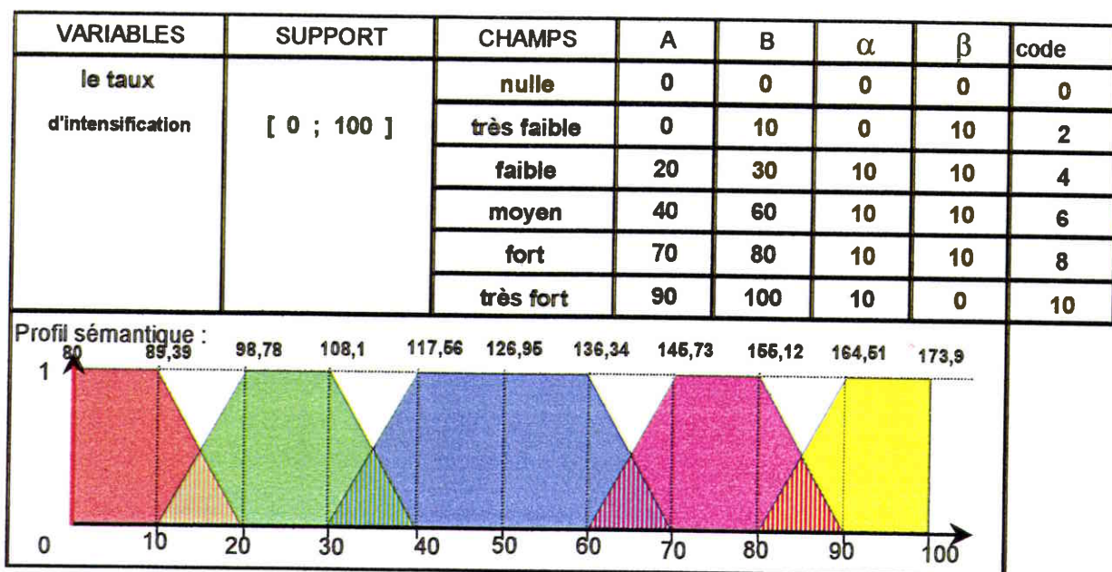
Figure 33 : Profil sémantique
