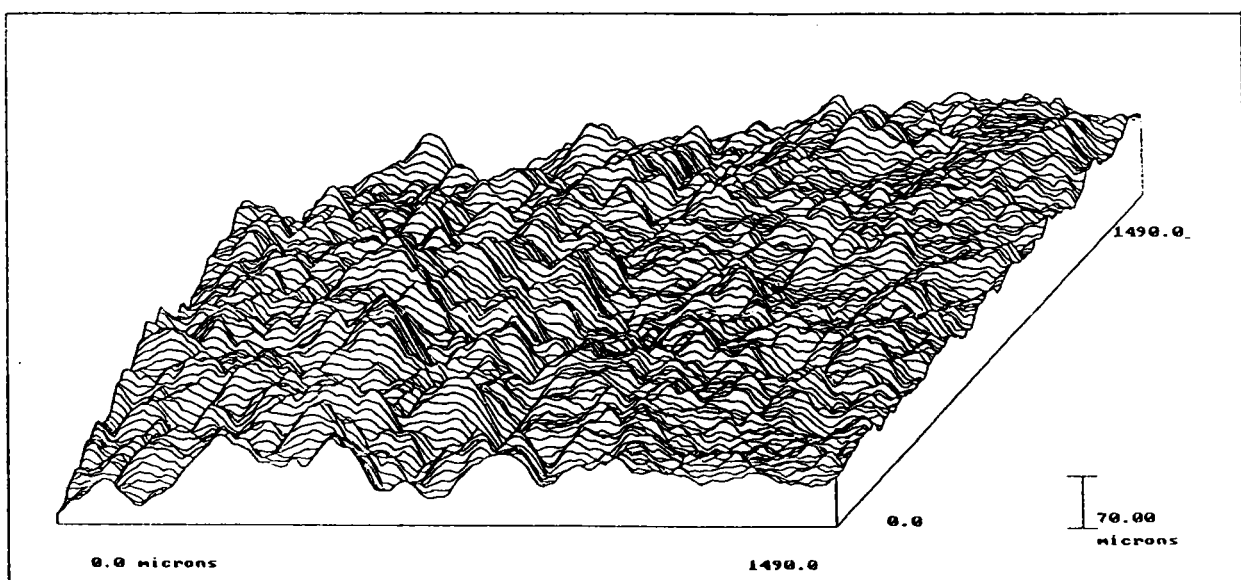
FIGURE 38 : Visualisation 3-D d'un faciès de l'alliage 7949 (N°33) effectué à BESANCON.
