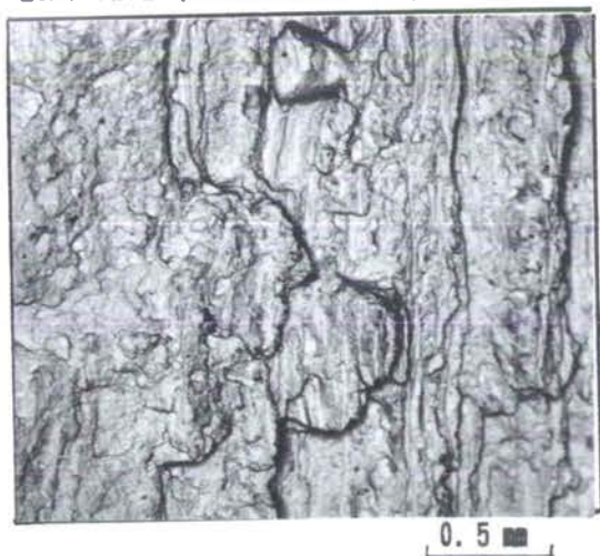
FIGURE 34 : Faciès de rupture de l'acier XC 35 traité (essai dynamique) observés au microscope électronique à balayage ; élect. rétrodiffusés (gauche), élect. secondaires (droite).
