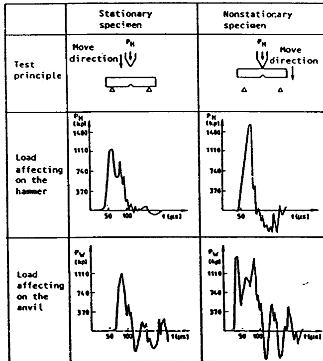
FIGURE N°A1-4a : Diagrammes force - temps mesurés pour un acier mi-dur testé à -60^{\circ}\text{C} [5] pour des éprouvettes normales :
