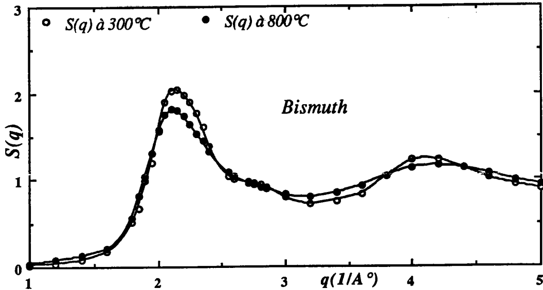
Figure 10 : Facteur de structure du bismuth calculé à partir du modèle de sphères dures.
