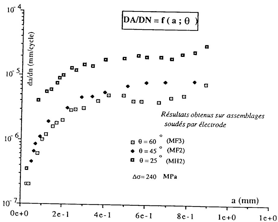
Evolution de la vitesse de propagation des microfissures de fatigue en zone I du cordon Influence de l'angle de raccordement \theta sur la vitesse de fissuration figure (46 b)
