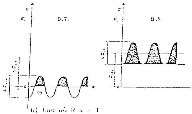
figure (5) : Effet de R et de contraintes résiduelles de traction \sigma_{res}
