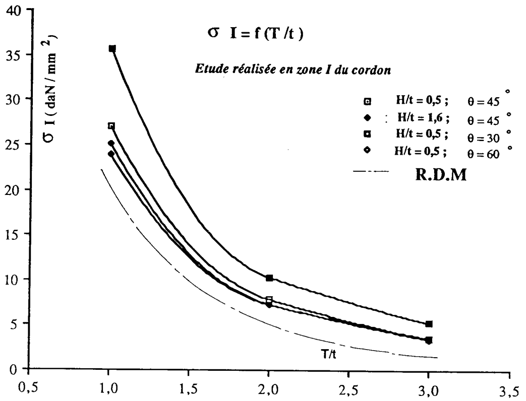
Evolution de \sigma_I en fonction du rapport d'épaisseurs T/t ( Etude effectuée en zone I du cordon )
