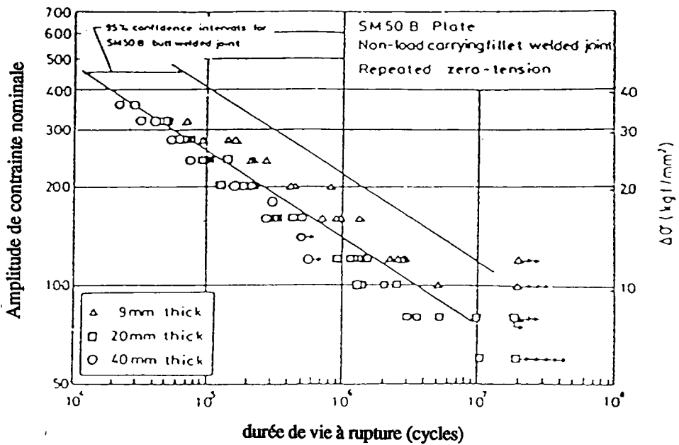
figure (7) : Influence de l'épaisseur de la tôle sur la durée de vie
