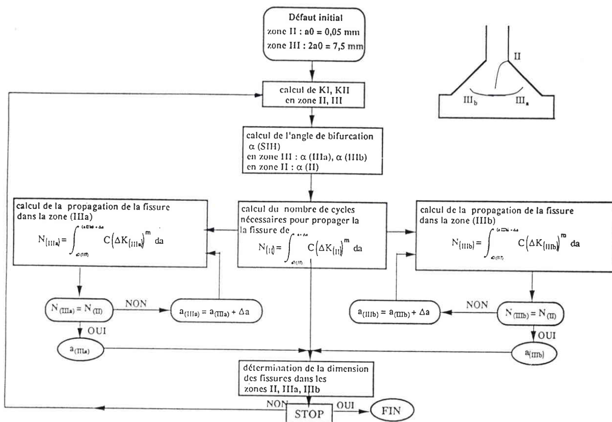
figure (5 a) Algorithme appliqué pour simuler le chemin de fissuration lorsque le mode de ruine de l'assemblage en angle est multiple (fissures de fatigue présentes en pied et en racine de la soudure)
