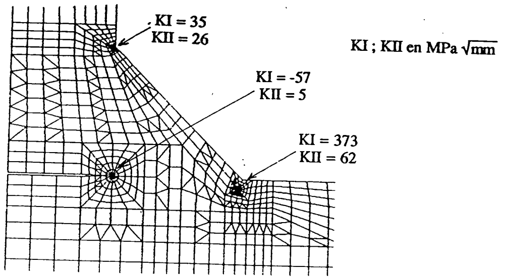
Amorçage prévu en zone I du cordon
