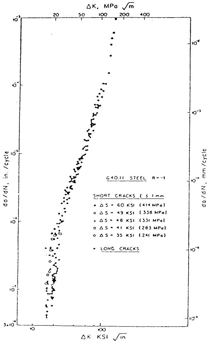
figure (35) : Vitesse de propagation de la fissure en fonction de \Delta K en tenant compte du paramètre l_0
