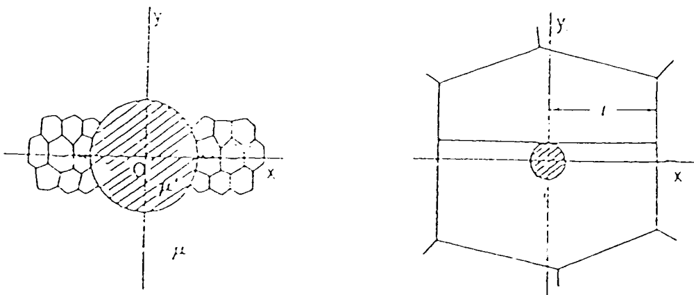
figure (11) : Contrôle de la fissure courte par la plasticité de l'entaille
