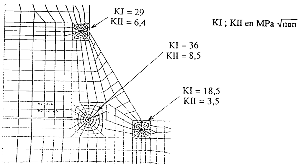
Amorçage prévu en zone III du cordon
