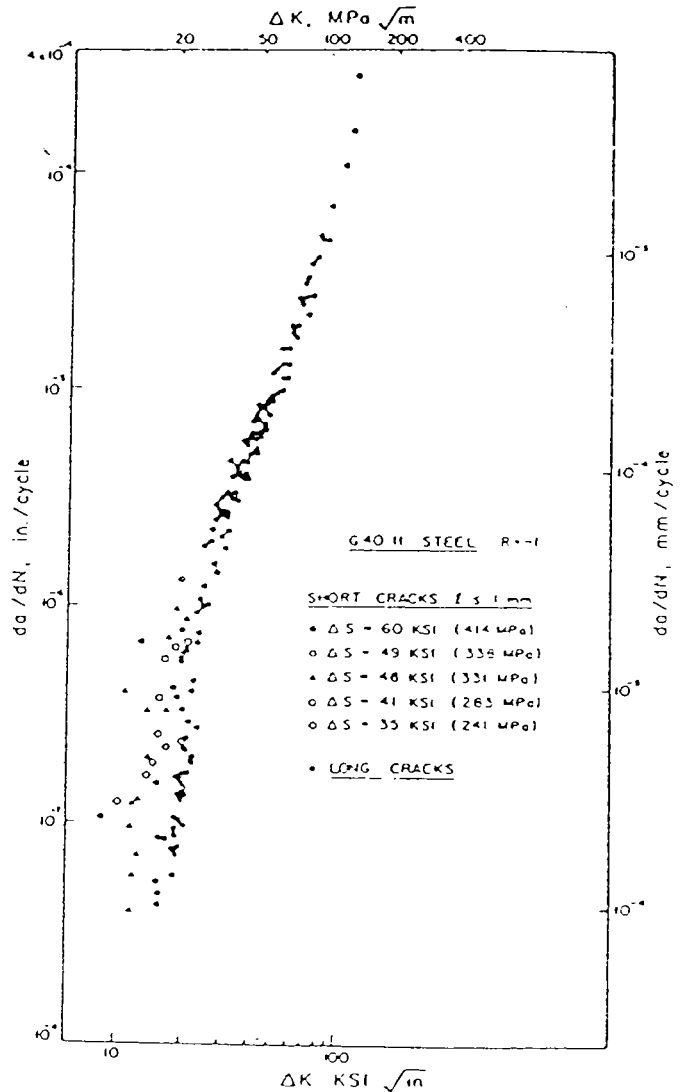
figure (36) : Comparaison des vitesses de propagation des fissures courtes et fissures longues pour un acier G 40-11 sans tenir compte du paramètre l_0 dans la détermination de \Delta K
