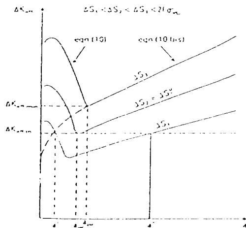
Variation de \Delta K_{eff} en fonction de la longueur de la fissure dans un joint soudé ( \psi = 135^\circ )
