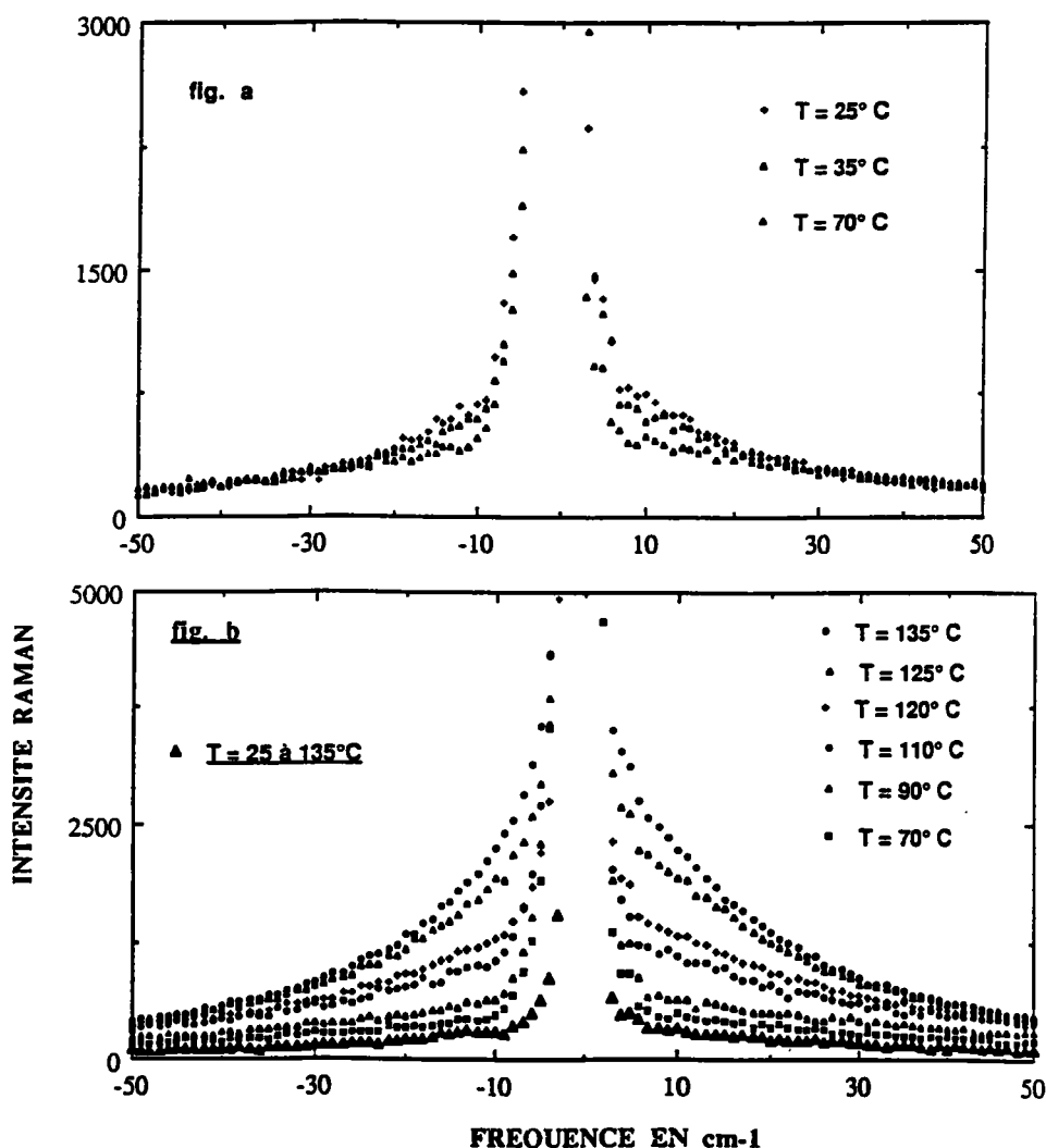
FIGURE 3A-13: Evolution de la composante centrale de la configuration Z(yz)Y pour les températures 25, 35 et 70^\circ\text{C} (fig.a) puis 70 à 135^\circ\text{C} (fig.b) . le spectre le plus bas représenté à titre de comparaison correspond aux configurations Z(xx)Y [et Z(yx)Y ] et reste identique entre 25 et 135^\circ\text{C}
