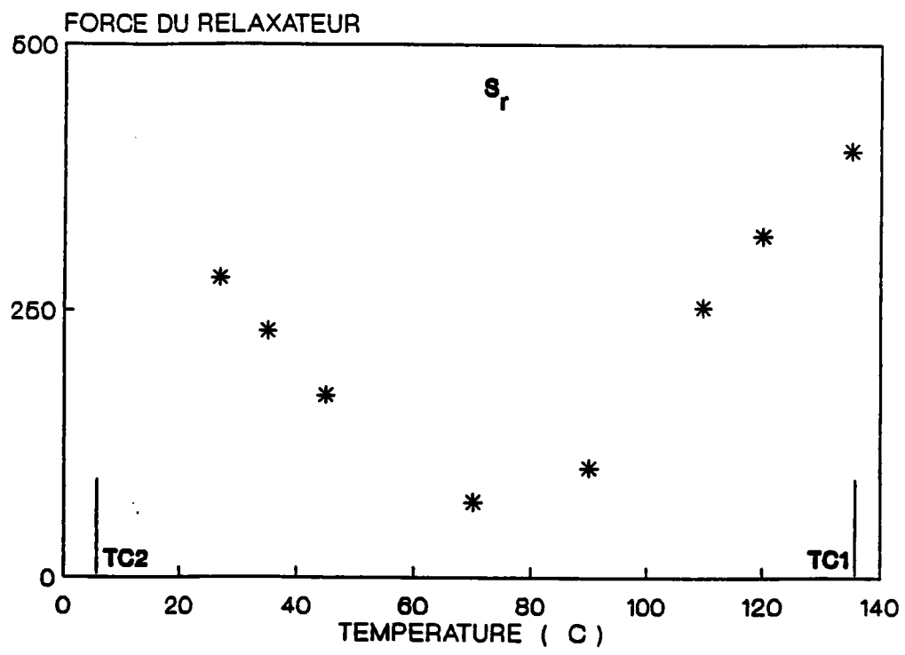
FIGURE 3B-12: dépendance en température de la vitesse de relaxation et de la force du relaxateur déduites de l'ajustement avec le modèle 2.
