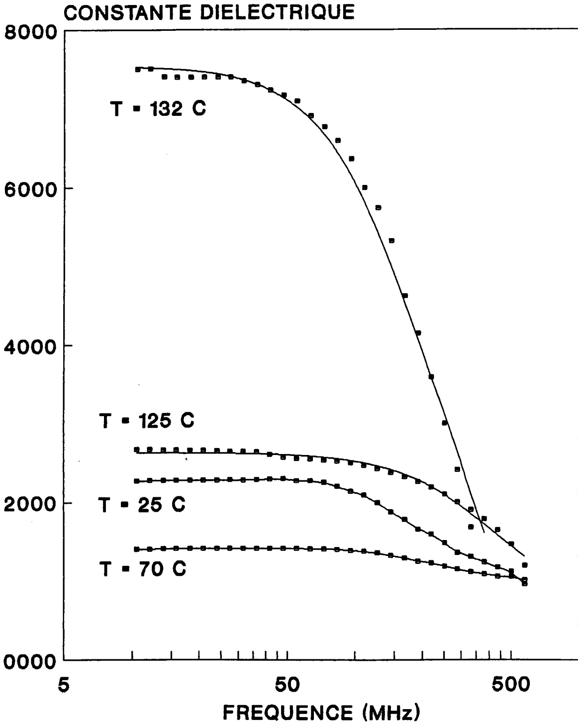
FIGURE 4-3: ajustement de la fonction diélectrique dans la phase quadratique (températures 25, 70, 125 et 135°C) avec le modèle donné par l'équation (4-4)
