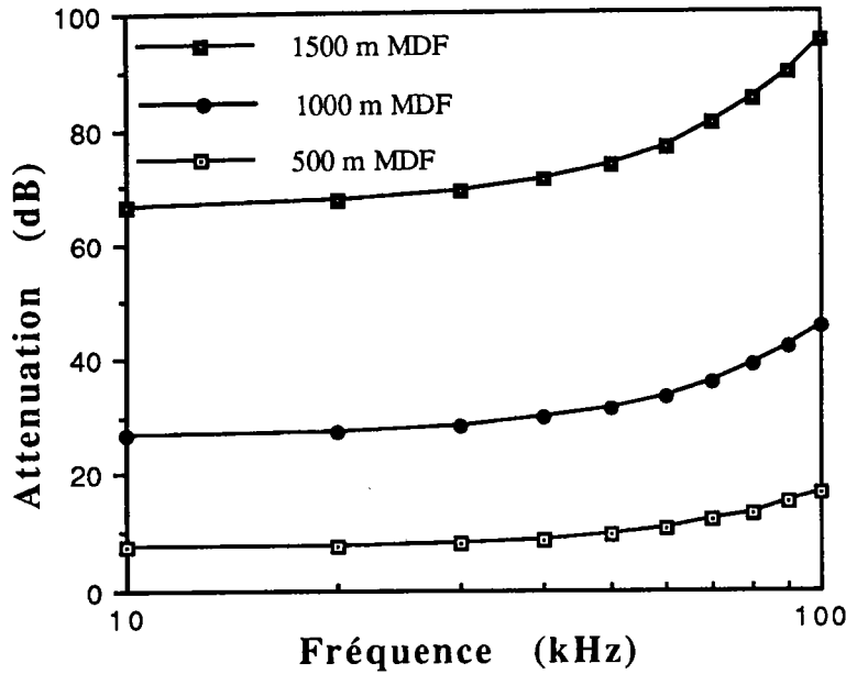
Figure 21: Atten.=f(Fréquence), L=500,1000 et 1500 m, R(z)=a+bz+cz^2 , Gradient non Linéaire.
