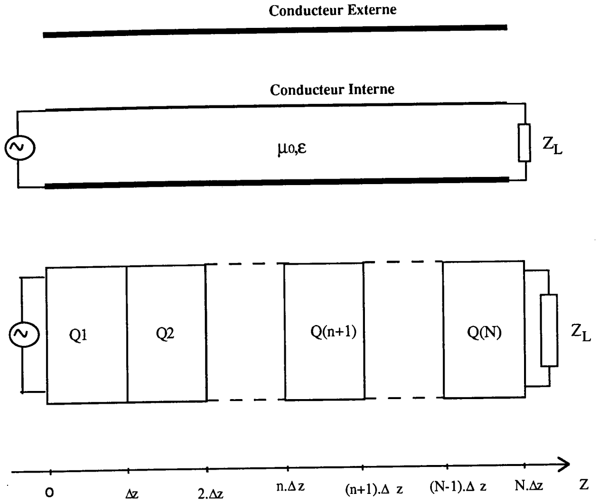
Figure 2: Le Câble Coaxial et son Modèle Equivalent de Quadripôles Elementaires en Cascade Dont les paramètres Varient en Fonction de Z
