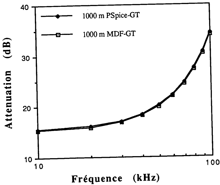
Figure 26: Atten.=f(Fréquence), L=1000 m, en BF avec Gradient de Température
