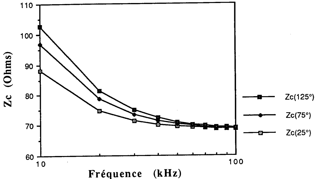
Figure 10 : Impédance Caractéristique=f(Fréq.,Temp.)
