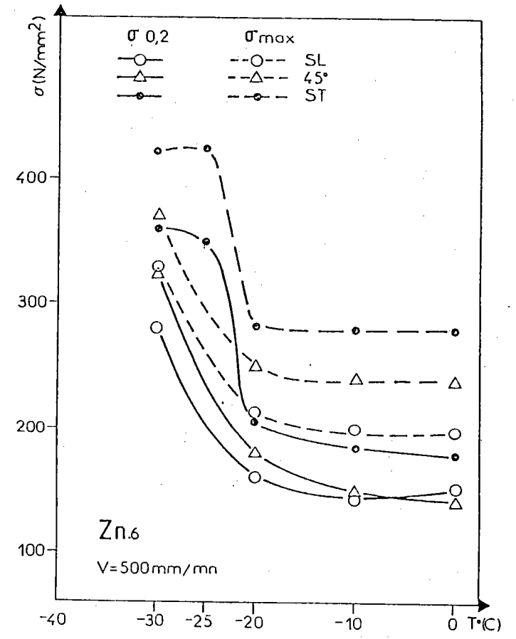
Fig. [V-11B] : Evolution de la charge à la limite élastique et de la charge maximum en fonction de la température.
