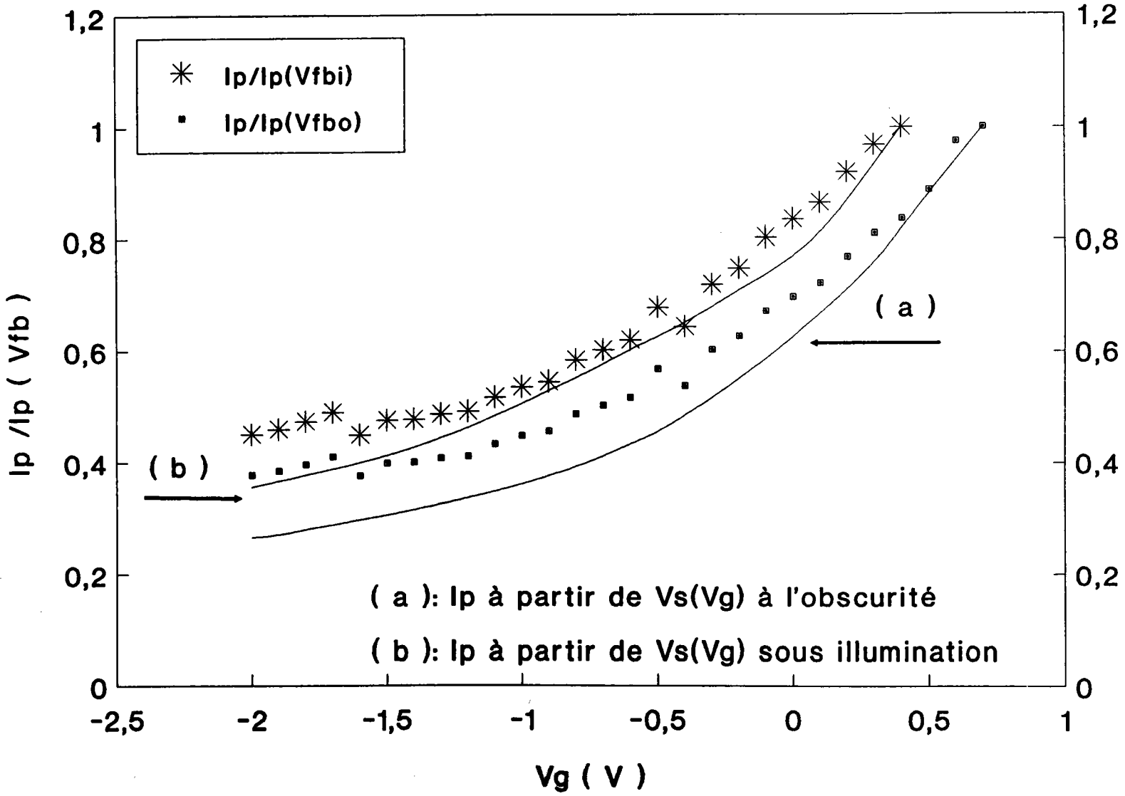
Figure 18: Comparaison de l'intensité de photoluminescence, I_p mesurée et l'intensité I_p calculée à partir de (a): La caractéristique V_s(V_g) à l'obscurité (b): La caractéristique V_s(V_g) sous illumination
