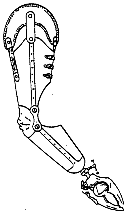
FIGURE 9 Avant-bras de Travail AMAR avec pince universelle - 1917 -
