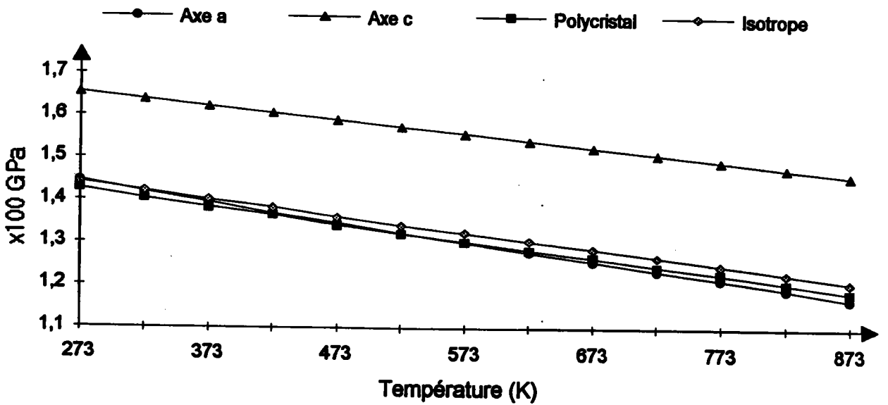
Figure I-37 : C22 en fonction de la température
