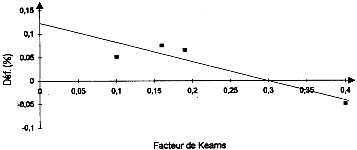
Figure A1-9 : Déformation de polycristaux de zirconium recuits à 5 \times 10^{25} n.m -2 en fonction de leur facteur de Kearns ( T_{irr}=353K )
