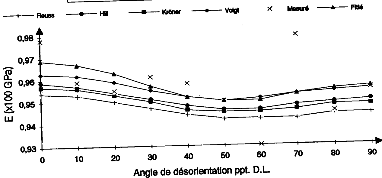
Figure I-15 : Module de Young de Zr11 dans le plan de la tôle
