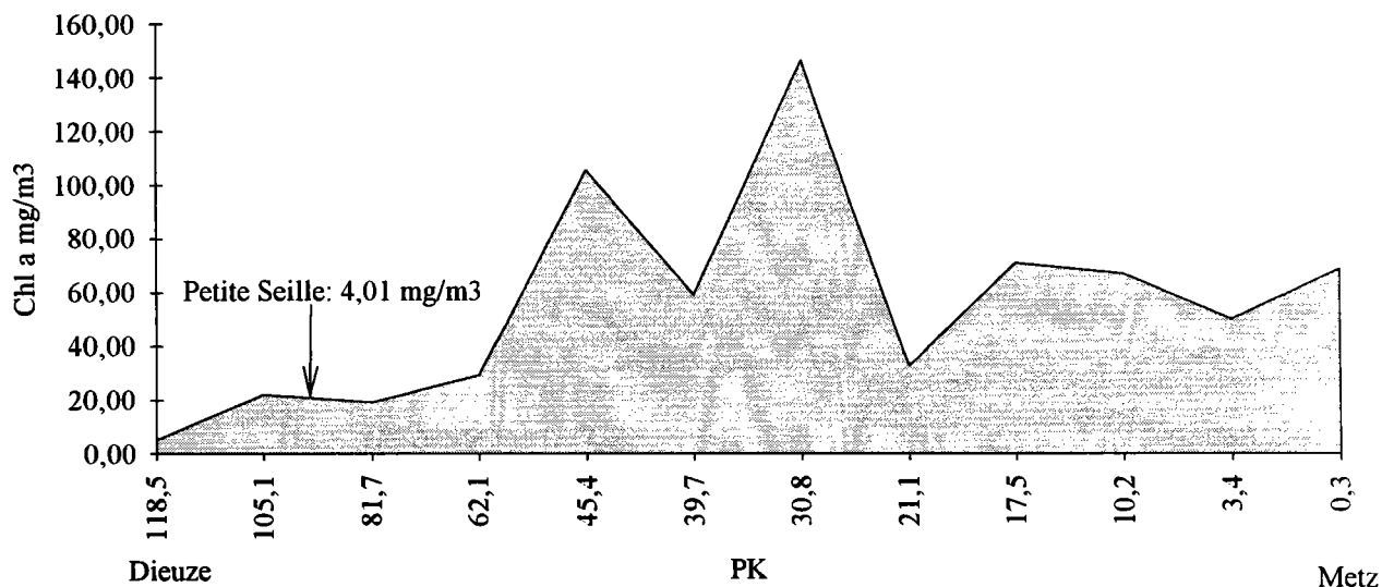
Figure 15: Profil chlorophylle a Seille du 02 août 1987
