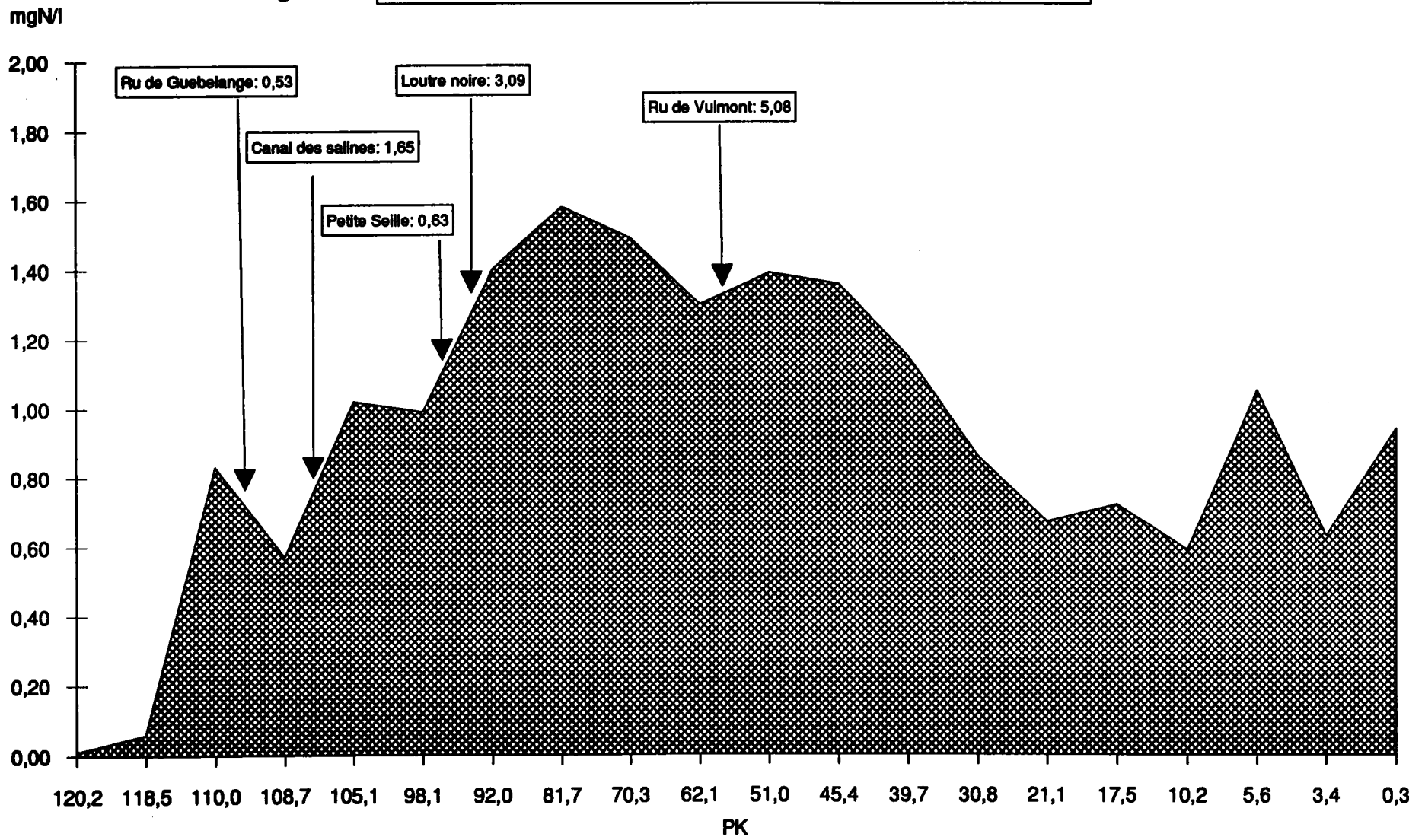
Figure 12 Concentrations minimales de nitrates mesurées au cours des trois profils Seille
