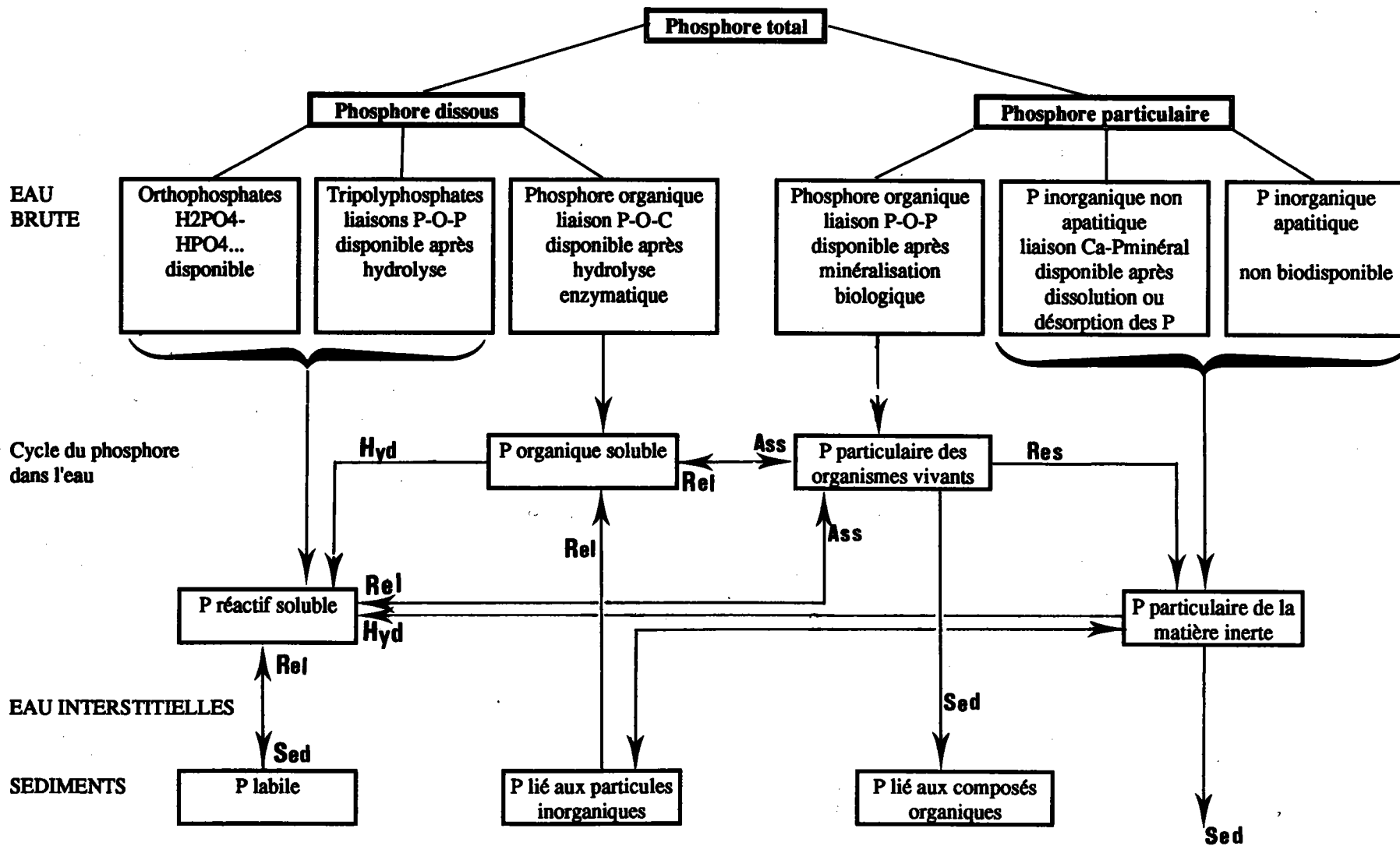
Figure 6 LES DIFFERENTES FORMES DE PHOSPHORE DANS LE MILIEU AQUATIQUE ( extrait du DEA GRASMUCK, 1989)
