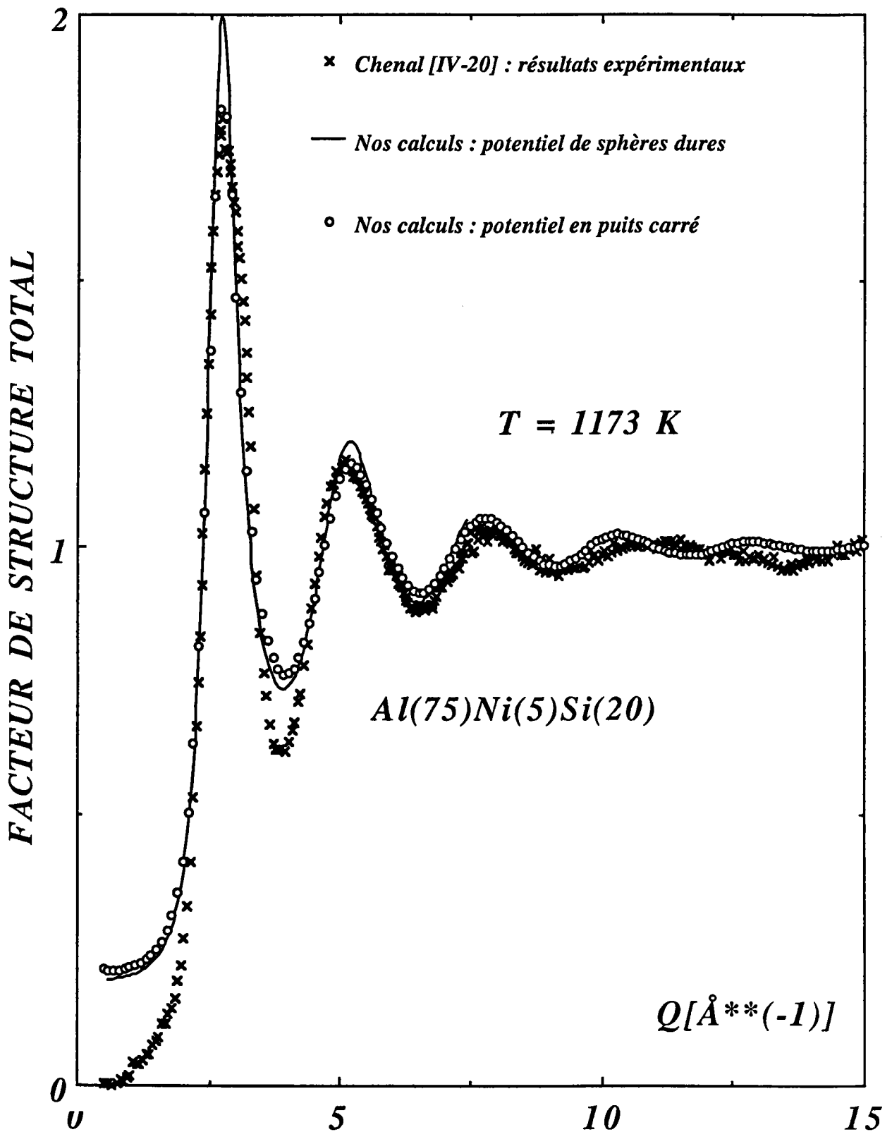
Figure 2 : Facteur de structure total de l'alliage liquide \text{Al}_{75}\text{Ni}_5\text{Si}_{20} à 900^\circ\text{C} .
