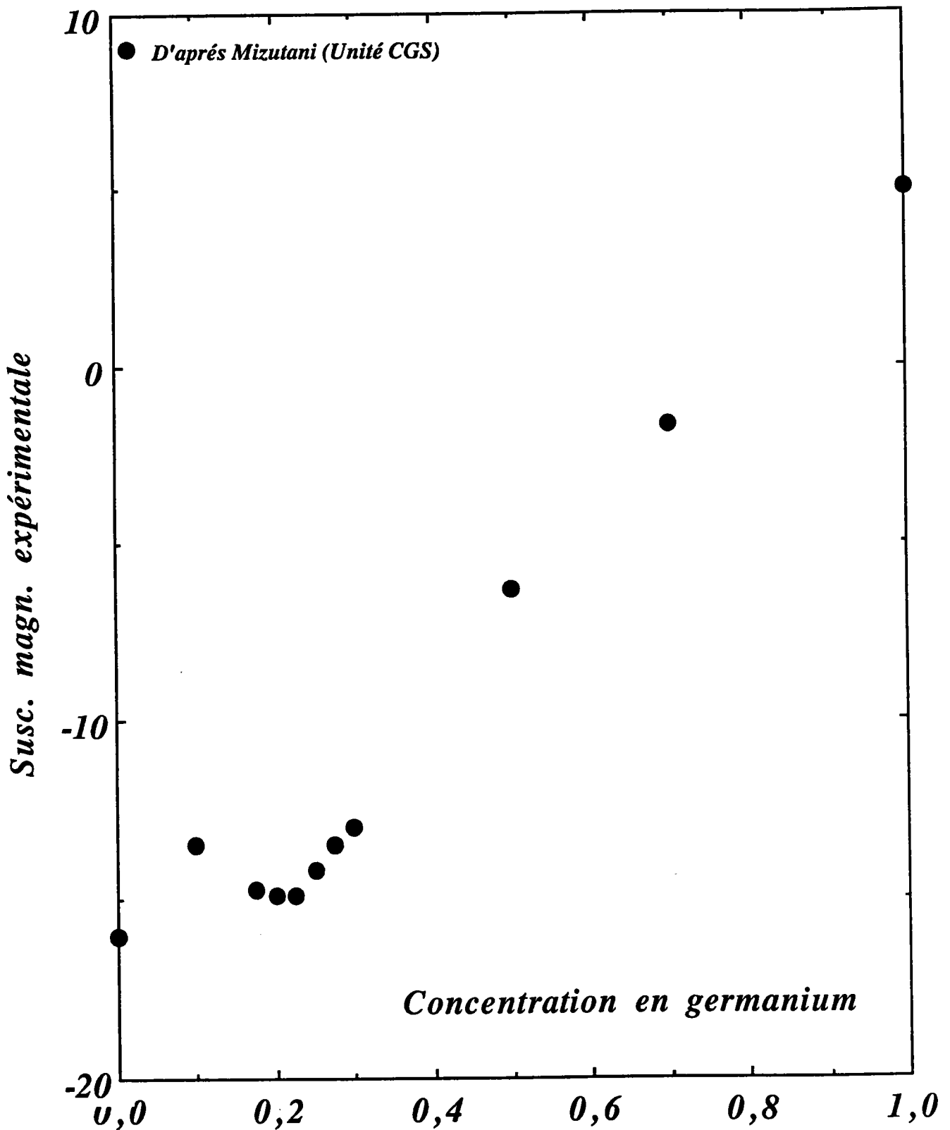
Figure 6 : Susceptibilité magnétique mesurée par Mizutani [V-32] de l'alliage (\text{Cu}_{0,5}\text{Ag}_{0,5})_{1-x}\text{Ge}_x en fonction de la concentration en germanium.
