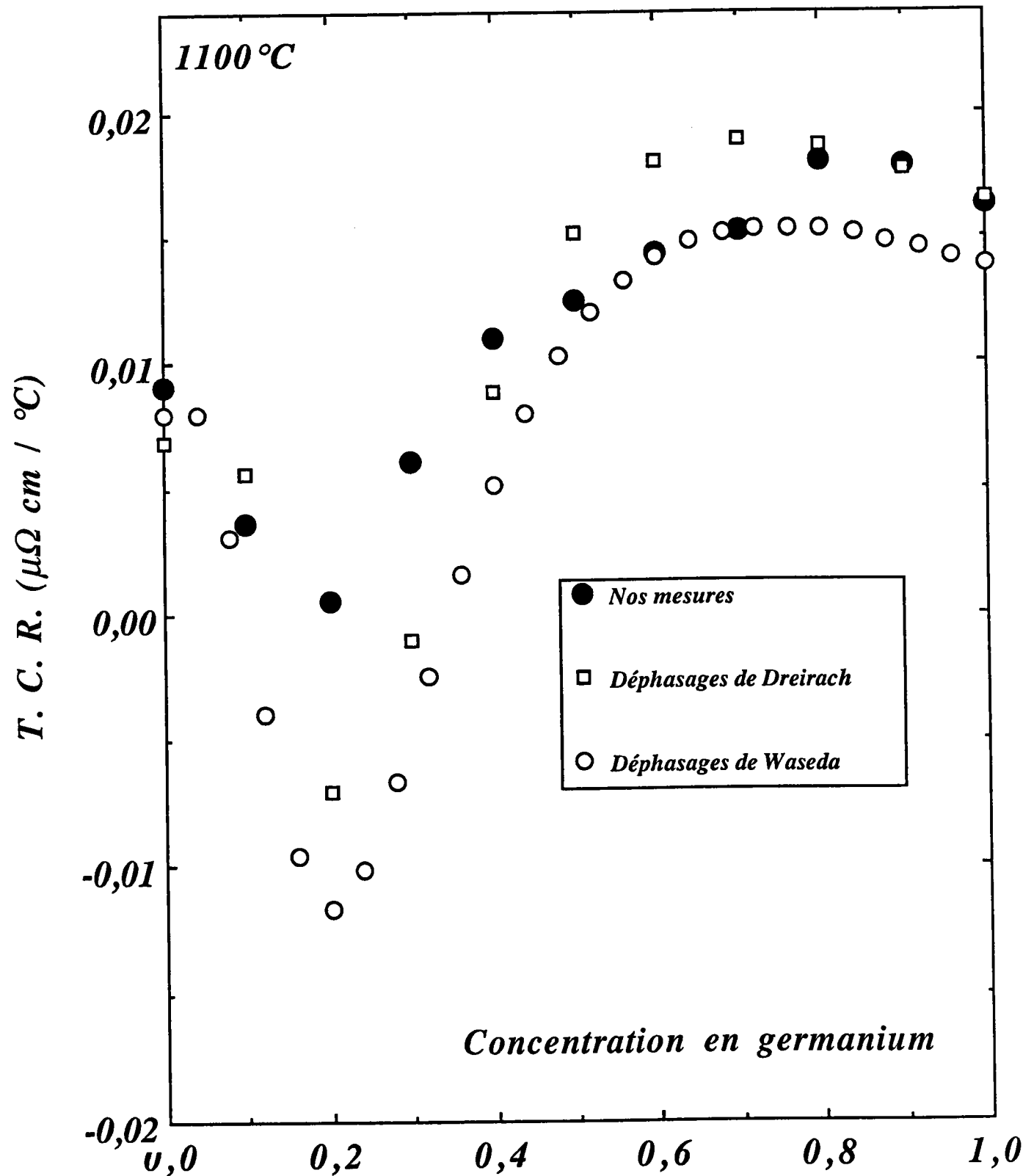
Figure 4 : Coefficient de température de la résistivité électrique de l'alliage (\text{Cu}_{0,5}\text{Ag}_{0,5})_{1-x}\text{Ge}_x en fonction de la concentration en germanium comparé à celui calculé par différents déphasages.
