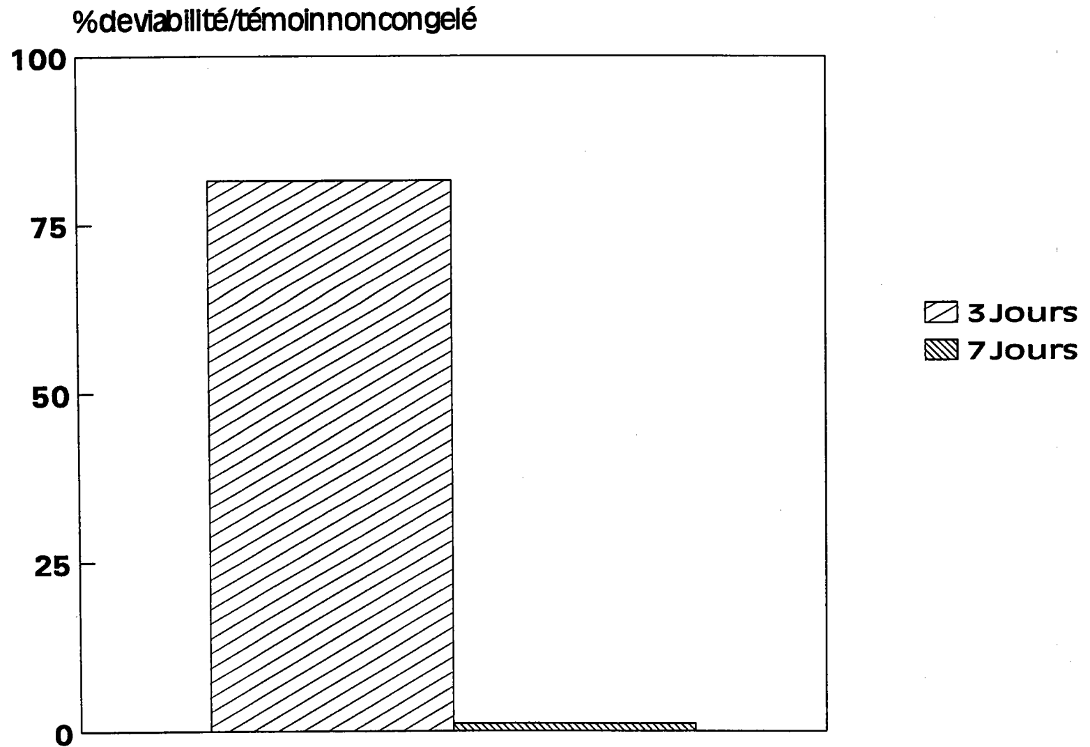
Figure 23 : effets de la congélation à -80°C sur la viabilité de Scenedesmus subspicatus sur milieu solide.
