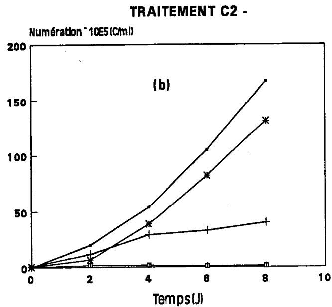
Figure 15 : Effets des traitements de congélation et de cryoprotection sur la viabilité de S. capricornutum .
