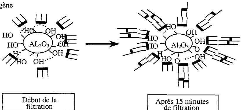
Figure III-20 adsorption des TGs sur une surface d'oxyde d'aluminium. (---- : liaison hydrogène)
