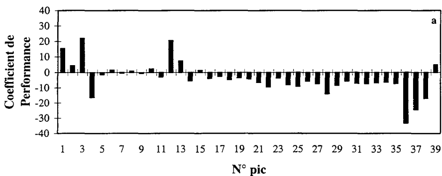
Figure IV-30 Coefficient de performance des TGs sur microbilles de verre (150-212µm) à 60°C a) MGLA adsorbée/ initiale en fonction du N° du pic.
