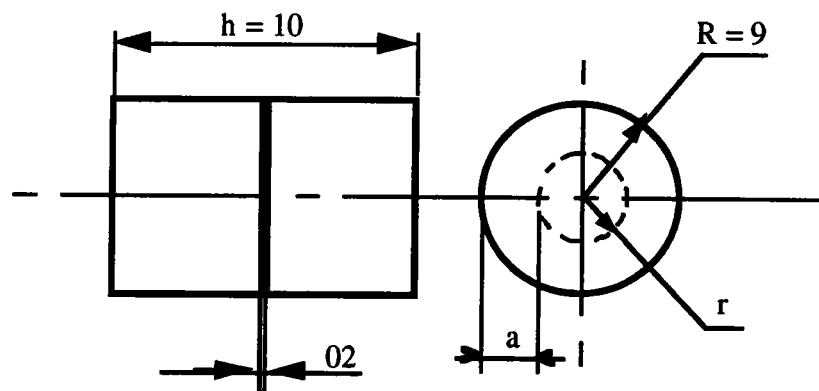
Figure 13.1 : essais dynamiques, géométrie des échantillons.
