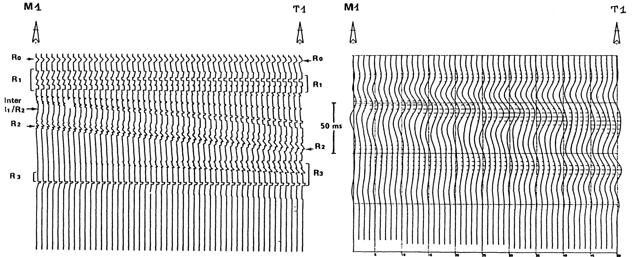
SECTION IMPÉDANCE
