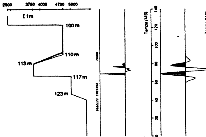
LOG VITESSE
