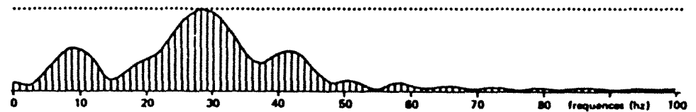
SPECTRE D'AMPLITUDE
