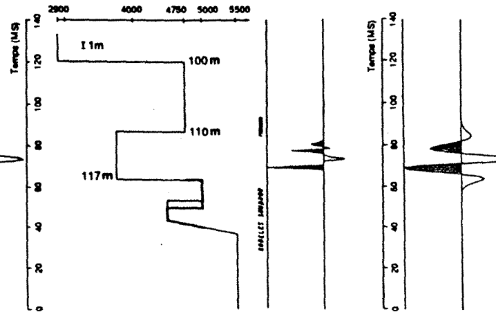
LOG VITESSE
