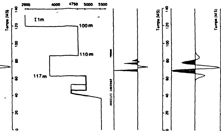
LOG VITESSE
