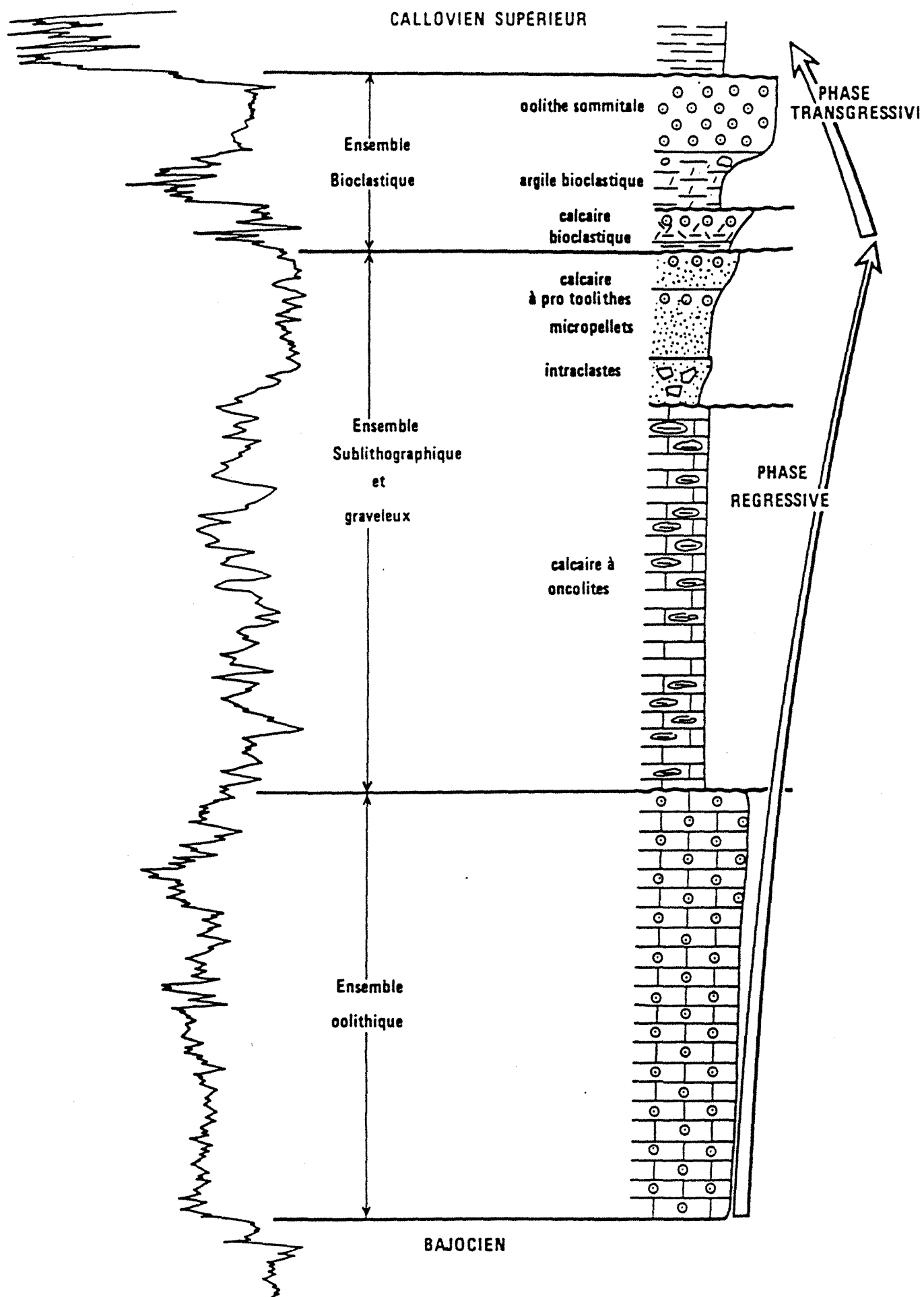
PRINCIPAUX ENSEMBLES DU BATHONIEN ET CALLOVIEN INFERIEUR
