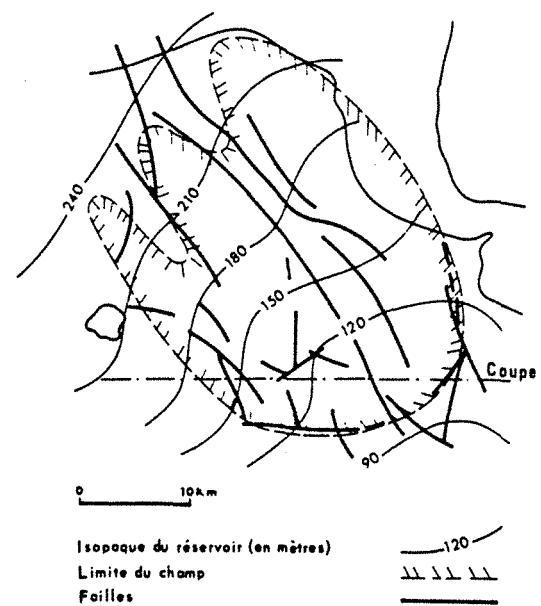
b — Carte et coupe du champ de Groningue, Pays-Bas (d'après STAUBLE & MILIOS, 1970).
