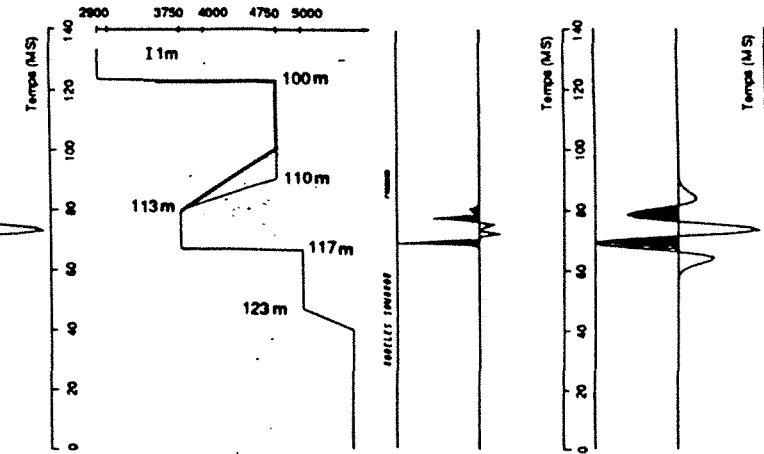
LOG VITESSE
