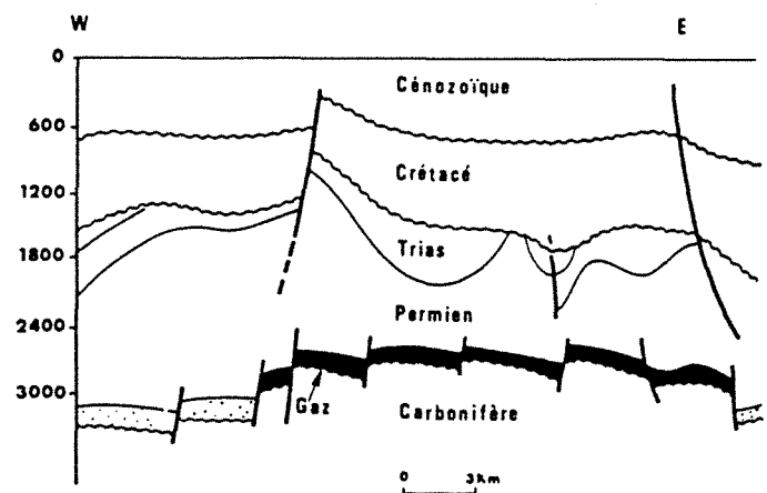
b — Carte et coupe du champ de Groningue, Pays-Bas (d'après STAUBLE & MILIOS, 1970).
