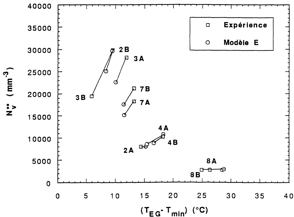
Figure 5.2. Relation entre le nombre de nodules N_V^{**} et la surfusion \Delta T_{EG} de tous les cylindres Ø62. Les petits cercles correspondent aux résultats des calculs faits avec le modèle E. Les résultats expérimentaux sont représentés par les petits carrés. Pour ces calculs, on a utilisé les constantes des lois germination, A_1 et A_{11} , employées dans le cas de la figure 5.1. Les lignes relient les points expérimentaux et ceux calculés qui correspondent à un cylindre.
