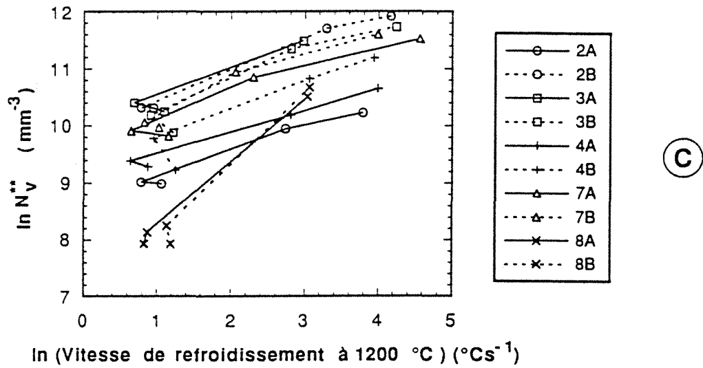
Figure 3.15 Relation entre le logarithme du module géométrique, \ln \text{Mod} , le logarithme de la vitesse de refroidissement à 1000\text{ }^{\circ}\text{C} , \ln V_{1000}^* , et le logarithme de la vitesse de refroidissement à 1200\text{ }^{\circ}\text{C} , \ln V_{1200}^* , avec le logarithme de la densité volumique des nodules de graphites, \ln N_v^{**} , des pièces coulées.
