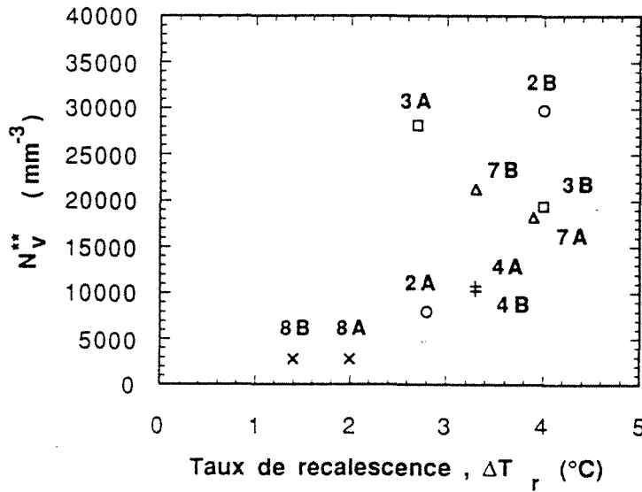
Figure 3.35 Relation entre le taux de recalescence, \Delta T_r et la densité volumique des nodules, N_V^{**} . Les données correspondent aux cylindres Ø62.
