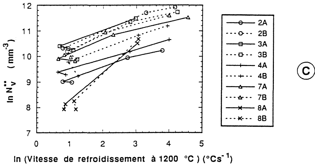
Figure 3.15 Relation entre le logarithme du module géométrique, \ln \text{Mod} , le logarithme de la vitesse de refroidissement à 1000 °C, \ln V_c , et le logarithme de la vitesse de refroidissement à 1200 °C, \ln V_c^* , avec le logarithme de la densité volumique des nodules de graphites, \ln N_v^{**} , des pièces coulées.
