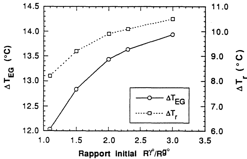
Figure 4.17 Effet de la valeur initiale du rapport R\gamma^\circ/R\theta^\circ de cellules eutectiques sur les valeurs de \Delta T_{EG} et \Delta T_r . Les calculs ont été faits en utilisant le modèle de solidification C avec un coefficient A_1 de la loi de germination égal à 10^{12}\ \text{m}^{-3}\ \text{°C}^{-1} et R\gamma^\circ étant égal à 2,5\ \mu\text{m} .
