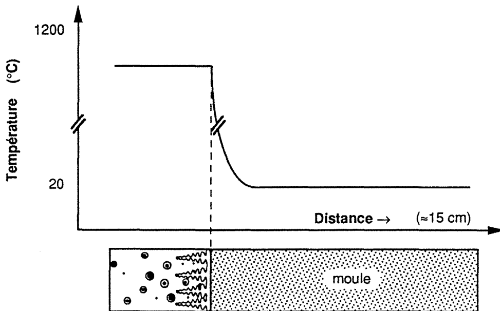
Figure 4.2 Schéma du profil de températures correspondant à un métal dont le refroidissement est contrôlé par le transfert de chaleur à travers le moule. La température du métal est homogène à tout instant.
