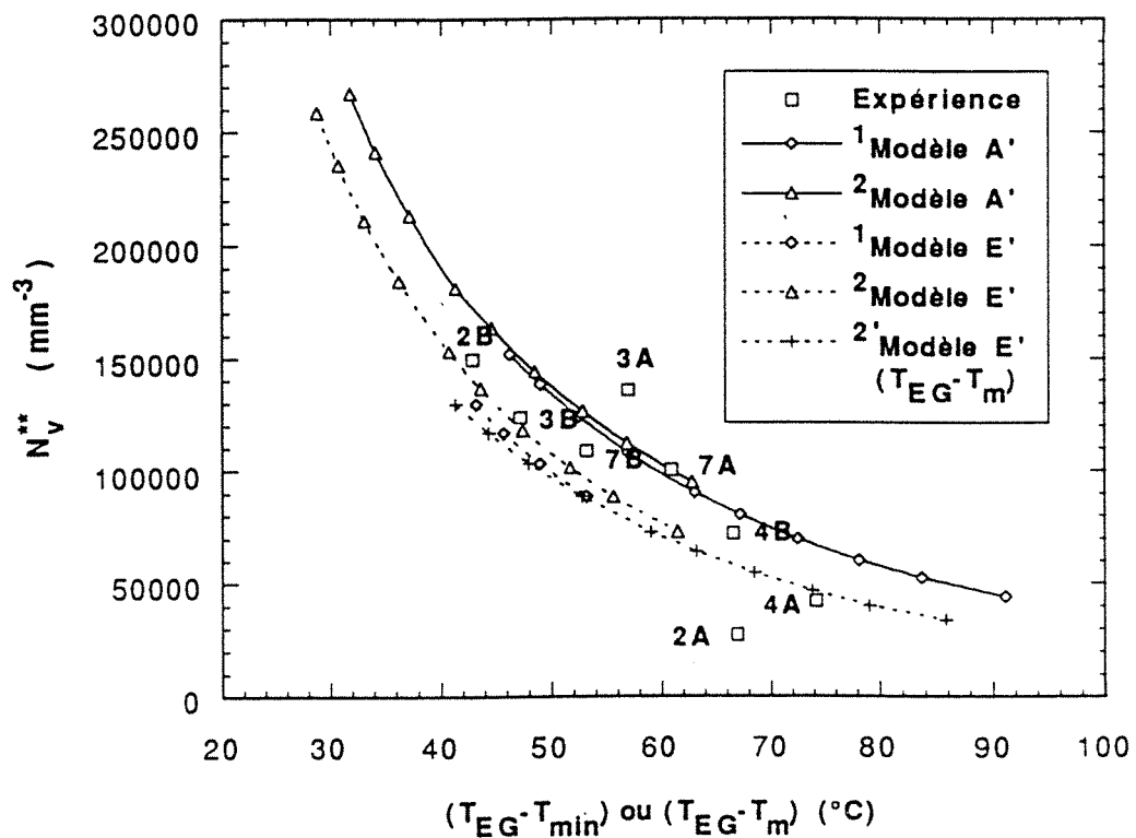
Figure 5.13 Effet du type de loi de germination sur les corrélations N_V^{**} - \Delta T_{EG} calculées pour les cylindres \varnothing 9 en faisant varier le taux d'inoculation. Les petits carrés représentent les points expérimentaux. Les courbes ont été obtenues par le calcul à l'aide des modèles A' et E'. Pour la loi de germination on a considéré n égal à 1 et à 2. Le couple de valeurs de \zeta et T_d est celui du cylindre 2B4 : \zeta = 404352 J \cdot m^{-3} \cdot ^\circ C^{-1} \cdot s^{-0,5} et T_d = 1400 ^\circ C . Les lignes en trait continu correspondent aux calculs faits avec le modèle A' et celles en pointillés résultent des calculs faits avec le modèle E'. 1 courbes qui correspondent à n égale à l'unité ; 2 courbes calculées avec n = 2 ; 2' courbe N_V^{**} - \Delta T_m calculé avec n égale à l'unité.
