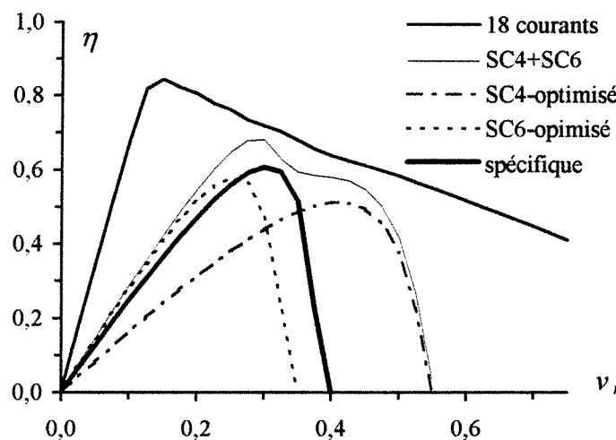
Fig. III.13 : Rendement optimal pour différents enroulements.
