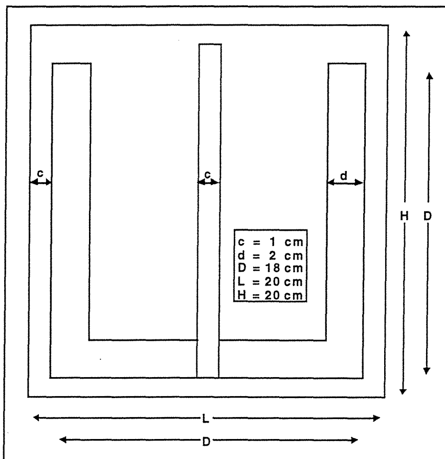
Figure 6.1 Caractéristiques géométriques du réservoir et de l'ancre.
