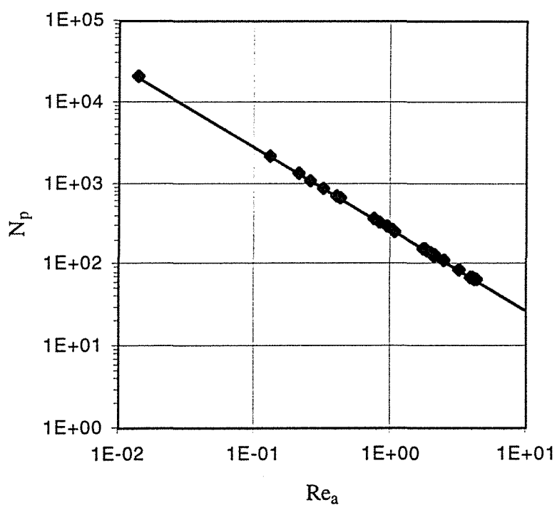
Figure 6.5 Courbe généralisée pour la puissance consommée.
