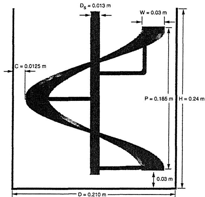
Figure 4.7 Caractéristiques géométriques du réservoir cylindrique muni d'un ruban hélicoïdal.
