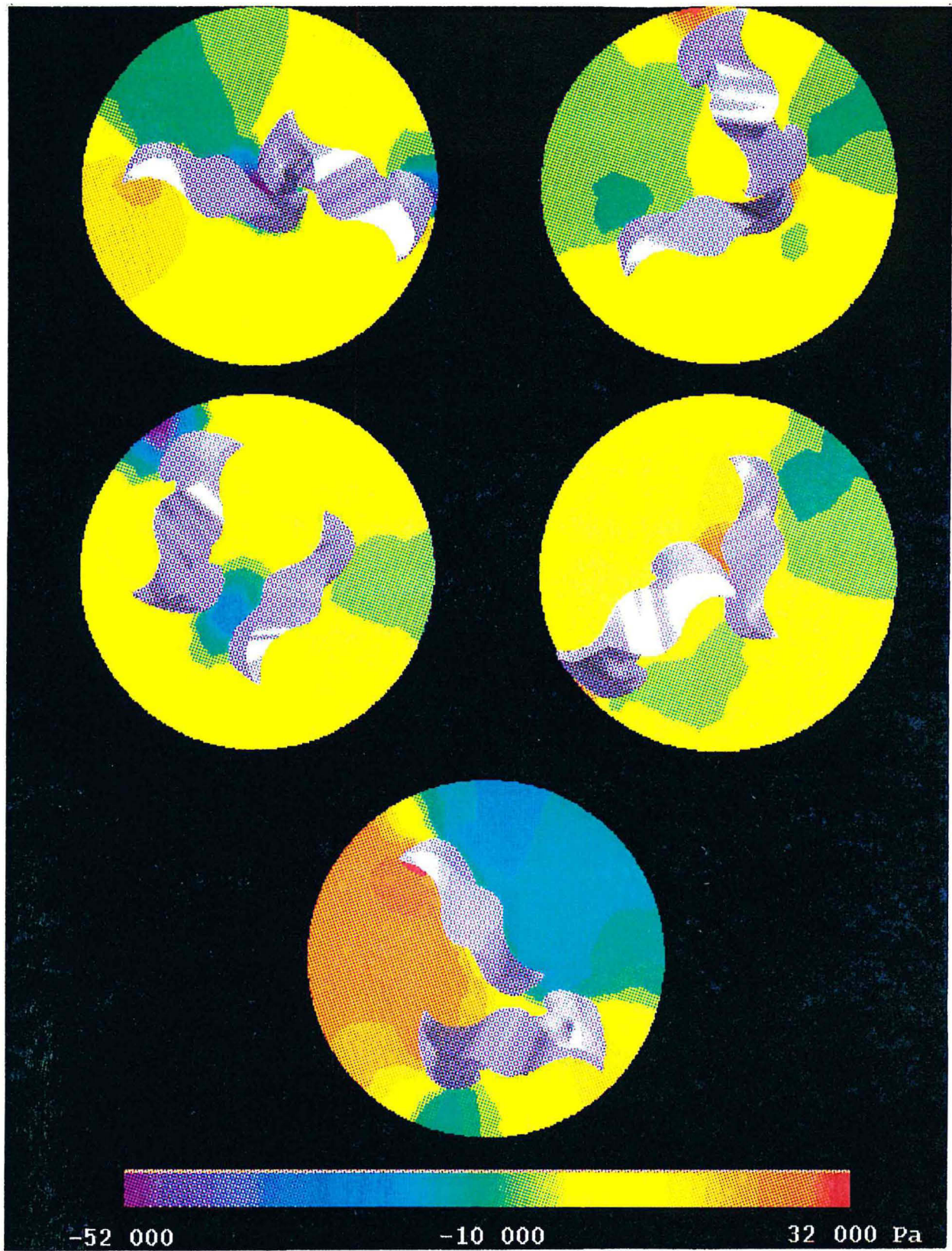
Figure 5.20 Champ de pression en régime périodique établi.
