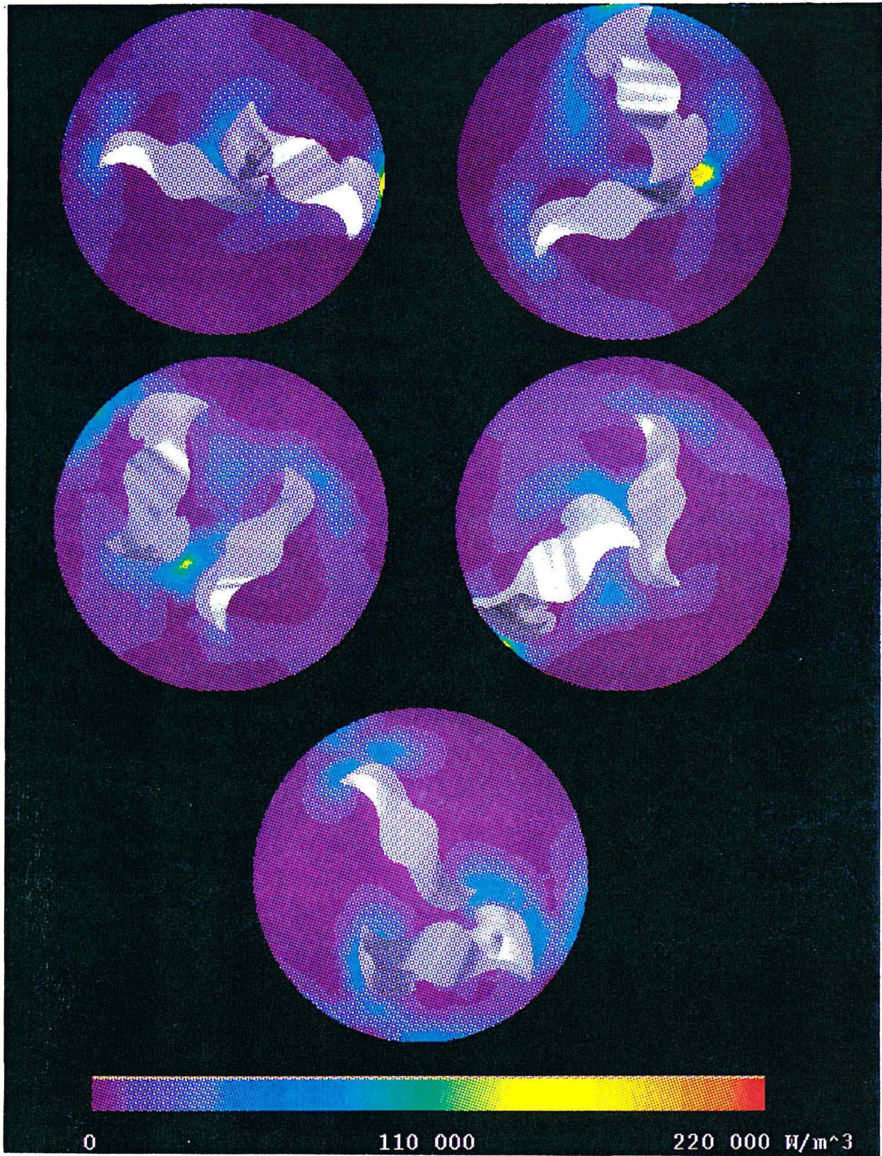
Figure 5.5 Puissance dissipée par friction en régime périodique établi.
