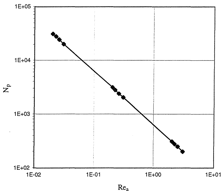
Figure 6.11 Courbe généralisée pour la puissance consommée.
