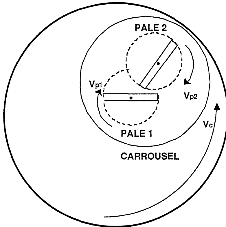
Figure 2.1 Représentation schématique d'un malaxeur à mouvement planétaire.
