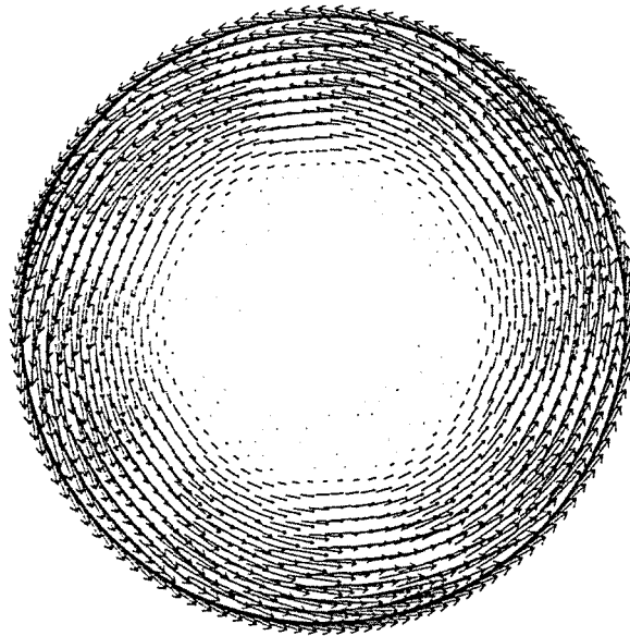
Figure 4.4 Champ de vitesse pour le problème de Couette-Hatschek ( h=0,025 ).
