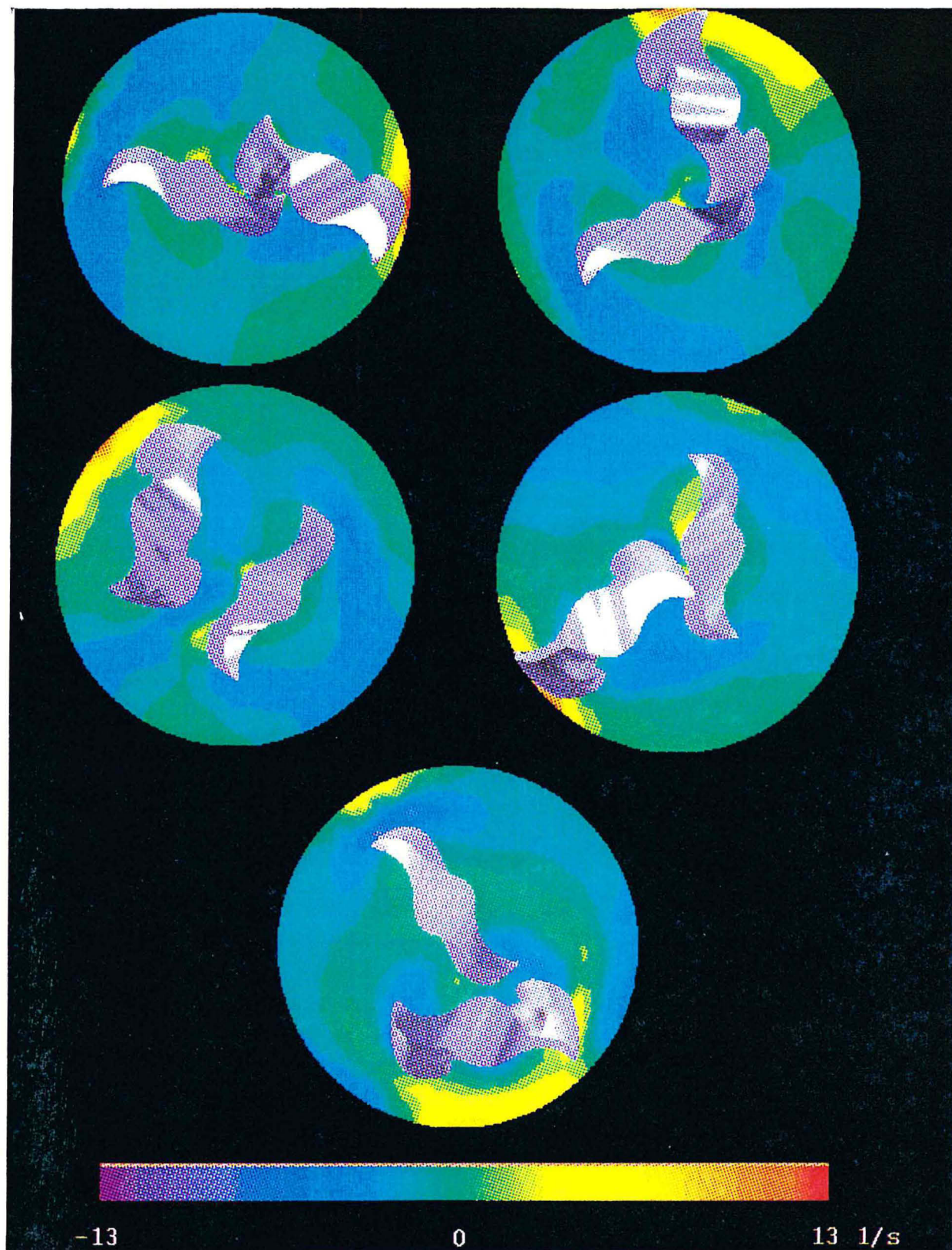
Figure 5.19 Champ de vitesse de cisaillement en régime périodique établi.
