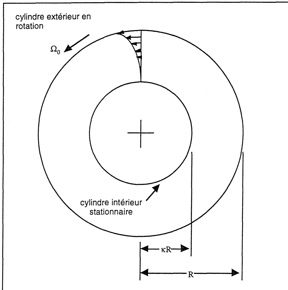
Figure 4.1 Problème de Couette-Hatschek.
