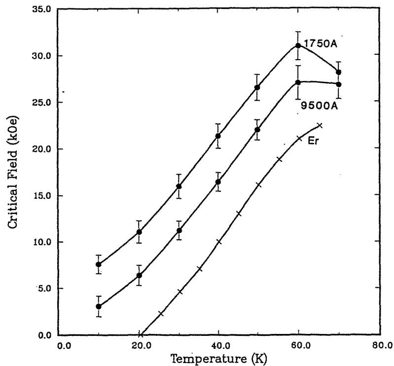
Fig. I-34 : champ critique en fonction de la température pour des films d'erbium de 1750 Å et 9500 Å épitaxiés sur yttrium, ainsi que pour l'erbium massif [58].
