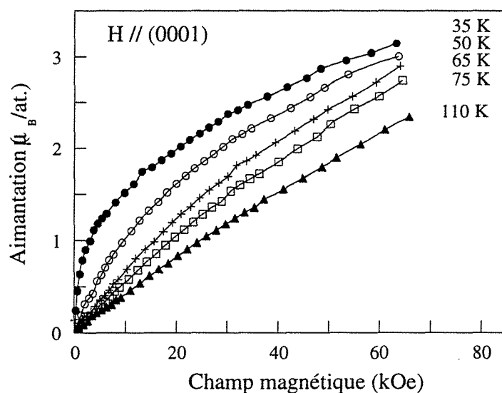
Fig. IV-41: courbes de première aimantation réalisées avec le champ magnétique appliqué perpendiculairement au plan des couches pour le superréseau [\text{Dy}(35 \text{ \AA})/\text{Er}(11 \text{ \AA})]_{\times 80} .
