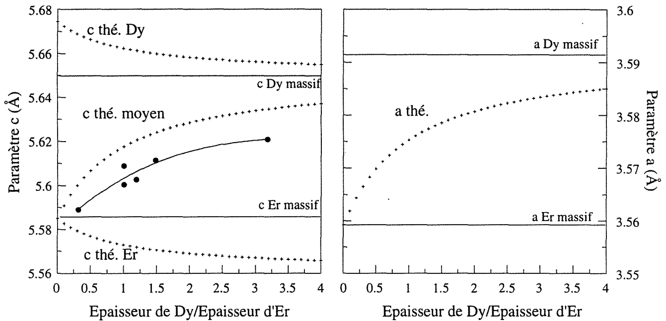
Fig. IV-2 : variation des paramètres a et c théoriques des superréseaux Dy/Er en fonction du rapport des épaisseurs des couches de dysprosium et d'erbium. Les paramètres c expérimentaux sont indiqués par les ronds noirs.
