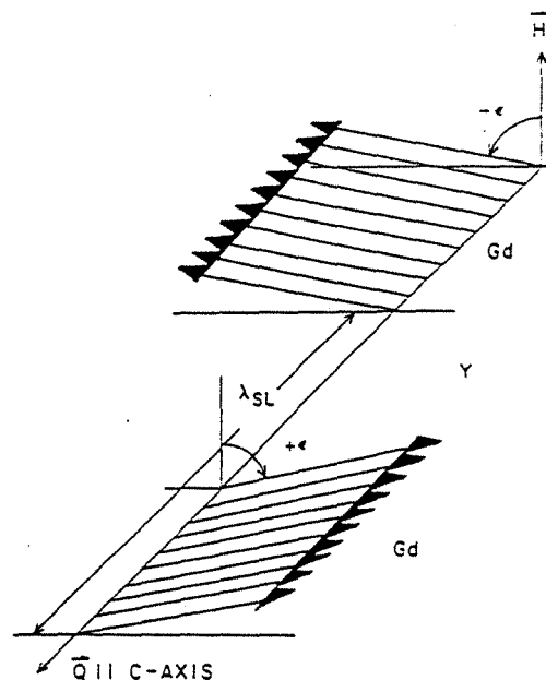
Fig. I-30 : représentation schématique de la configuration des moments magnétiques de gadolinium sous faible champ dans le superréseau [Gd_{10}Y_{10}]_{x225} [43].
