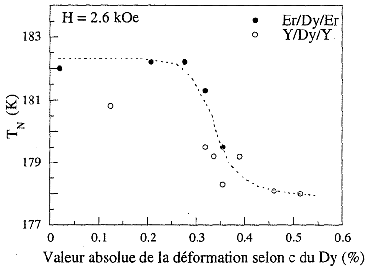
Fig. III-25 : variation de la température de Néel d'un film de dysprosium épitaxié en fonction de la valeur absolue de sa déformation selon c. Les valeurs indiquées par les symboles noirs correspondent aux films épitaxiés entre erbium ; les valeurs indiquées par les symboles blancs correspondent aux films épitaxiés entre yttrium.
