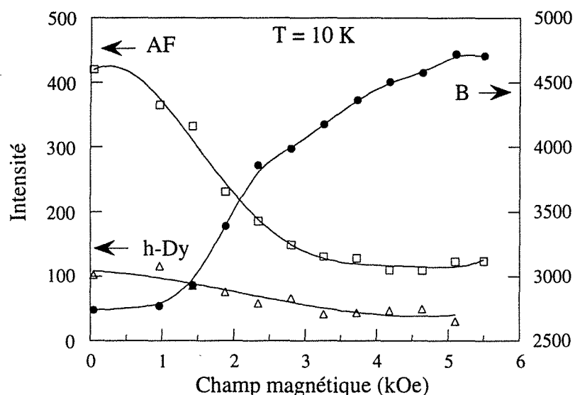
Fig. IV-15: évolutions sous champ à 10 K des intensités intégrées du pic de Bragg (B), antiferromagnétique (AF), et du pic dû à l'ordre hélicoïdal (h-Dy).
