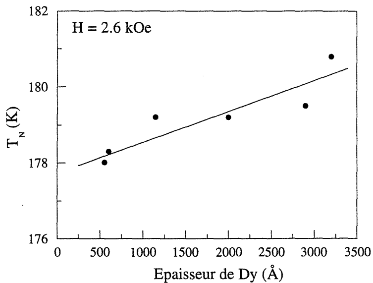
Fig. III-18: variation de la température de Néel (déterminée sous 2.6 kOe) des films de dysprosium épitaxiés entre yttrium en fonction de l'épaisseur de dysprosium.
