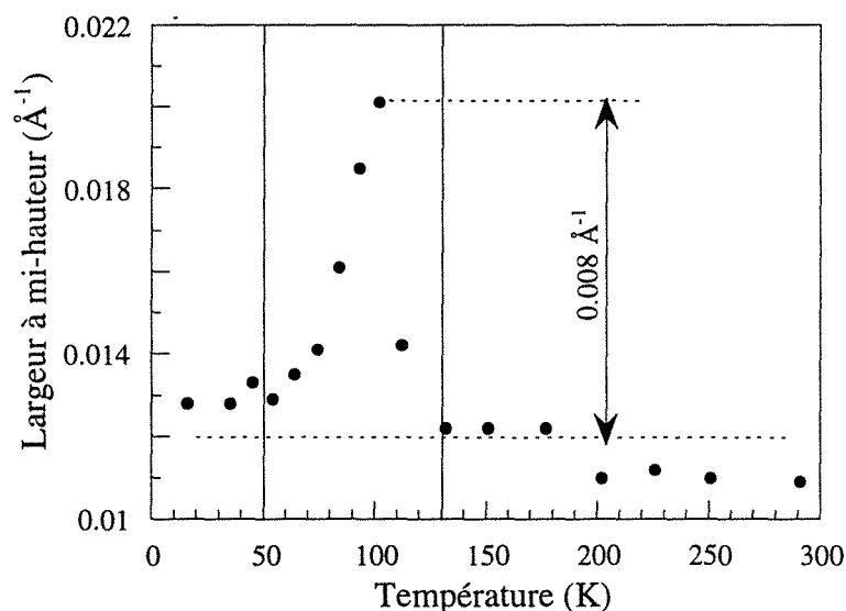
Fig. III-35 : évolution thermique de la largeur à mi-hauteur du pic de Bragg (0002) du dysprosium, mesurée par diffraction de neutrons pour l'échantillon Er/Dy 600 \text{\AA}/\text{Er} .
