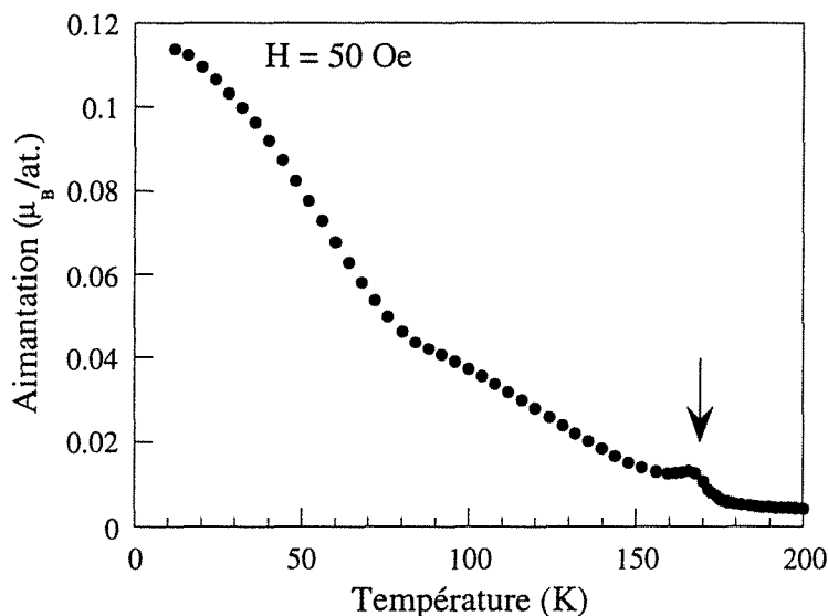
Fig. IV-7 : variation thermique de l'aimantation (FC) du superréseau [Dy(35 Å)/Er(111 Å)] x 47 sous un champ magnétique de 50 Oe. Le champ est appliqué dans le plan des couches et les mesures effectuées en température décroissante.
