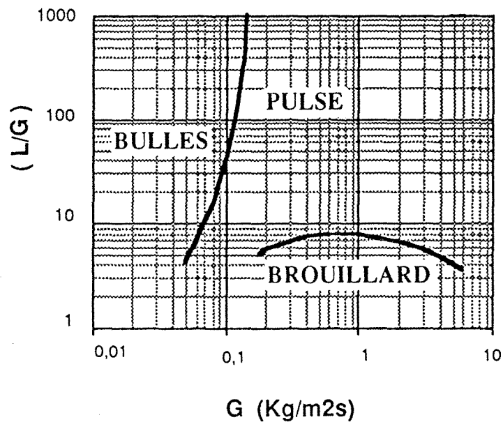
FIGURE 2.4. Diagramme des régimes d'écoulement pour le RCLFCA d'après Turpin et Huntington (1967)
