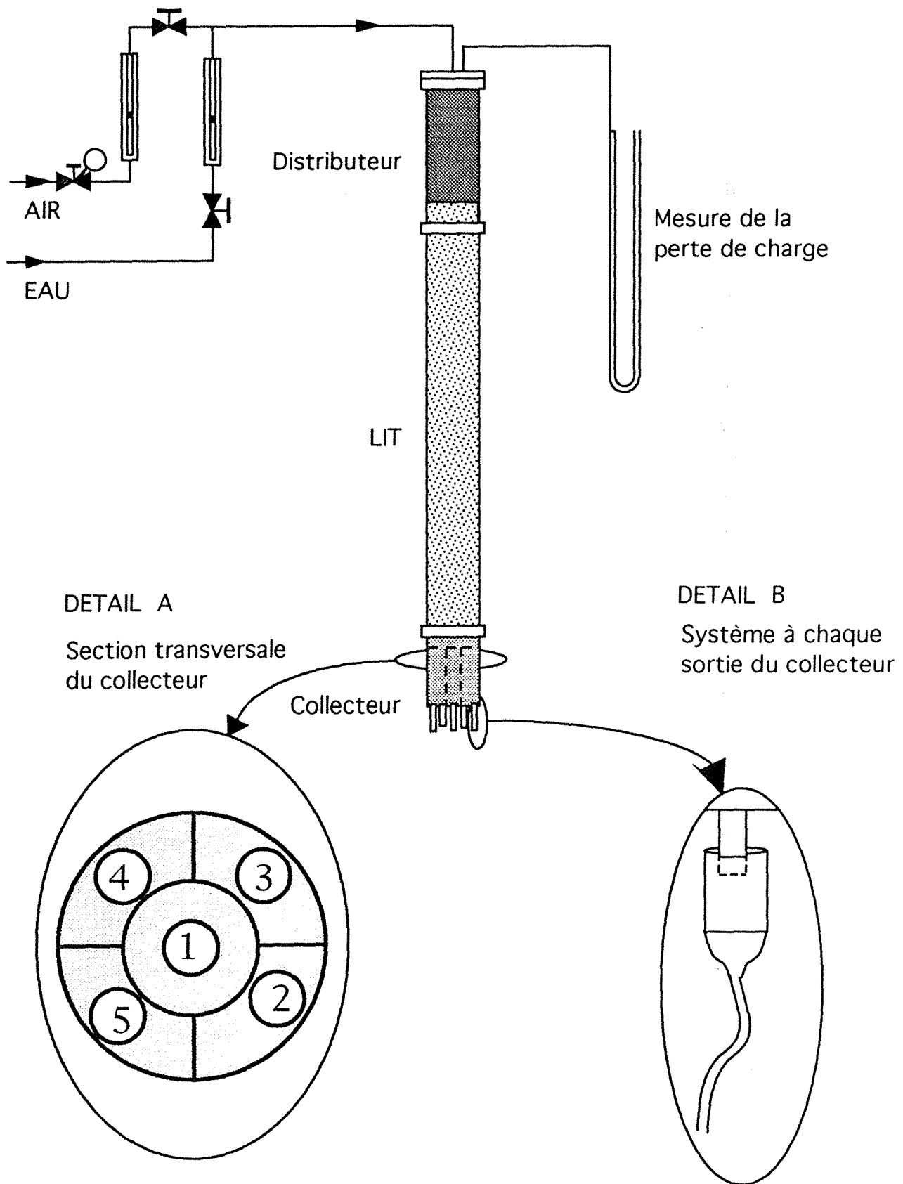
FIGURE 5.1. Schéma de l'installation utilisée pour l'étude de la distribution du liquide dans un réacteur à lit fixe avec écoulement gaz-liquide.
