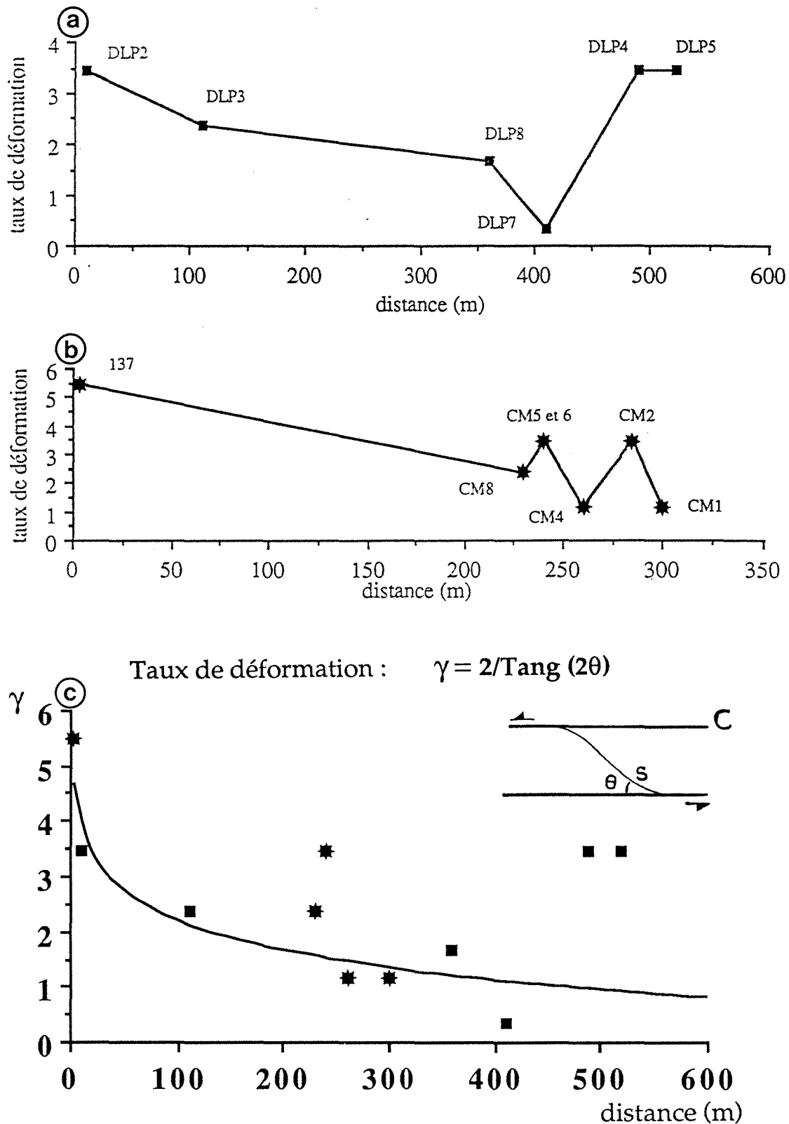
Figure III.6 : Evolution du taux de déformation ( \gamma ), déterminé par la méthode de Ramsay et Graham (1970), en fonction de la distance par rapport à la faille de la Marche. (a) Dun le Palestel (branches E-W), (b) Côte Moreau (branche N120°E), (c) synthèse de l'ensemble des échantillons des deux profils.
