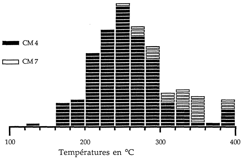
Figure V.5 : histogramme des températures d'homogénéisation des deux phases fluides pour les 2 échantillons CM 4 et CM 7.
