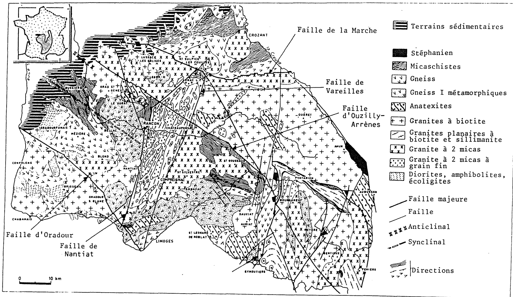
Figure I.1 : Géologie du Nord-Ouest Limousin (in Flageollet, 1977).
