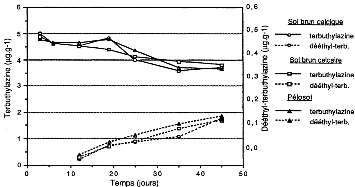
Figure 2-11 : Evolution des teneurs en terbuthylazine et son dérivé dééthyli, dans les trois sols incubés à 20°C pendant 45 jours.
