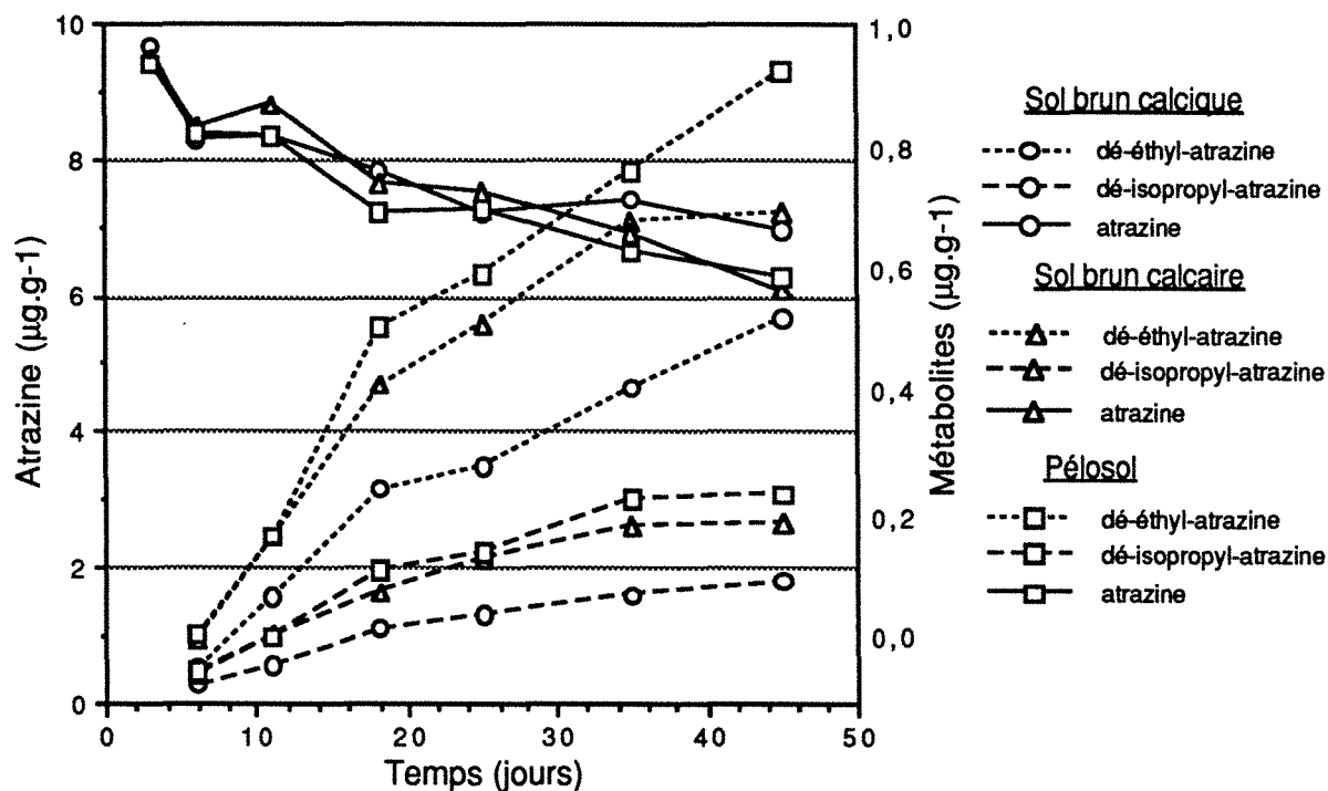
Figure 2-4 : Evolution des concentrations d'atrazine et de ses métabolites, dans les trois sols incubés à 20°C pendant 45 jours.
