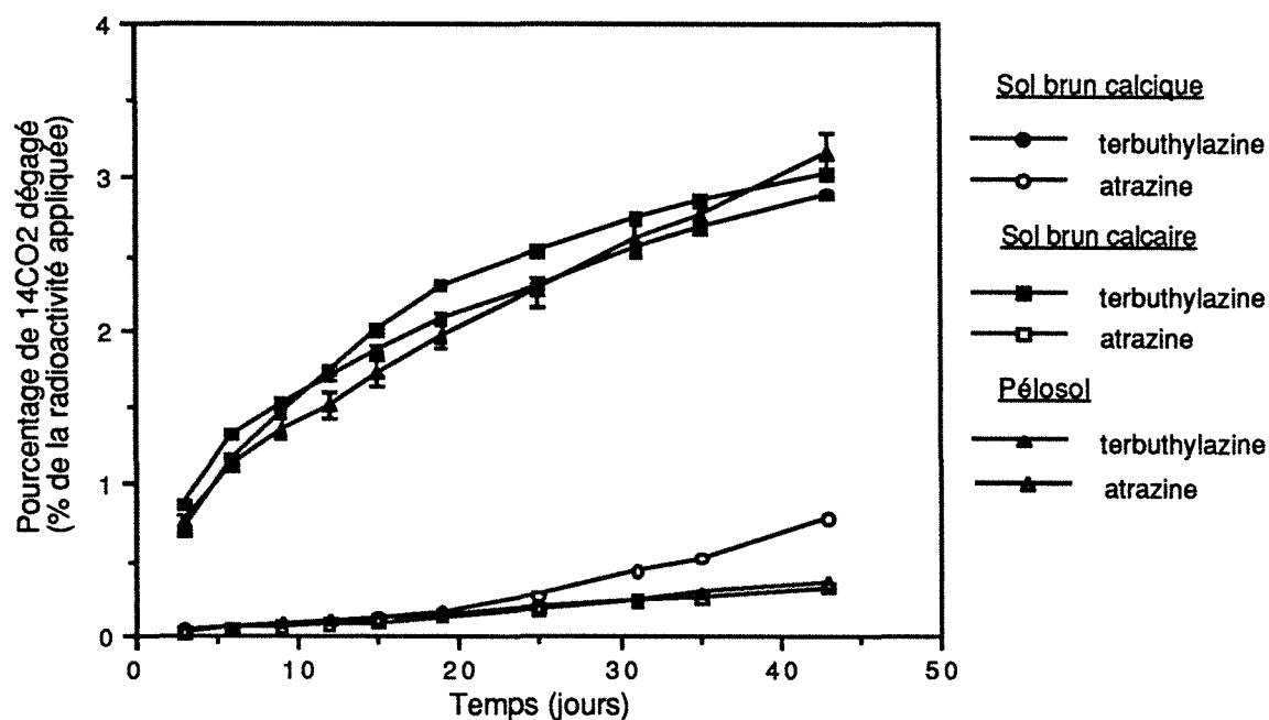
Figure 2-9 : Courbes cumulées de la minéralisation de la terbutylazine et de l'atrazine pendant 43 jours d'incubation à 20°C.
