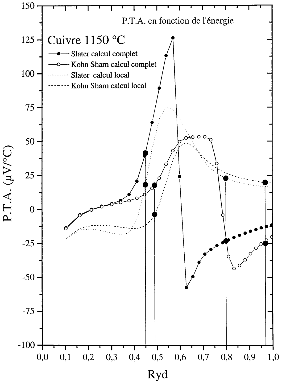
Figure III.21: P.T.A. du cuivre en fonction de l'énergie.
