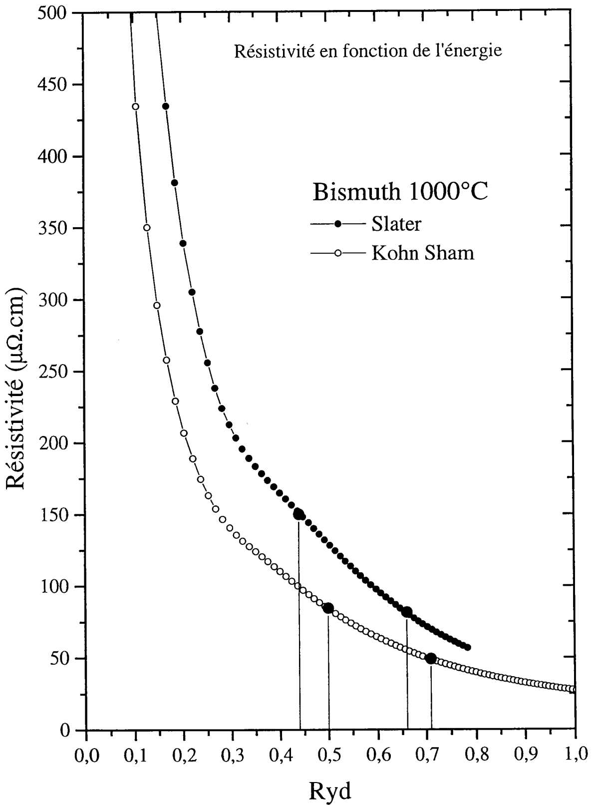
Figure III.12: Résistivité du bismuth en fonction de l'énergie.
